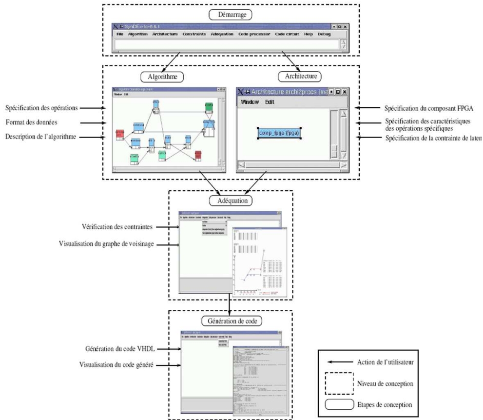
FIGURE 3.29 – Interface de l'outil SynDEx-IC
