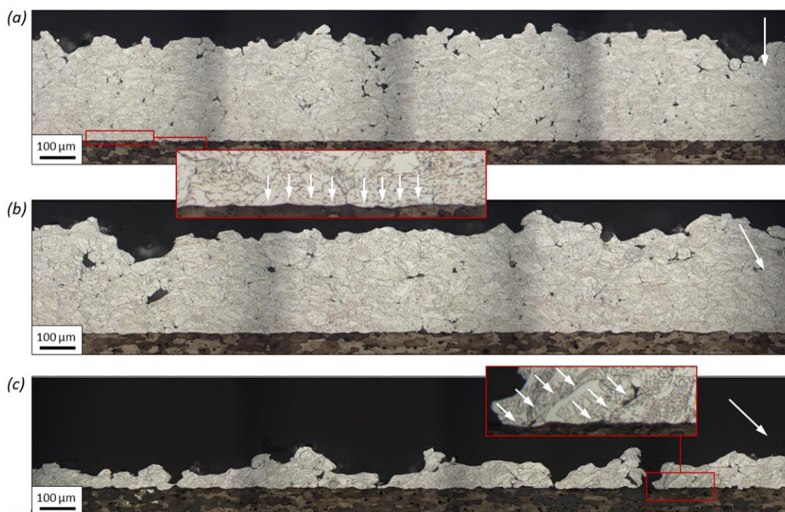
Figure 3-24 : Microscopies optiques en coupe, obtenues avec une attaque chimique « Keller » des revêtements d'aluminium pur 1050 élaborés sur substrats d'aluminium 2024-T3 avec un angle de projection de : (a) 90°, (b) 70° et (c) 50°, les flèches blanches représentent les directions de projection des particules.
