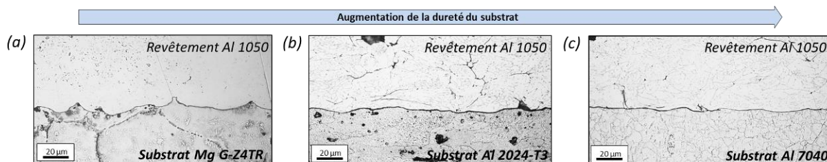
Figure 7-8 : Images optiques des interfaces des substrats bruts (a) de magnésium G-Z4TR, (b) d'aluminium 2024-T3 et (c) d'aluminium 7040 revêtus par de l'aluminium pur 1050, obtenues après une attaque chimique « Keller », montrant l'influence de la dureté du substrat sur la pénétration des particules.
