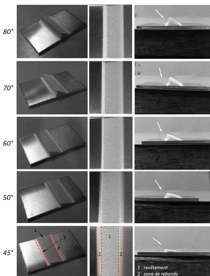
Figure B-4 : Photographies des cordons de projection de forte épaisseur observés respectivement en perspective (à gauche), en vue de dessus (au milieu) et en vue de profil (à droite) pour différents angles de projection, les flèches blanches représentent la direction de vitesse des particules projetées.
