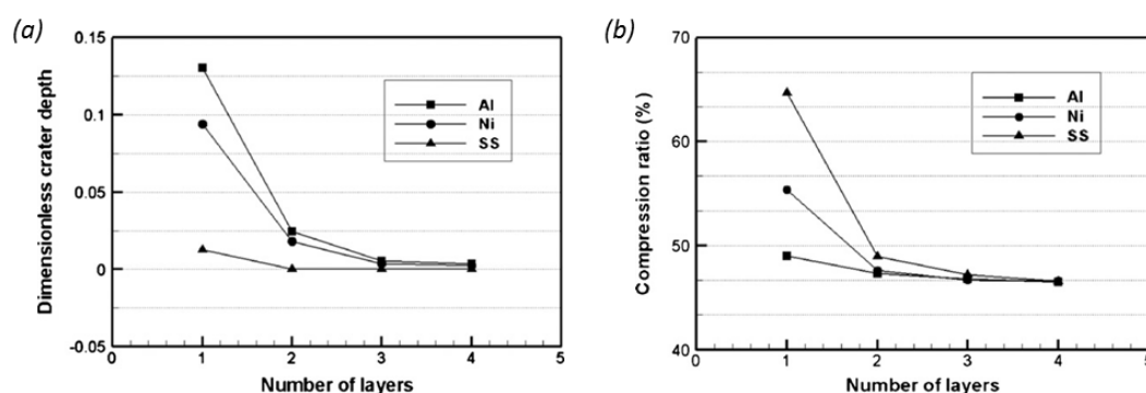
Figure 1-14 : Evolution (a) de la profondeur du cratère du substrat en fonction du nombre de couches déposées et de la nature du substrat et (b) du taux de compression de la particule [YIN11-1].
