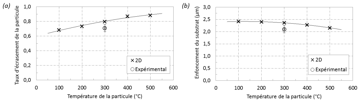
Figure 5-9 : Evolution (a) du taux d'écrasement de la particule d'aluminium pur 1050 et (b) de l'enfoncement du substrat d'aluminium 2024-T3 en fonction de la température d'impact de la particule pour des simulations 2D et comparée à l'expérimental.
