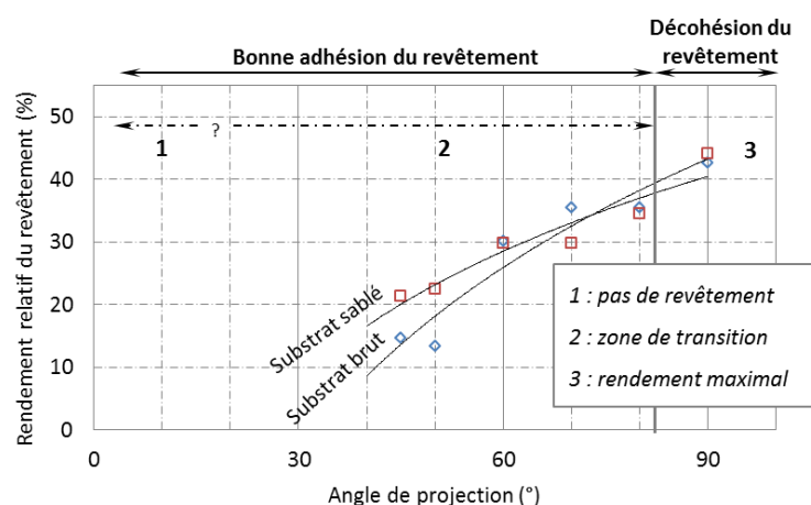
Figure B-5: Evolution du rendement de projection en fonction des angles de projection.
