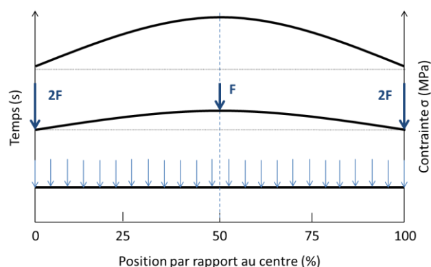
Figure A-14 : Evolution de la contrainte résiduelle au cours du temps en fonction de la position par rapport au centre de l'échantillon sablé.
