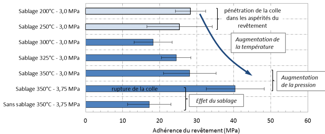
Figure 7-10 : R sultats d'adh rence d termin s par traction plots coll s des rev tements d'aluminium 2024 d pos s sur substrats d'aluminium 2024-T4 en fonction de la temp rature de gaz, de la pression de gaz et du pr -sablage du substrat.
