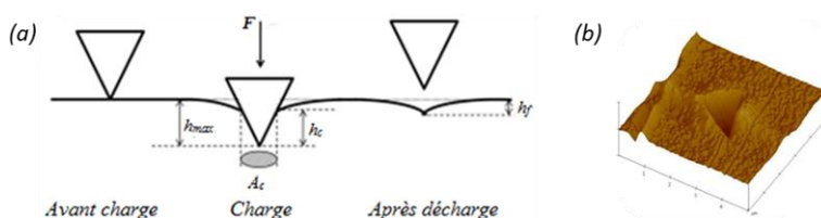
Figure 2-32 : (a) Schéma de principe de la nano-indentation (b) image AFM 3D d'une empreinte.
