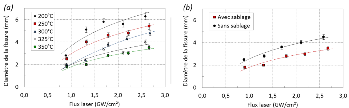
Figure 7-11 : R sultats d'adh rence d termin s par choc laser sur des rev tements d'aluminium 2024 d pos s sur substrats d'aluminium 2024-T4 en fonction (a) de la temp rature de gaz, pression fix e   3 MPa avec un sablage du substrat et (b) du sablage du substrat, temp rature de gaz fix e   350 C et pression de gaz de 3,75 MPa.
