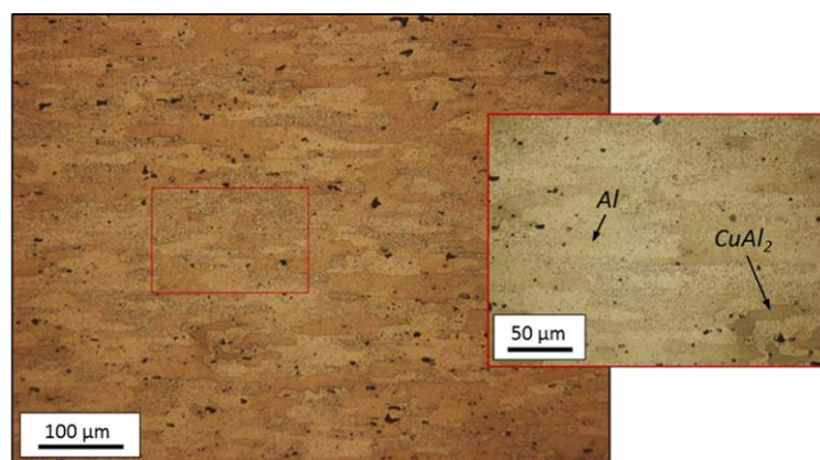
Figure A-8 : Images optiques en coupe de la microstructure de l'aluminium 2024-T3 observée après attaque chimique « Keller ».
