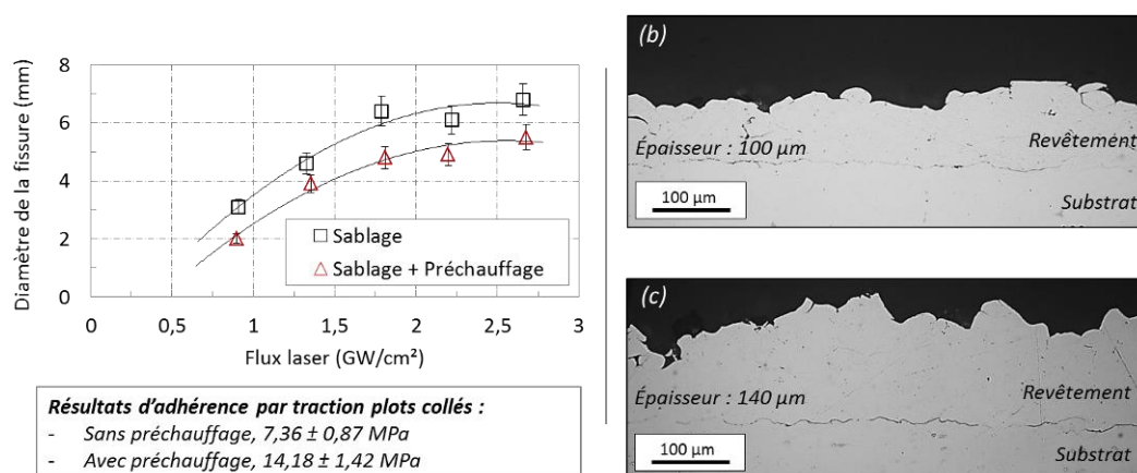
Figure 6-15 : (a) Mesures d'adhérence par choc laser (Centre des Matériaux) et plots collés (IRTES-LERMPS) des substrats d'aluminium 2024-T3 sablés (b) sans préchauffage et (c) avec préchauffage, revêtus par de l'aluminium pur 1050 et observés optiquement en coupe.
