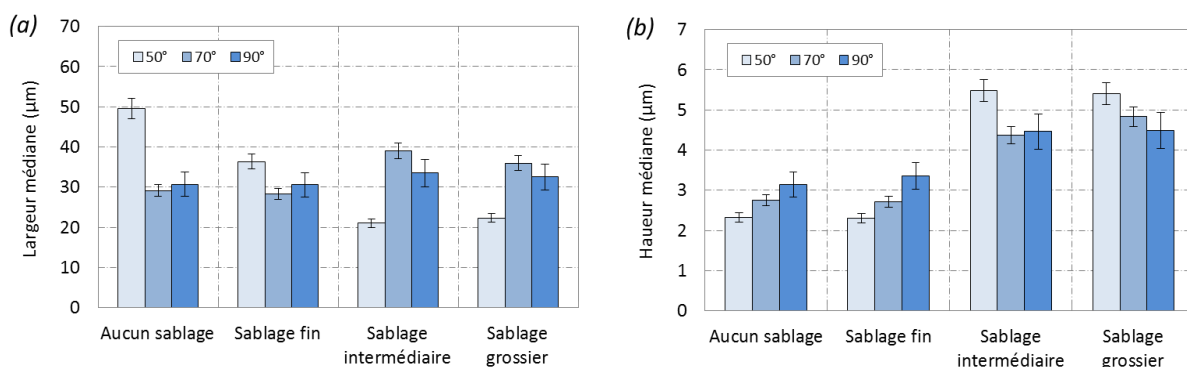
Figure 4-35 : Valeurs médianes (a) des largeurs et (b) des hauteurs des vallées des profils de l'interface aluminium pur/aluminium 2024-T3 sablés et bruts pour différents angles d'incidence de particules formant le revêtement.
