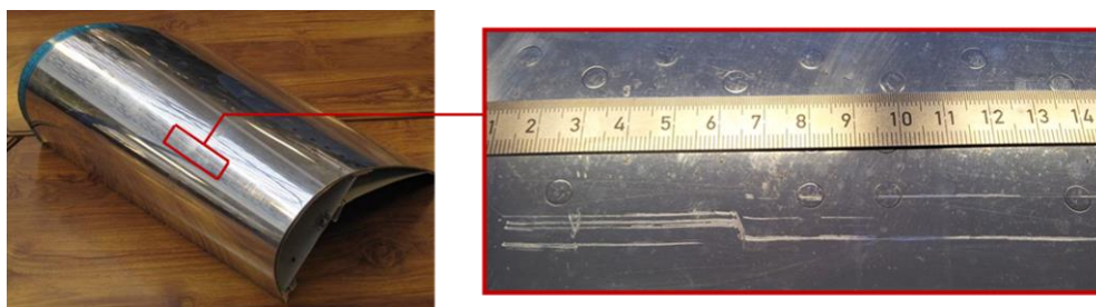
Figure 7-38 : Traces d'usure par impact en vol et au cours de la maintenance sur un bord d'attaque en aluminium 2024-T3 plaqué par de l'aluminium pur 1050, d'épaisseur 80-100 \mu\text{m} [CSA12].
