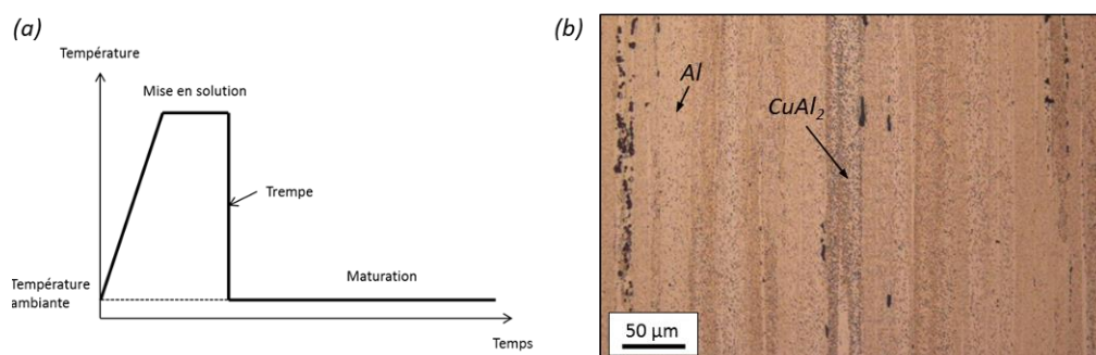
Figure A-9 : (a) Traitement thermique de type T4 et (b) image optique en coupe, obtenue après attaque chimique « Keller » de la microstructure de l'aluminium 2024-T4.
