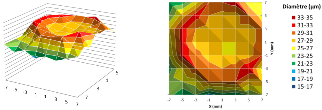
Figure 3-36 : Vue 3D et vue de dessus de la cartographie de la taille de particules d'aluminium pur 1050 grossières et sphériques (30 µm) dans un jet cold spray.
