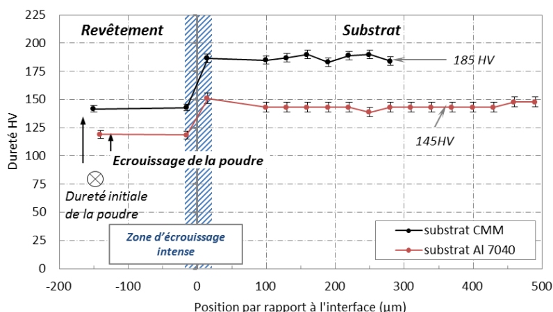
Figure 7-20 : Profils de dureté du système revêtement-substrat, depuis la surface des revêtements composites d'Al-SiC jusqu'à dans les substrats bruts d'aluminium 7040 et de CMM.
