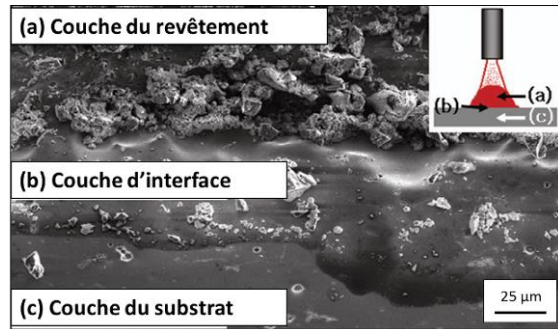
Figure 7-27 : Micrographie en coupe du moule réparé : (a) revêtement (b) interface revêtement-substrat et (c) substrat [LEE07].
