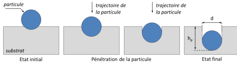
Figure 7-12 : Evolution temporelle de la pénétration d'une particule dure de SiC dans un substrat relativement plus mou, en aluminium.
