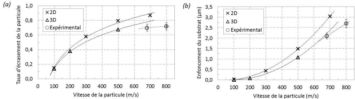
Figure 5-11 : Evolution (a) du taux d'écrasement de la particule d'aluminium pur 1050 et (b) de l'enfoncement du substrat d'aluminium 2024-T3 en fonction de la vitesse d'impact de la particule pour des simulations 2D et 3D et comparée à l'expérimental.
