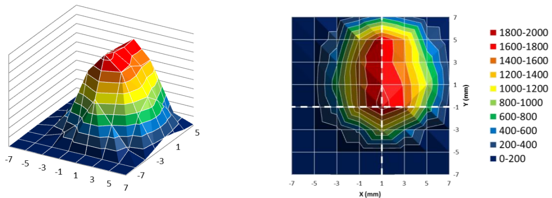
Figure 3-33 : Vue 3D et vue de dessus de la cartographie en nombre des particules d'aluminium pur 1050 grossières et sphériques (30 µm) dans un jet cold spray.
