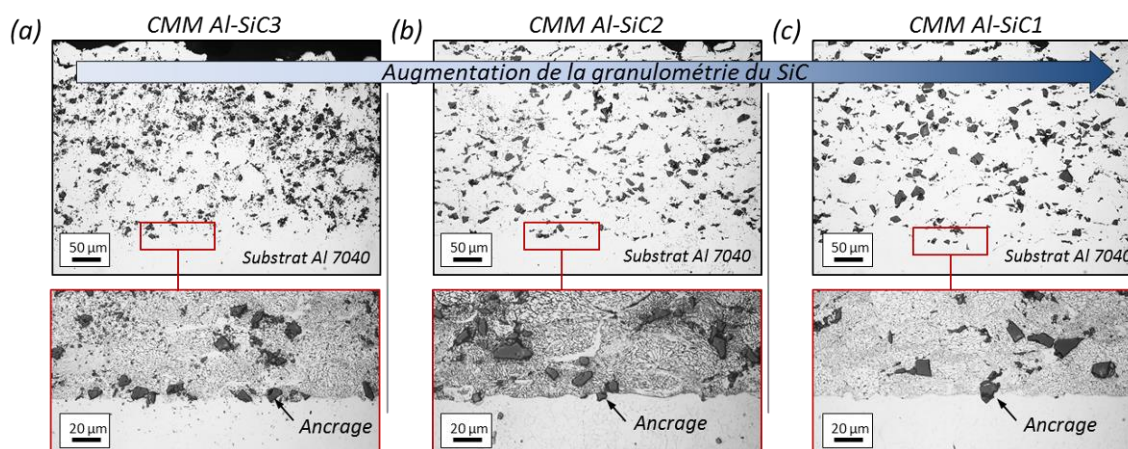
Figure 7-19 : Images optiques en coupe, sans attaque chimique (en haut) et avec attaque chimique « Keller » (en bas) des revêtements composites CMM élaborés à partir d'une poudre d'Al-SiC sur un substrat d'aluminium 7040 et dont la granulométrie des particules de SiC, d(0,5) , varie : (a) 15 \mu\text{m} , (b) 21 \mu\text{m} et (c) 26 \mu\text{m} .
