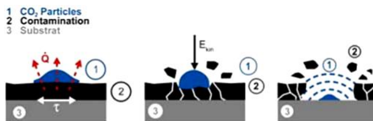
Figure 2-23 : Mécanismes d'activation de la surface du substrat par projection de carboglace [DON12-2].
