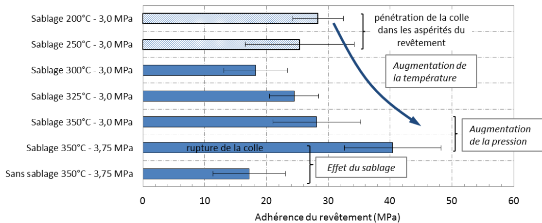
Figure 7-10 : Résultats d'adhérence déterminés par traction plots collés des revêtements d'aluminium 2024 déposés sur substrats d'aluminium 2024-T4 en fonction de la température de gaz, de la pression de gaz et du pré-sablage du substrat.
