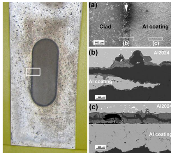
Figure 7-34 : Image de l'éprouvette réparée après une immersion pendant 480 h dans un bain corrosif, en vue de dessus (a gauche), (a) présence de corrosion par piquûre à la jonction revêtement/couche protectrice initiale, indiquée par la flèche blanche et (b et c) images MEB en coupe, en électrons secondaires, de cette jonction [YAN14].
