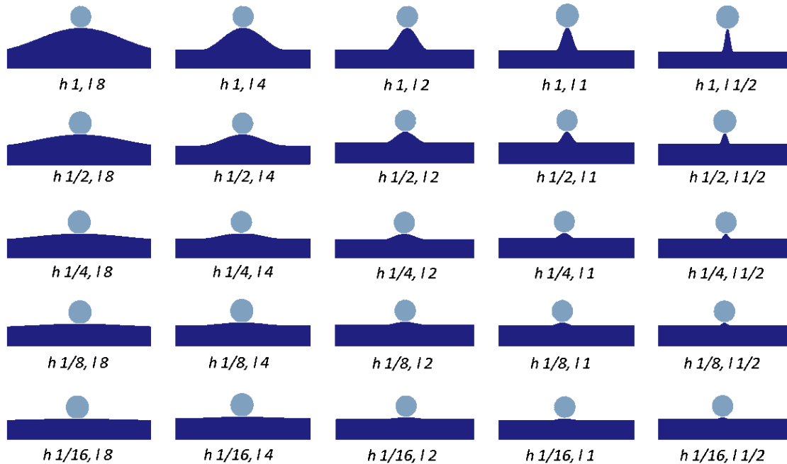
Figure 4-16 : Configurations d'impact d'une particule d'aluminium pur 1050 sur un pic défini par une largeur et une hauteur, pour un substrat d'aluminium 2024-T3.
