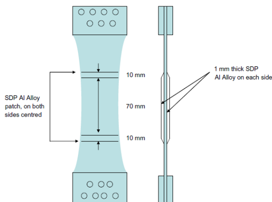
Figure 7-32 : Epreuves en aluminium 2024-T3 sollicitées en traction avec l'ajout d'un revêtement d'aluminium élaboré par cold spray [JON11].
