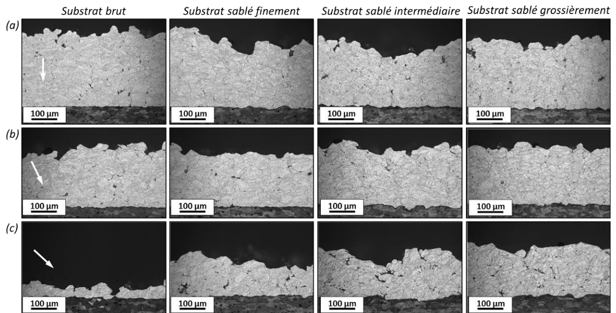
Figure 3-4 : Images optiques en coupe, obtenues après une attaque chimique « Keller », des revêtements d'aluminium pur élaborés à partir de poudre de 30 µm de diamètre moyen, sous différents angles de projection : (a) 90°, (b) 70° et (c) 50°, la direction de projection, sur substrats d'aluminium 2024-T3 brut et sablés, est représentée par les flèches blanches.
