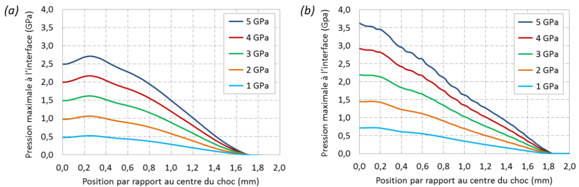
Figure 6-22 : Profils radiaux 1D des contraintes en traction le long de l'interface revêtement-substrat (a) plane et (b) rugueuse, pour des pressions maximales incidentes de choc allant de 1 à 5 GPa.
