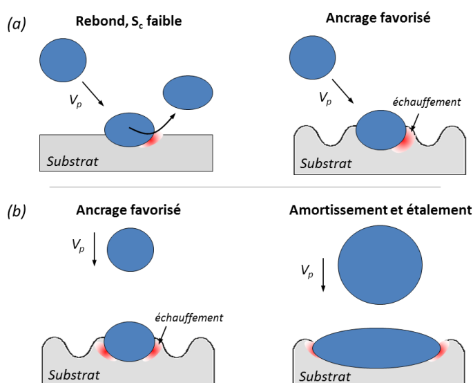
Figure 6-25 : Représentation schématique des mécanismes de déformation de la particule et du substrat en fonction (a) de l'angle d'incidence de la particule avec le substrat plan (à gauche) et rugueux (à droite) et (b) du diamètre de la particule comparativement aux dimensions des rugosités du substrat, petite particule (à gauche) et grosse particule (à droite).
