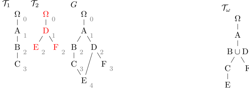
(b) Les AdFs marginaux \mathcal{T}_1, \mathcal{T}_2 et le GdF. La profondeur apparaît en gris clair près des nœuds.
