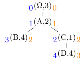
(a) Image originale u , ses formes et ses lignes (b) L'AdF de u et l'évaluation de \rho_{TV} (bleu) et de \rho_{CV} (orange).
