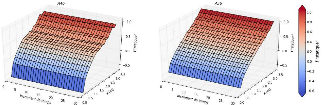
Figure 4-23 : f_{statique} pour les armatures A36 et A46
