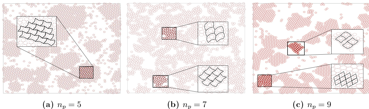
FIGURE 6.11 – Types de cristaux obtenus en fonction du nombre patches par particule n_p
