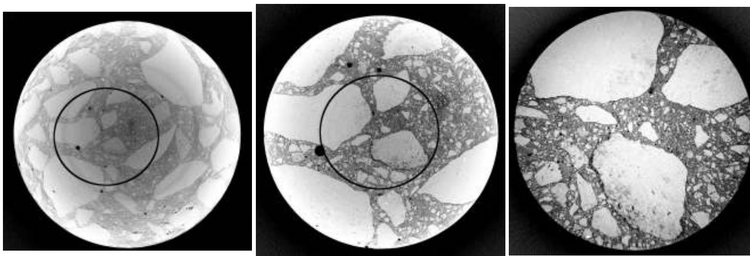
FIGURE 1.19 – Extraits de tomographies, diamètre 95mm, 50mm et 20mm. On retrouve la même zone d'une image sur l'autre. Un côté d'un granulat semble fissuré sur les deux images les mieux résolues. Ce défaut est-il la conséquence du retrait de la pâte de ciment ? Ce côté du grain semble présenter plus de défauts que les grains voisins.
