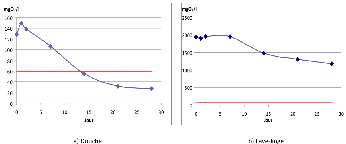
Figure 30 : Evolution de la DCO dans les eaux a) de douche et b) de lave-linge au cours du temps
