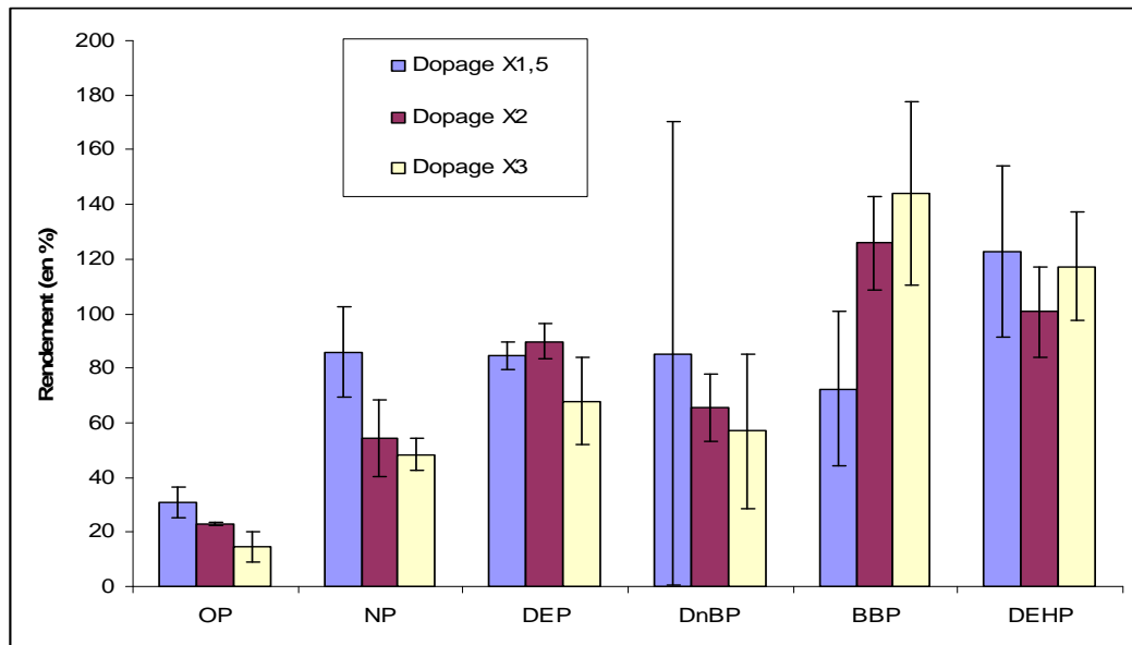
Figure 51 : Rendements d'extraction pour les alkyphénols et les phtalates (en %)
