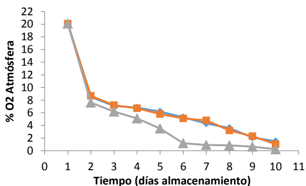
Figura 8. Desempeño de consumo de oxígeno de película activa Polipropileno/Aceite de linaza encapsulado con tamaño de partícula inferior a 25 µm (▲), entre 45 y 25 µm (■) y entre 105 y 45 µm (♦) , activación 90% humedad 1 h, espesor 58 µm.
