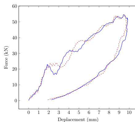
(d) Force/Déplacement
