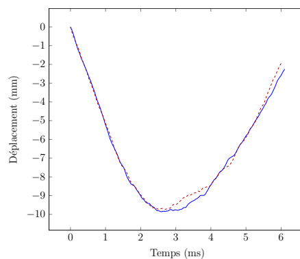
(b) Déplacement/temps
