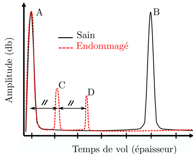
FIGURE 3.10: Représentation d'un signal A-scan pour un matériau sain et pour un matériau endommagé
