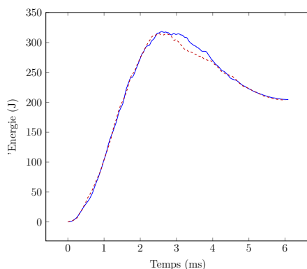
(g) Énergie/temps
