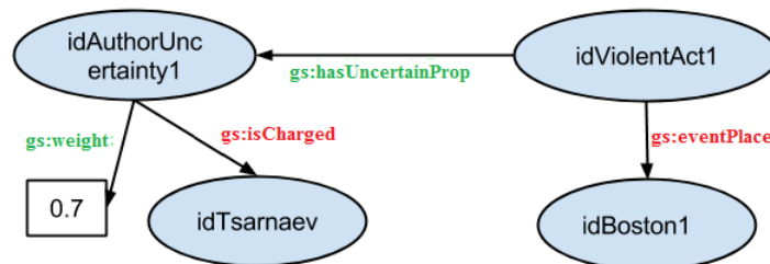
FIGURE 3.8 – Graphe RDF de l'exemple 18 relatif au patron 2.
