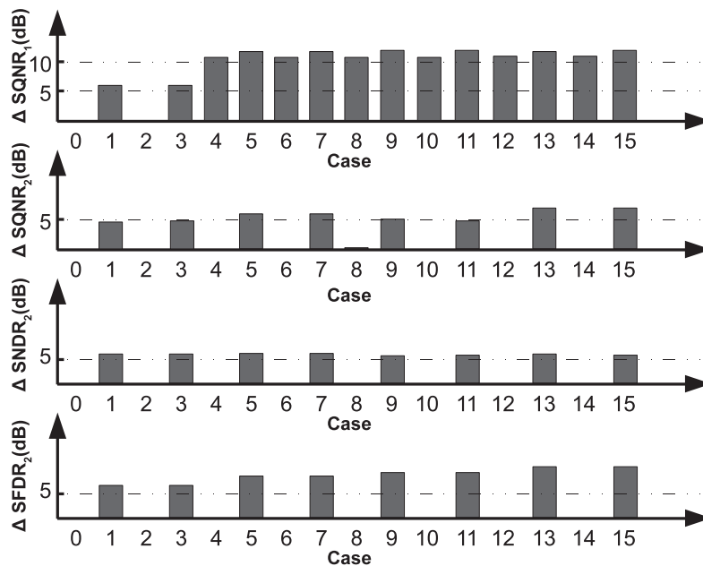
Figure 19: La dégradation de la performance versus le cas faillant du blocque par la barre graphique, SQNR 1 (cas minimum du design) et SQNR 2 , SNDR 2 , SFDR 2 (cas de sur-design). \Delta = X_0 - X_i est la paramètre de la performance, 'i' est l'index des cas.
