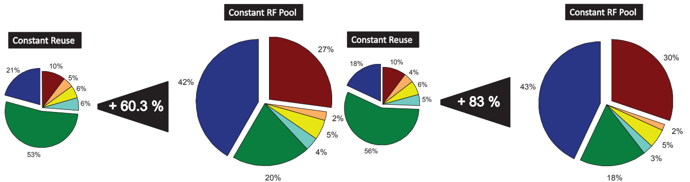
(d) Four RFs per cell.
