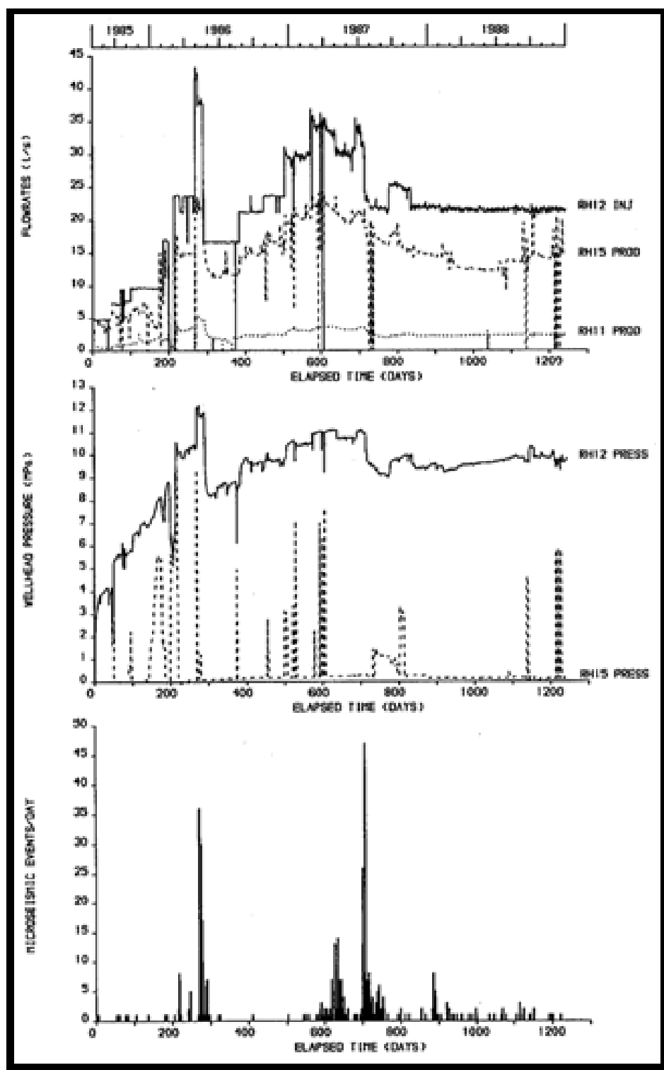
Figure 3.3 : Pression, débit, nombre des événements micro-séismiques par jour, du 7 août 1985 au 31 décembre 1988 (Baria et Green, 1989)
