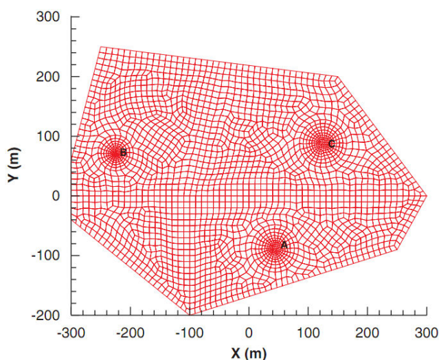
Figure 2.23 : Discretisation d'une fracture d'extension finie et de forme arbitraire plane, où A est le puits d'injection de fluide, et B et C sont des puits des productions (Zhou et al., 2009).
