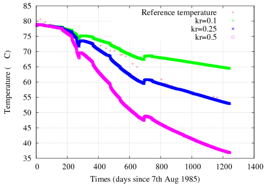
Figure 3.37 : Température de production pour différentes valeurs du coefficient kr et données de terrain (rouge)
