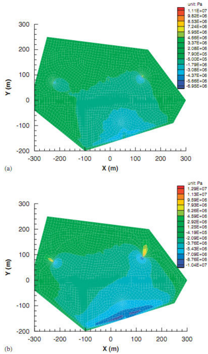
Figure 2.25 : Distributions de la contrainte \sigma_{zz} (Pa) à la surface de la fracture lorsque les temps d'injection de fluides sont de 6 mois (haut) et 3 ans (bas) (Zhou et al., 2009)
