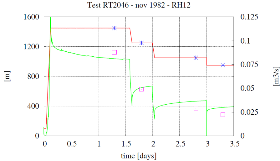
Figure 3.28 : Scénario de simulation du test de stimulation hydraulique RT2046. Les surpressions exprimées en m sont prescrites constantes par palier et linéaires entre paliers (courbe continue rouge). Les couples de points avec les figurés « étoile » et « carré » sont les mesures en fin de palier que l'on peut relever sur la Figure 3.24. La courbe verte est le débit d'injection simulé par FRACAS sur le modèle calibré.
