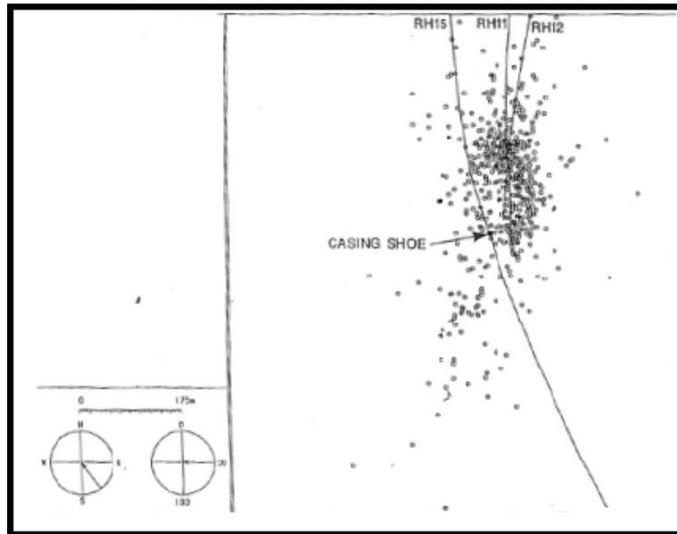
Figure 3.26 : Localisation des micro-séismes induits pendant les premières 38 h du test RT2A046 (vue dans la direction Nord 150), d'après Parker (1989)
