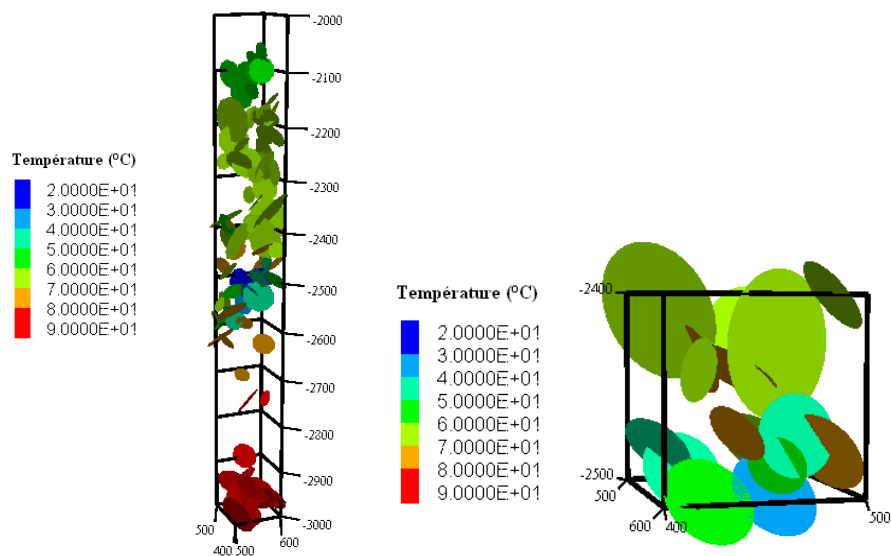
Figure 2.21 : (à gauche) Température du fluide dans une « colonne » verticale au centre du bloc, entre les abscisses x=400 et x=500 , et les ordonnées y=500 et y=600 , extraites du réseau 3D. (à droite) Unité du modèle continu à grande échelle de 100 m de côté, située à l'intersection de la tranche horizontale de la Figure 2.19 et de la colonne de la Figure 2.20. Les disques présentés ont tous leur centre situé dans cette unité et sont utilisés pour le calcul du terme source discrétisé (2:17) dans l'équation (2:20).
