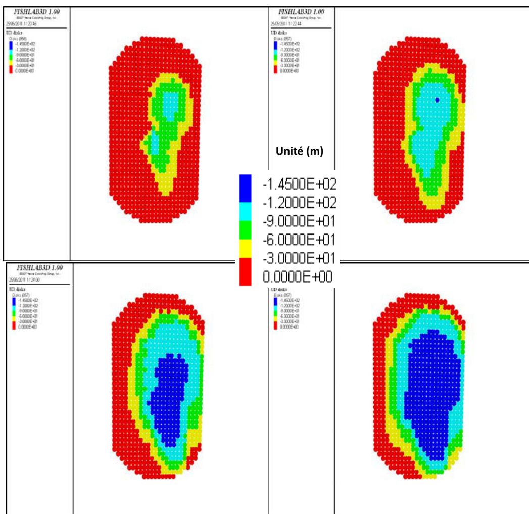
Figure 3.22 : Evolution de la contrainte thermique, au cours des 3 années de test de circulation divisées en 4 périodes de durée de 300 jours, sur la fracture d'injection C1 (N135) en partant du gauche vers la droite et du haut vers le bas. Le maximum de contrainte de traction induite est de l'ordre de 1.5 MPa, sur plus de 150 m de hauteur dans le réservoir.
