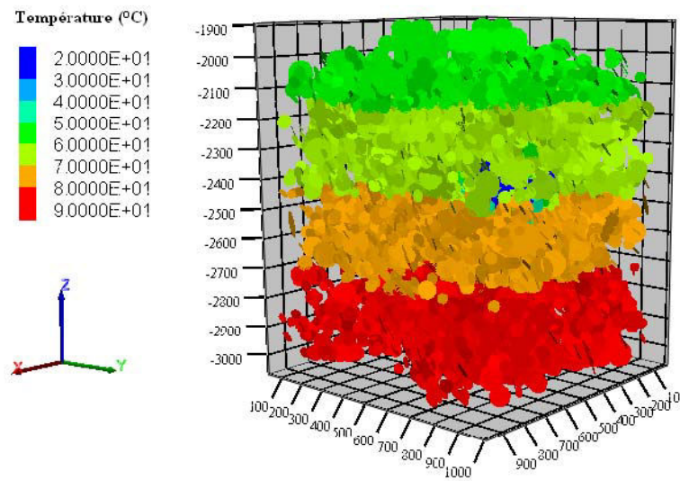
Figure 2.18 : Image du bloc réservoir fracturé à la date t = 10 ans après le début de l'injection. La couleur indique la température au centre de chaque élément « disque » du réseau simulé.
