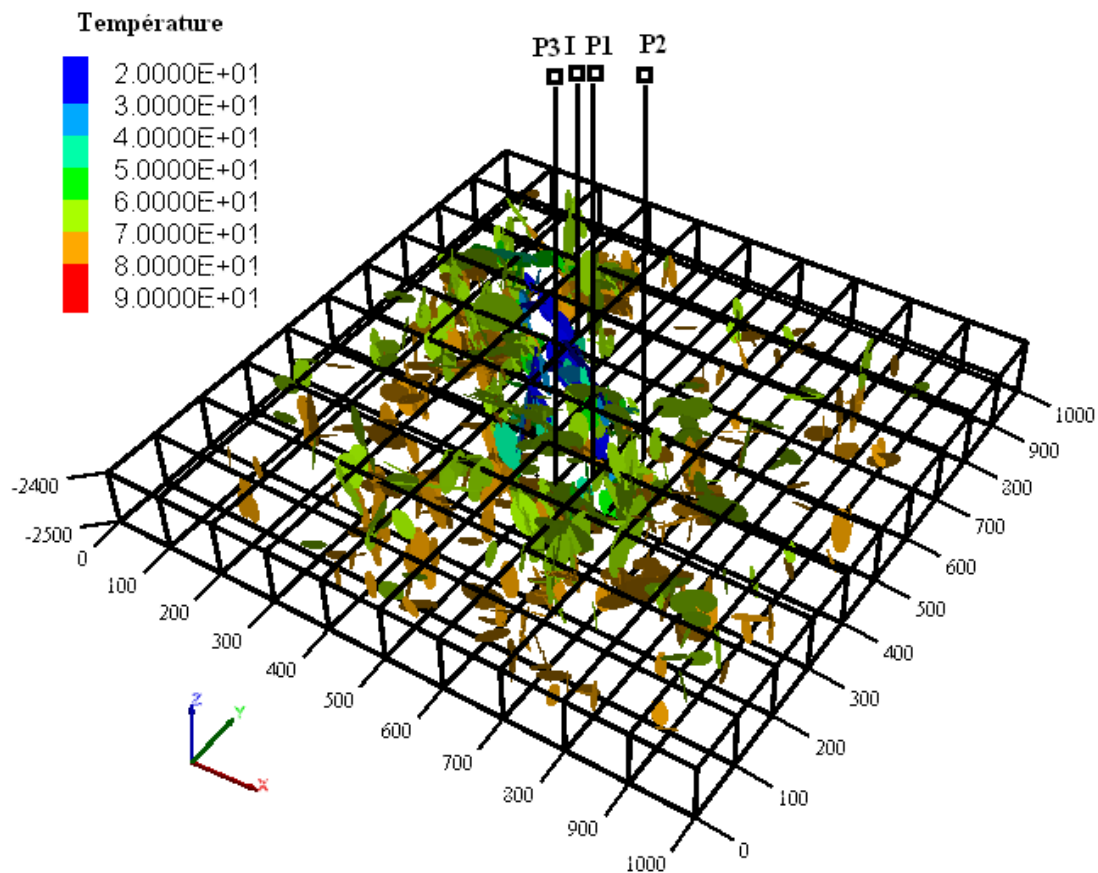
Figure 2.19 : Température du fluide \theta_f calculée dans les disques du réseau situés entre les profondeurs 2400 et 2500 à la date 10 ans. Les points I, P1, P2, P3 marquent la position des puits verticaux. Dans cette coupe horizontale la distance entre le puits I et P est de l'ordre de 350 m.
