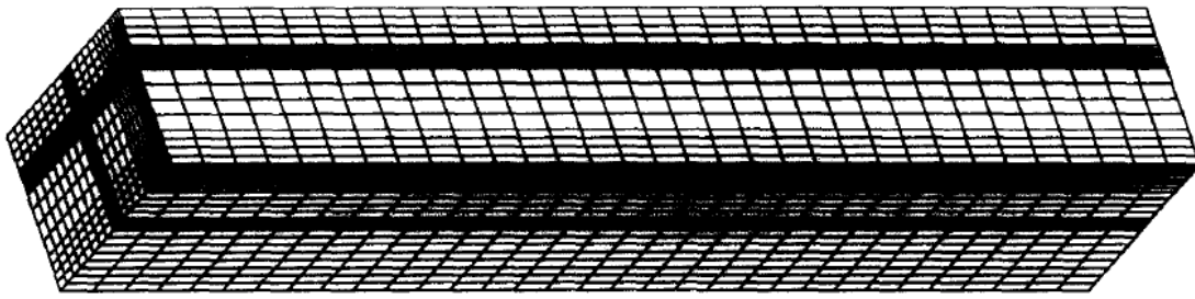
Figure 3.10 : Maillage d'élément fini utilisée pour la simulation numérique (Kolditz et Clauser, 1998)
