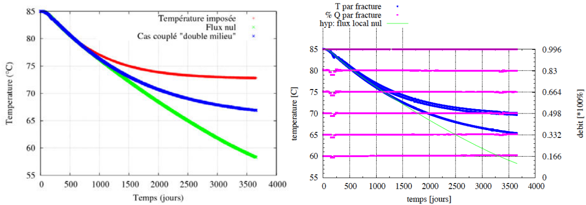
Figure 2.16: (a) Température de production simulée (bleu) par le modèle double milieu-discret, comparée aux valeurs obtenues avec les anciennes hypothèses de traitement du milieu continu adjacent aux fractures (hypothèse d'une valeur imposée fixée ou d'un flux nul aux limites des blocs locaux attachés aux disques du modèle d'écoulement). (b) Evolution des débits cumulés montrant la stabilité de la répartition par fracture et évolution des températures par fracture, montrant le refroidissement plus marqué des fractures « internes ».
