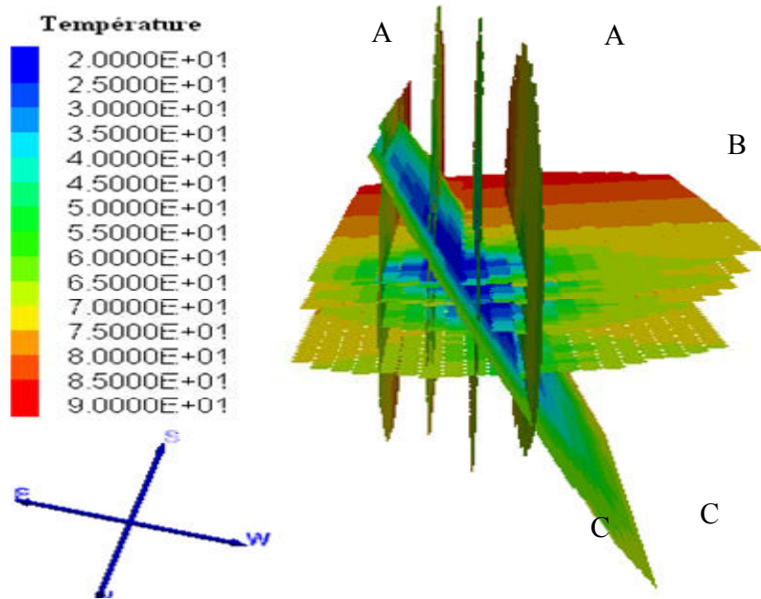
Figure 3.19 : Température de production du modèle 3D au cours de 3 années de test de circulation, les fractures B sont orientées du Sud vers le Nord et les fractures A de l'Est vers l'Ouest
