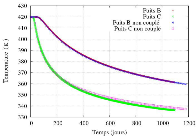
Figure 2.29 : Comparaison des températures de production dans le cas où il y a un couplage entre perméabilité et contrainte normale effective et dans le cas où le couplage est omis pour 3 années d'injection.
