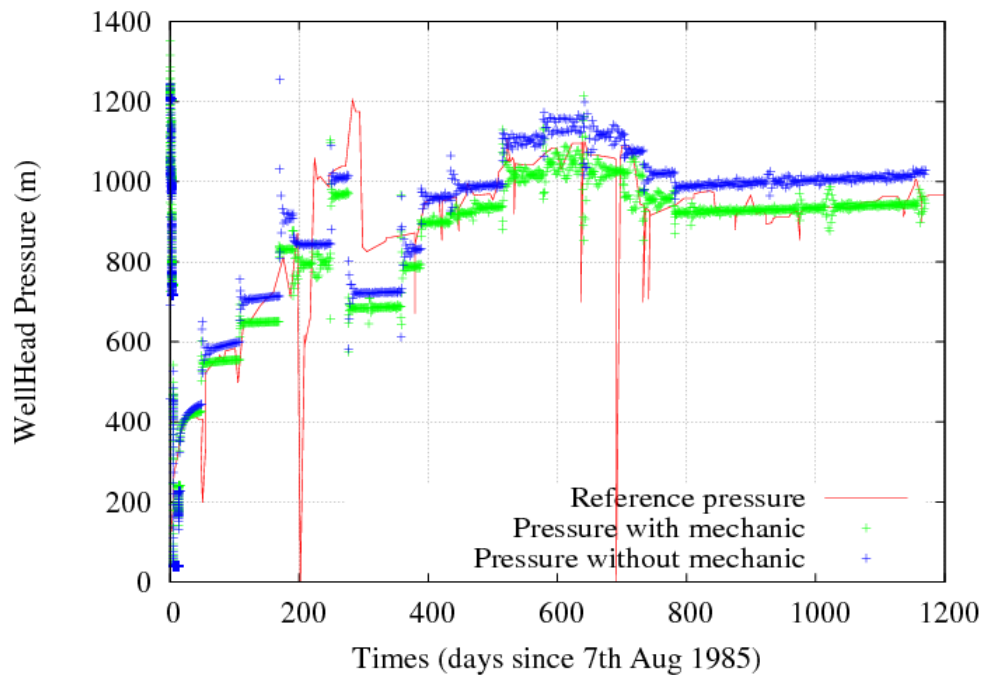
Figure 3.16 : Pression de production du modèle, avec le couplage mécanique (vert) et sans le couplage mécanique (bleu) et données de terrain (rouge) ( 100\text{ m} = 1\text{ MPa} )
