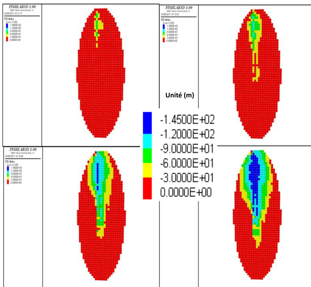
Figure 3.24 : Evolution de la contrainte thermique, au cours des 3 années de tests de circulation divisées en 4 périodes de durée de 300 jours, sur la fracture de production A3 (N165), en partant du gauche vers la droite et du haut vers le bas
