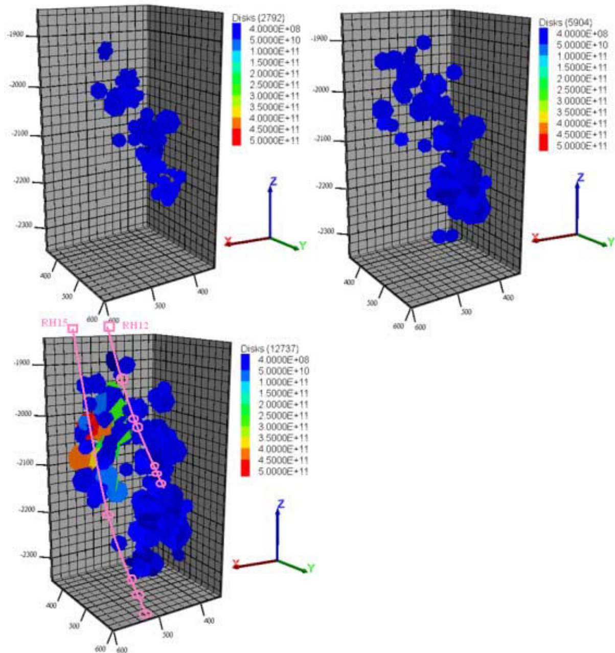
Figure 3.36 : Evolution des lieux des ruptures et des moments sismiques durant le test de circulation suivant l'hypothèse PTC de pression et température constante, en partant du gauche vers la droite entre les dates de 0 et 1 an, entre 1 et 2 ans et entre 2 et 3 ans. En rose, le puits d'injection RH12 et de production RH15 avec, superposées, les traces des disques d'entrée et sortie.
