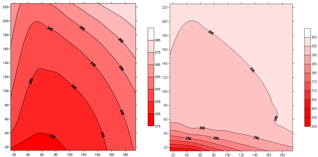
Figure 2.14 : Carte de température T_m dans le bloc continu. A gauche dans la coupe passant par les mailles contenant le plan de fracture et à droite par une coupe parallèle, passant par les mailles situées à la distance de 30 m dans le massif, obtenues à la date de 5 ans.
