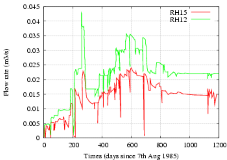
Figure 3.8 : Variation du débit d'injection mesuré au pied du casing du puits RH12 (vert) et du débit de production mesuré à la tête du puits RH15 (rouge), durant la circulation principale (C/S=au Pied de tubage ; W/H=à la tête de puits) (Richard et al., 1994)
