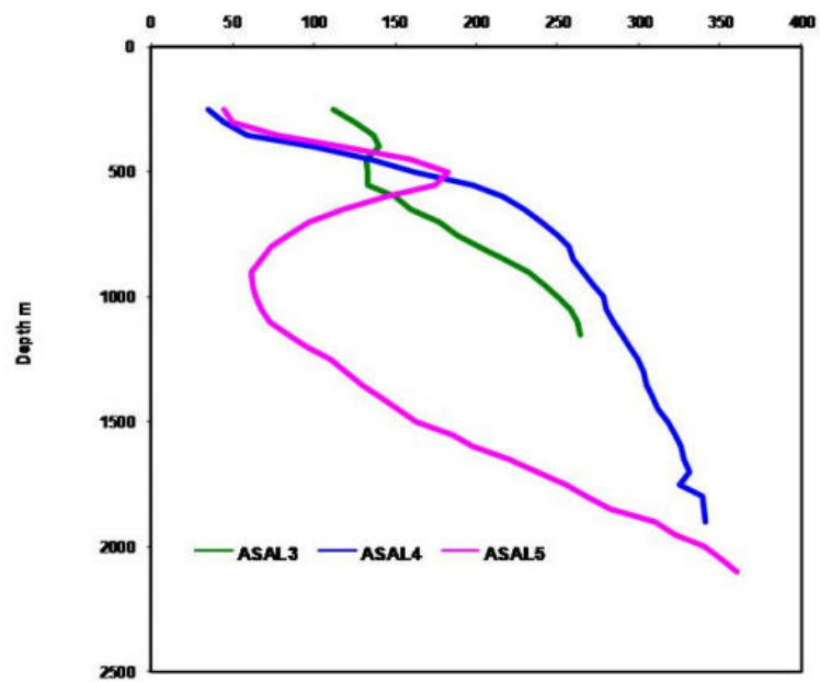
Figure A6 : Profil de température des forages A3, A4, A5 (Aquater, 1989 et cité dans Daher, 2010)
