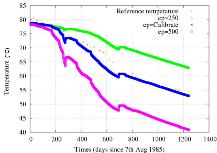
Figure 3.40 : Effet du choix d'une épaisseur égale pour toutes les familles. Température de production pour différentes valeurs du paramètre épaisseur, les données de terrain étant en rouge
