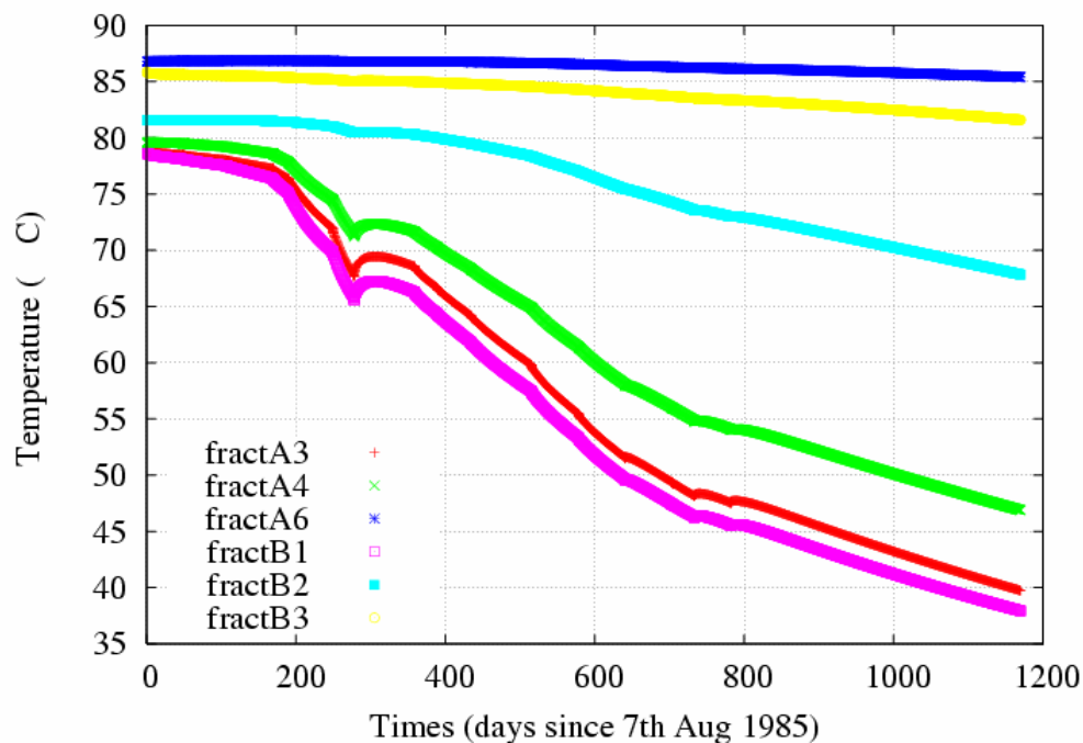
Figure 3.21 : Température de production dans les 6 fractures de production
