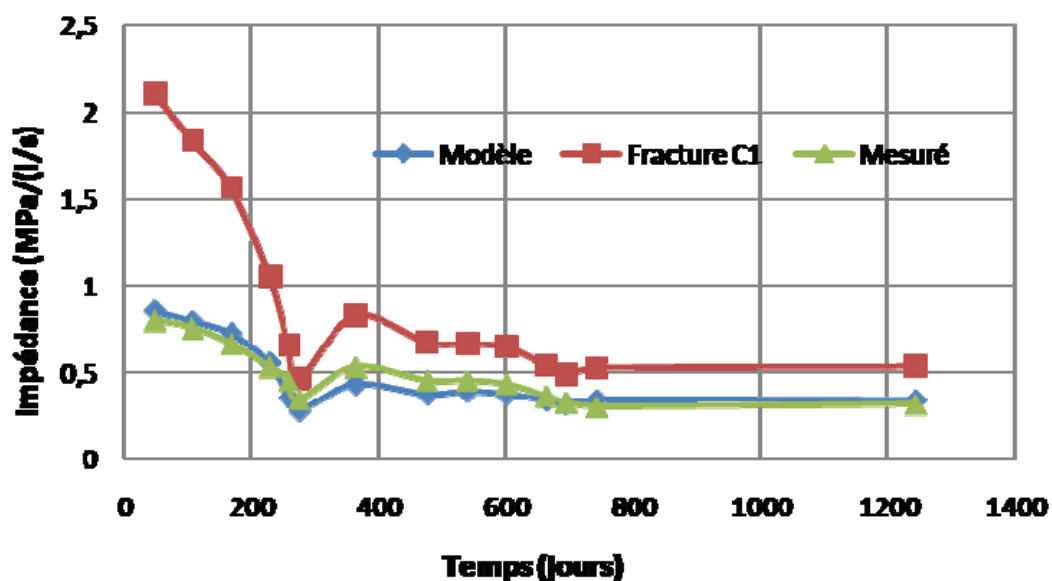
Figure 3.18 : Evolution de l'impédance hydraulique du doublet RH12/RH15 au cours du temps et rôle de la fracture C1 dans notre modèle
