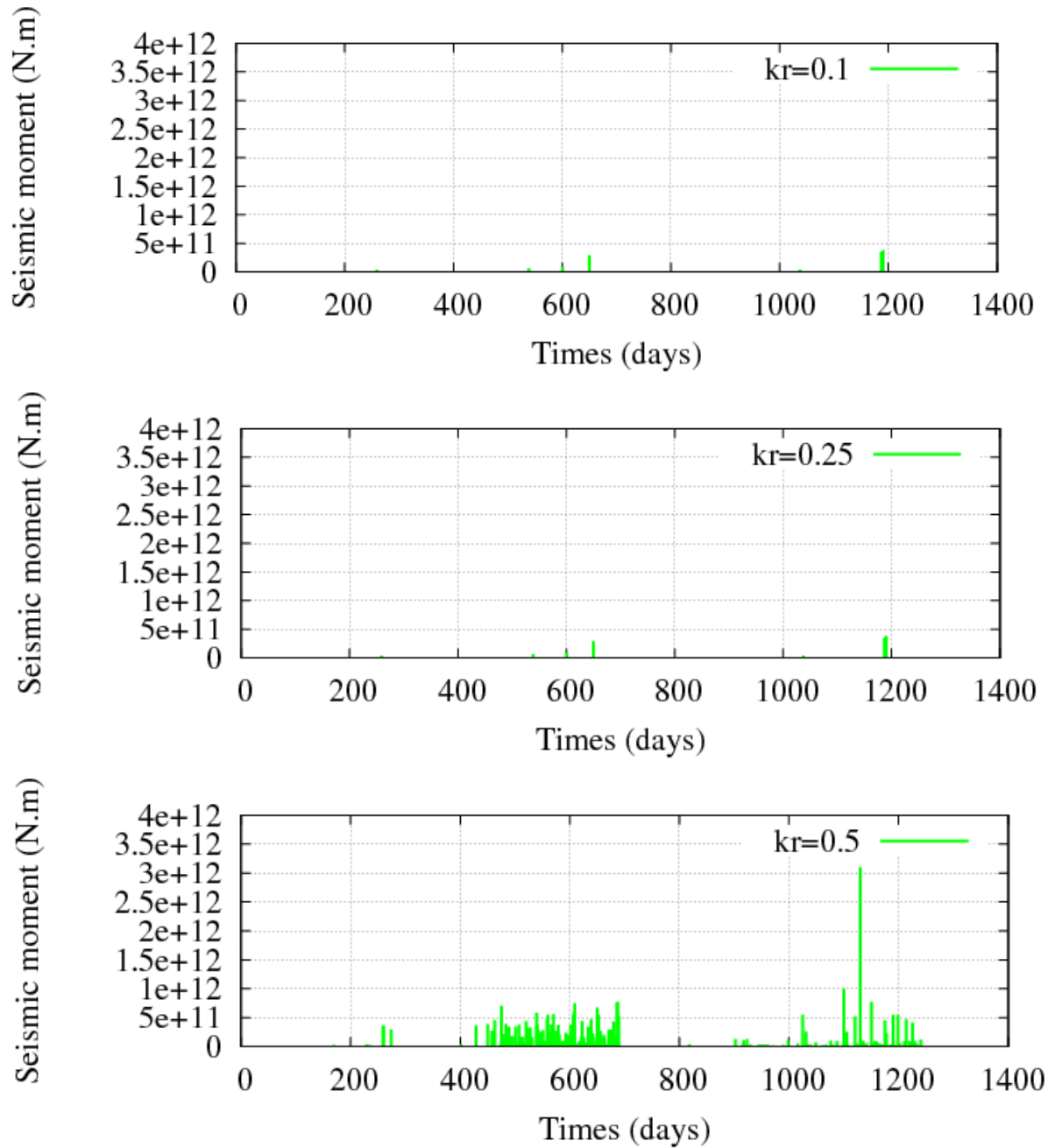
Figure 3.39 : Moments sismiques calculés pendant le test de circulation 2B/2C pour différentes valeurs du coefficient d'abattement Kr
