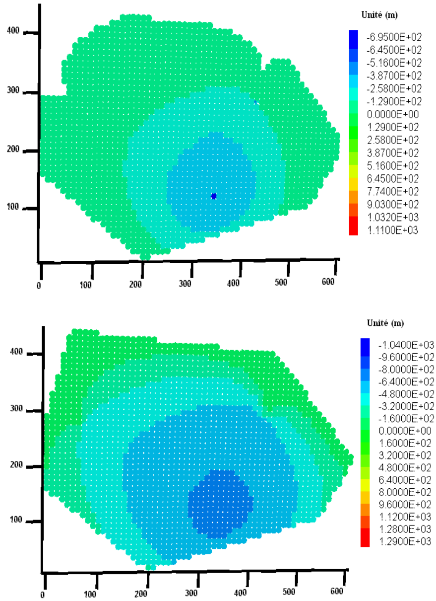
Figure 2.27 : Distributions de la contrainte \sigma_{zz} exprimées en m de colonne d'eau à la surface de la fracture lorsque les temps d'injection de fluides sont de 6 mois et 3 ans respectivement.
