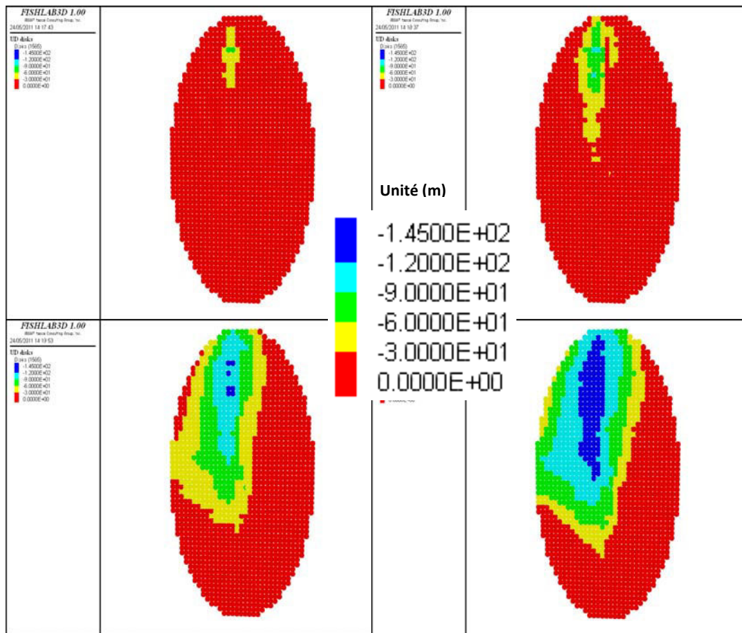
Figure 3.23 : Evolution de la contrainte thermique, au cours des 3 années de tests de circulation divisées en 4 périodes de durée de 300 jours, sur la fracture de production A4 (N165), en partant du gauche vers la droite et du haut vers le bas
