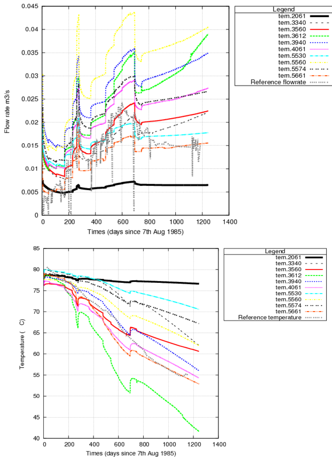
Figure 3.31 : Profils des débits (haut) et des températures (bas) de production calculés au cours du temps, respectivement pour 10 réalisations équi-probables du réseau fracturé, la réalisation 5661 (en rouge pointillé) est celle qui se rapproche le mieux aux données de terrain.
