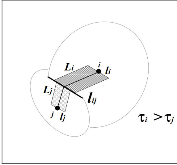
Figure 2.4 : Exemple de deux disques i et j connectés. La largeur des liens est fonction de la longueur du segment d'intersection l_{ij} et du niveau de contrainte normale effective supportée, via les coefficients de degré de séparation \tau_i et \tau_j (Bruel, 1990).
