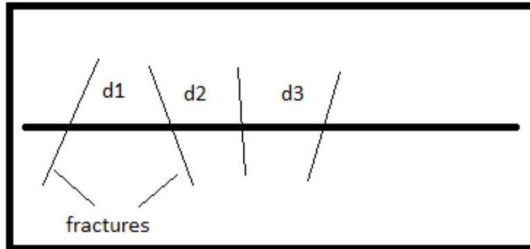
Figure A10 : Définition de la distance inter-fracture (Bourguine et al., 1995) séparant deux traces successives le long d'une ligne d'observation
