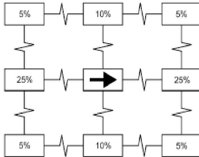
Figure 2.8 : Schéma de redistribution de la chute de contrainte autour d'une portion d'un plan de faille ayant subi un glissement selon Baisch et al. (2010)
