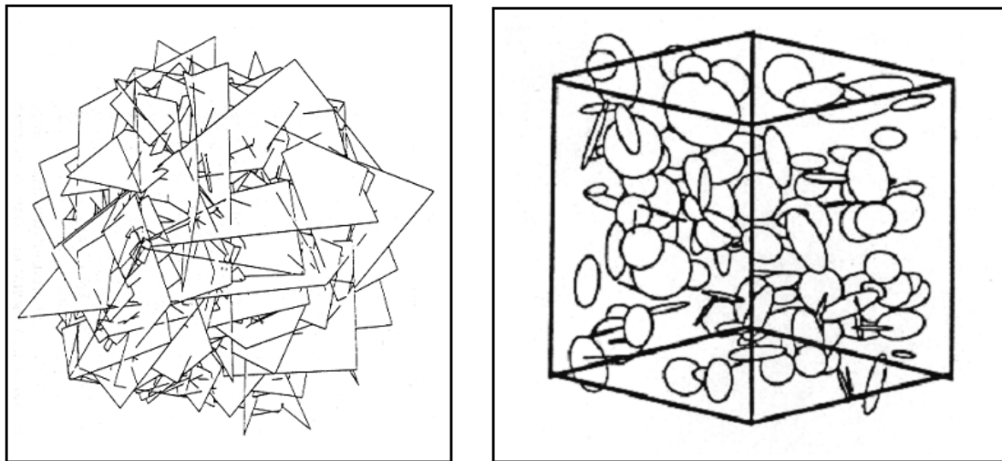
Figure 1.7 : Modèle à réseau de fractures discrètes. À gauche un réseau de fractures polygonales (Stratford et al., 1990) et à droite un réseau de fractures circulaires (Ezzedine, 1994).
