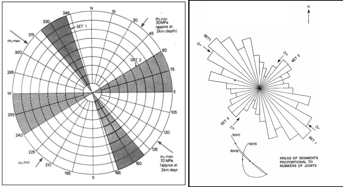
Figure 3.5 : Direction des principales familles des fractures, aux affleurements (gauche) et proportions selon les statistiques obtenues par BHTV dans les puits (droite) en relation avec l'orientation de la contrainte maximum in situ, horizontale dans le SW de l'Angleterre (Parker, 1999)
