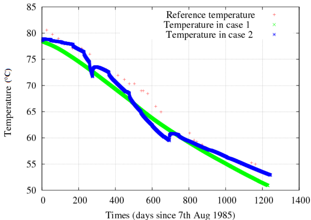
Figure 3.32 : Température de production dans le puits RH15 au cours du temps à partir du modèle stochastique. Dans le cas 1, PTC, pression et température d'injection sont constantes. Dans le cas 2, PTV, la température et la pression d'injection sont variables selon l'historique de la Figure 3.29.
