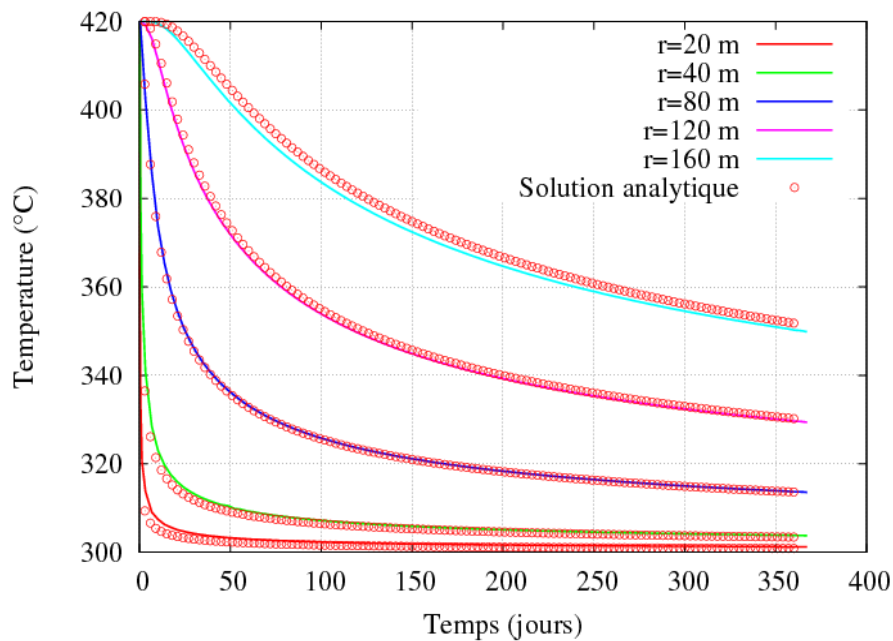
Figure 2.10 : Distribution de la température \theta_f dans une fracture infinie et à différentes distances du point d'injection en fonction du temps, entre 0 et 1 an.
