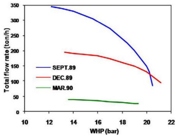
Figure A5 : Courbe de production du forage A3, (Aquater, 1989 et cité dans Daher, 2010)
