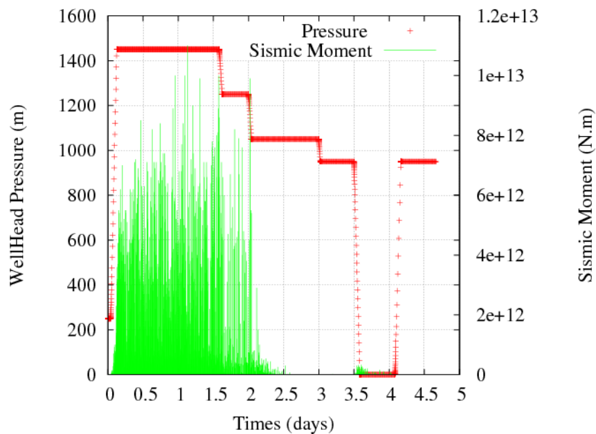
Figure 3.29 : Test de stimulation hydraulique RT2A046 04/11/82 10:00 - 09/11/82 09:40. En rouge la pression d'injection appliquée au réservoir en RH12 et en vert les pulses illustrent le moment sismique de chacune des ruptures obtenues numériquement au cours du temps pendant cette simulation.
