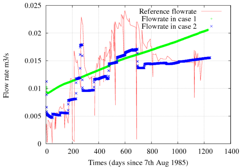
Figure 3.33 : Débit de production dans le puits RH15 à partir du modèle stochastique. Dans le cas 1, pression et température d'injection sont constantes. Dans le cas 2, la température et la pression d'injection sont variables).
