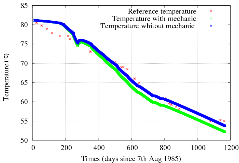
Figure 3.17 : Température de production du modèle, avec le couplage mécanique (vert) et sans le couplage mécanique (bleu) et données de terrain (rouge)
