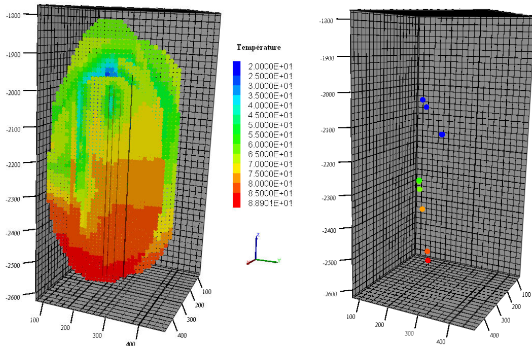
Figure 3.11 : (a) Modèle à 11 fractures majeures, La couleur se réfère à la température simulée à l'instant final des calculs. On voit le haut de la zone froide (bleu), qui marque une des entrées (fracture C1) dans le modèle par le puits RH12. (b) Localisation des points d'entrée (froid) et de sortie, précisée dans les Tableau 3.2 et Tableau 3.3. L'axe X, rouge, pointe vers l'Est, l'axe Y, en vert, pointe vers le Nord.
