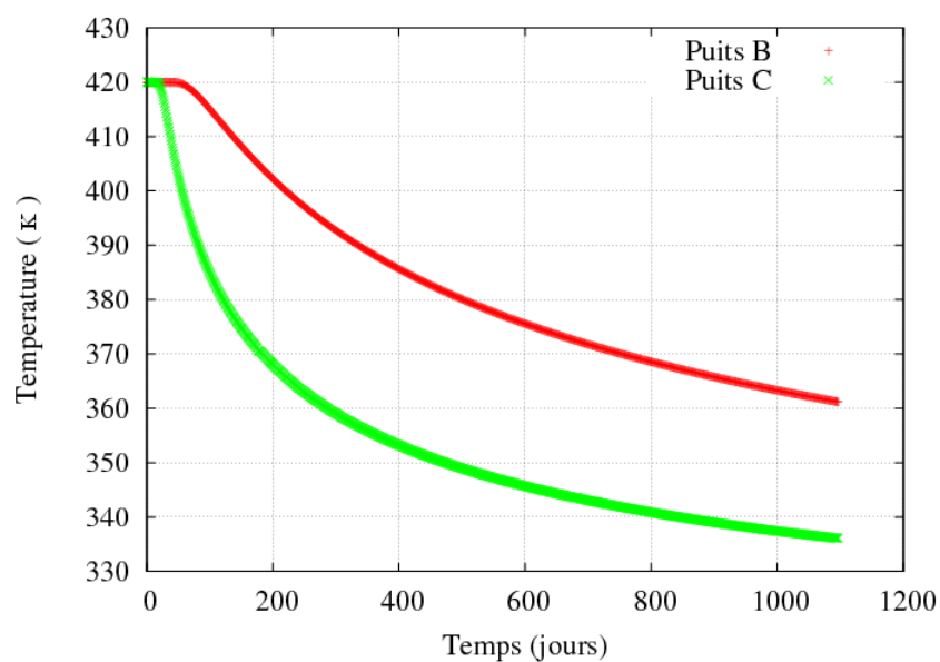
Figure 2.28 : Profils de température de production dans les puits de production et au bout de 3 années d'injection selon le code FRACAS.
