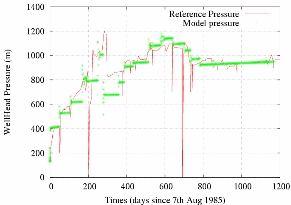
Figure 3.13 : Pression d'injection calculée au puits selon le modèle (vert), données de terrain (rouge) et résultats obtenus en ne tenant pas compte du couplage thermo-élastique (100 m = 1MPa)
