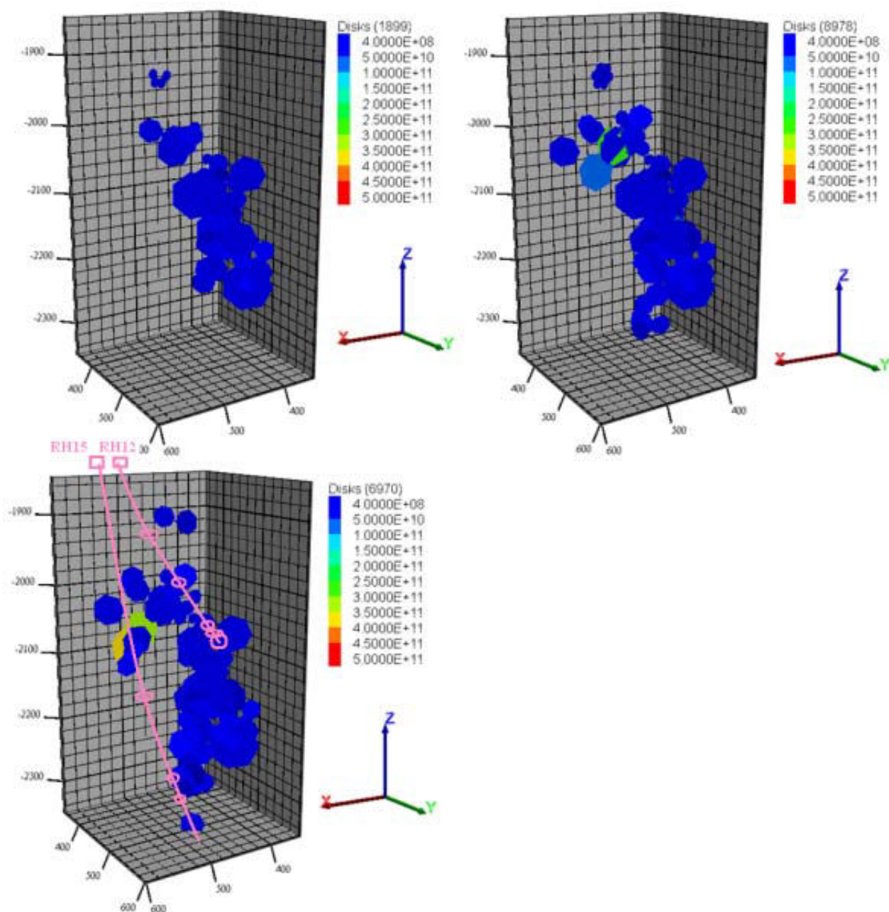
Figure 3.35 : Evolution dans l'espace des lieux de rupture et des moments sismiques durant le test de circulation avec l'hypothèse PTV. En partant de la gauche vers la droite, évènements obtenus entre la date 0 et la date 1 an, évènements entre la date 1 an et la date 2 ans, évènements obtenus entre la date 2 ans et la date 3 ans. En rose, le puits d'injection RH12 et de production RH15, avec, superposées, les traces des disques d'entrée et sortie. La gamme de couleur est relative au moment calculé de la rupture.
