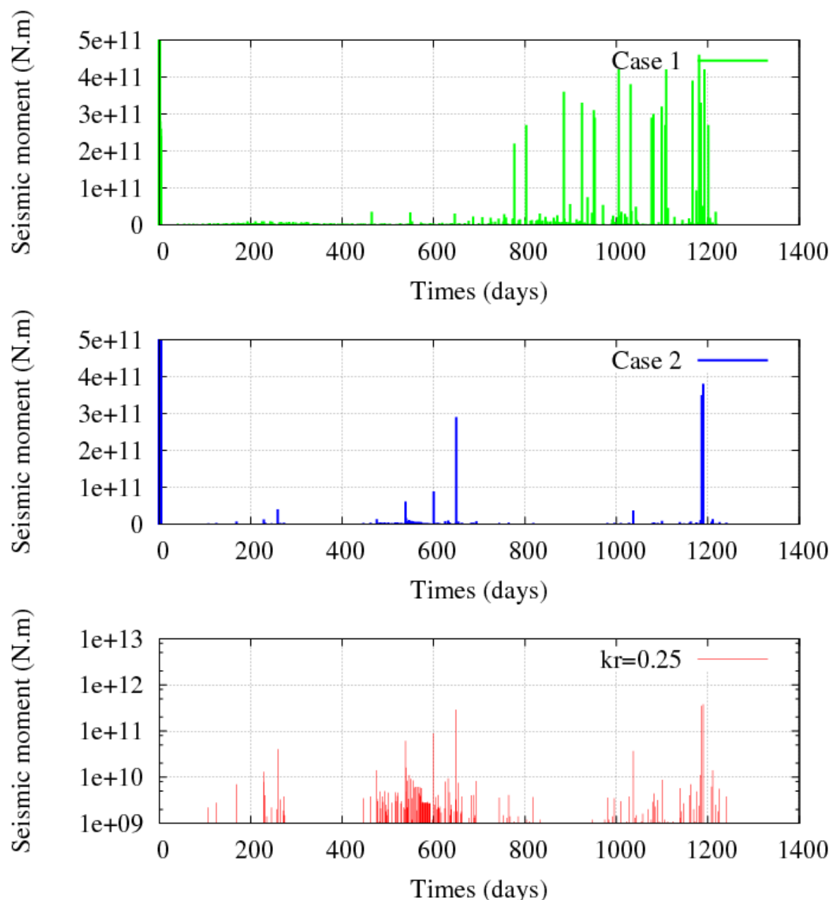
Figure 3.34 : Moments sismiques simulés pour le test de longue circulation. Cas 1 (Haut), avec une pression et température moyenne constante tout au long du test. Cas 2 (Milieu), avec la température et la pression d'injection variables au cours du temps et Cas 3 (Bas), même situation dans une échelle logarithmique pour les moments, montrant mieux l'apparition des événements de rupture en trois bouffées successives.
