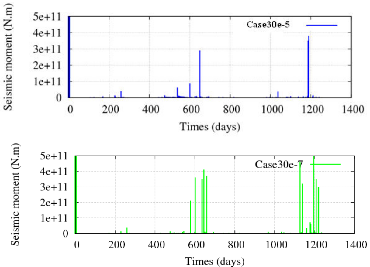
Figure 3.42 : Moment sismique pour le test de longue circulation principale (3 ans), pour différentes valeurs de densité de la famille « court-circuit »
