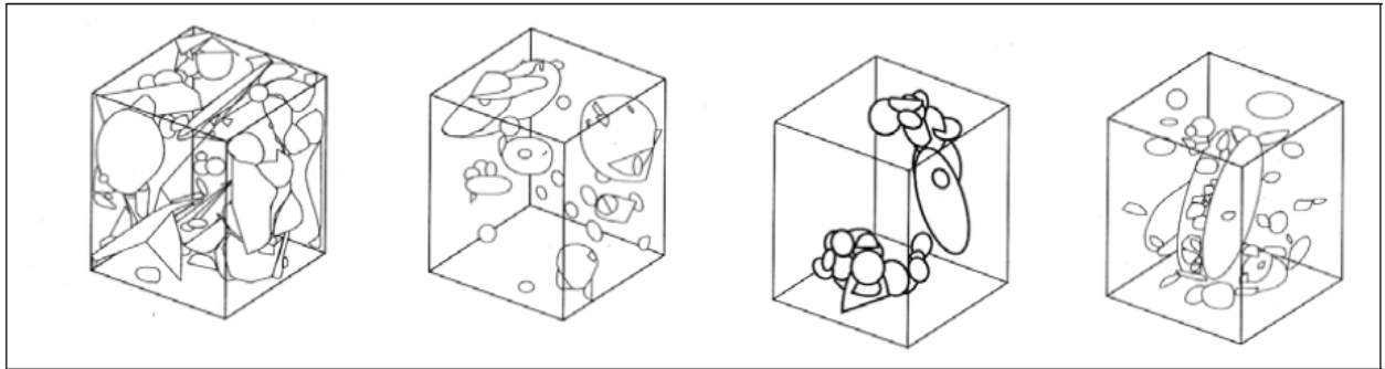
Figure 2.2 : Modèles conceptuels présentant une non uniformité de la densité spatiale des fractures, de gauche à droite : le modèle de poisson stationnaire, le modèle de poisson non stationnaire, le modèle de Levy-Lee fractal et le modèle dit de « war zone » (Dershowitz et Miller, 1995).
