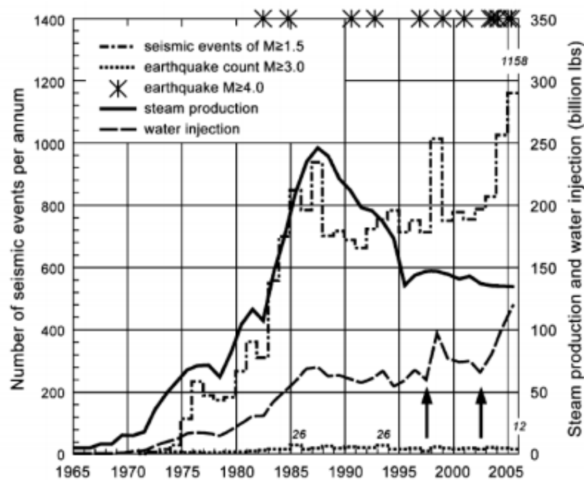
Figure 1.10 : Historique de la sismicité de 1965 à 2006 au Geyser. Les deux flèches indiquent les augmentations de l'injection de fluide en 1997 et 2002 (Majer et al, 2008).
