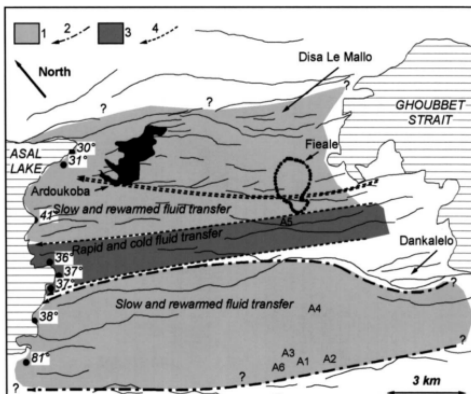
Figure A1 : Représentation schématique de la circulation des eaux souterraines entre le Ghoubbet et le lac Assal. 1: Anomalie positif SP qui correspond à la circulation faible des eaux souterraines chauffées. 2 : Limites de l'anomalie de SP. 3 : Anomalie SP négative, correspondant à la circulation rapide des eaux souterraines. 4 : Forte anomalie négative associée à la faille D. (Mlynarski et al., 2001)
