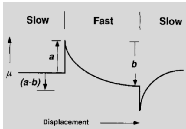
Figure 1.16 : Diagramme schématisant de la loi de friction « rate/state » (Scholz, 1998).
