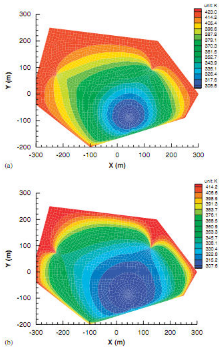
Figure 2.24 : Distributions de la température du fluide dans la fracture lorsque les temps d'injection de fluides sont de 6 mois (haut) et 3 ans (bas) (Zhou et al., 2009)
