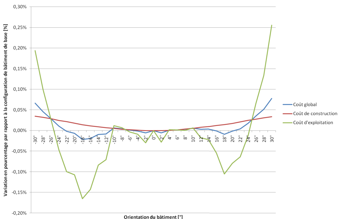
Figure 4.5. Variation en pourcentage des indicateurs économiques pour la configuration de bâtiment de base en fonction de l'angle d'orientation pour valeurs entre -30° et 30°.
