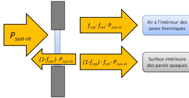
Figure A.2. Répartition de la puissance thermique solaire entrant dans l'espace.
