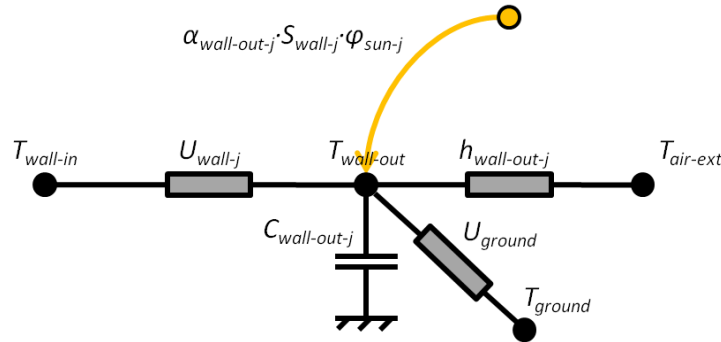
Figure A.5. Bilan thermique du nœud représentant la surface extérieure des parois opaques composant l'enveloppe de la zone thermique.
