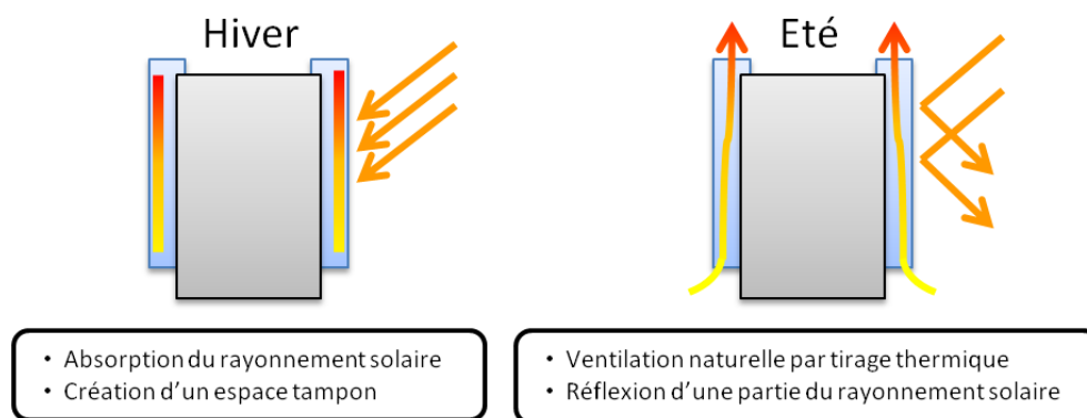
Figure 1.12. Principe thermique d'opération d'une façade double peau vitrée.
