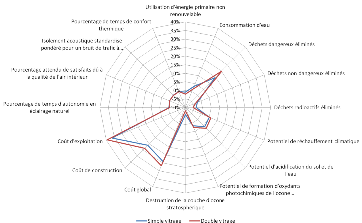
Figure 4.14. Variation en pourcentage des indicateurs de performance en fonction du type de vitrage de la façade double peau vitrée.
