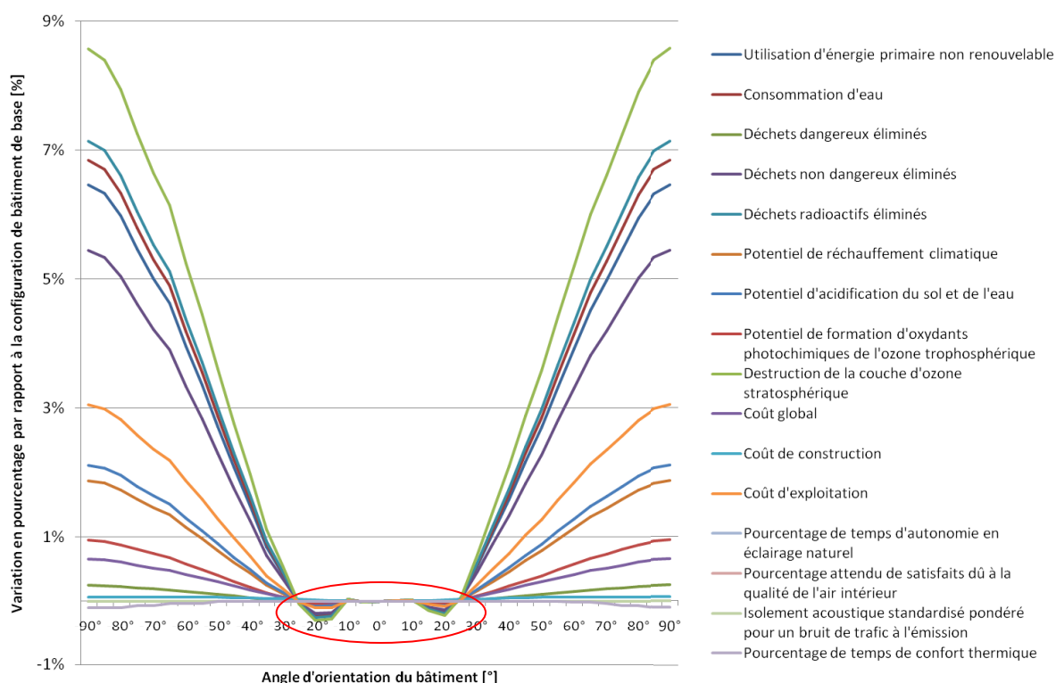
Figure 4.3. Variation en pourcentage de tous les indicateurs de performance pour la configuration de bâtiment de base en fonction de l'angle d'orientation.
