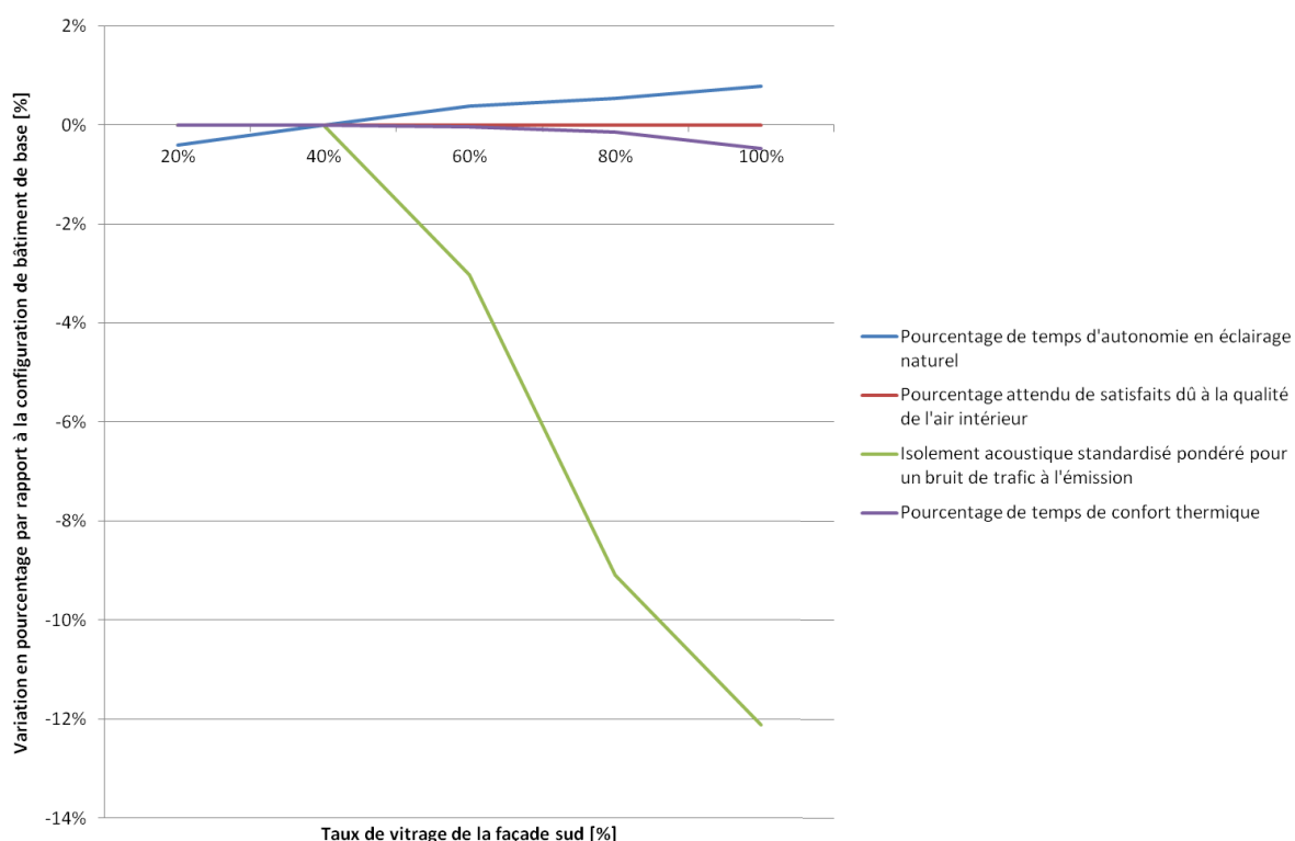
Figure 4.10. Variation en pourcentage des indicateurs de confort des usagers en fonction du taux de vitrage de la façade sud.
