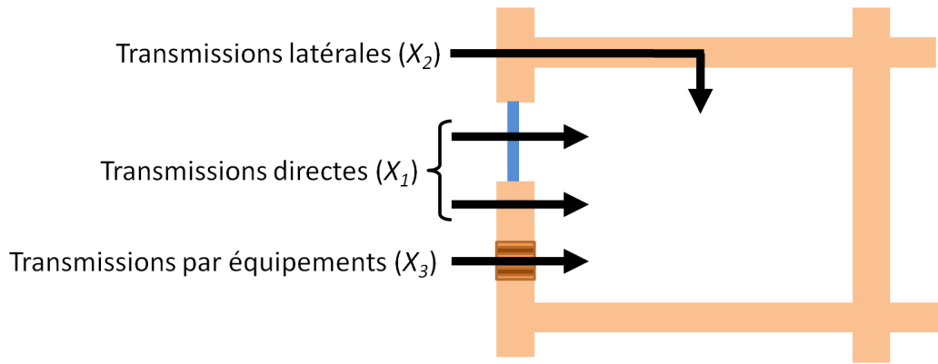
Figure 2.13. Types de transmission acoustique d'un bruit aérien.
