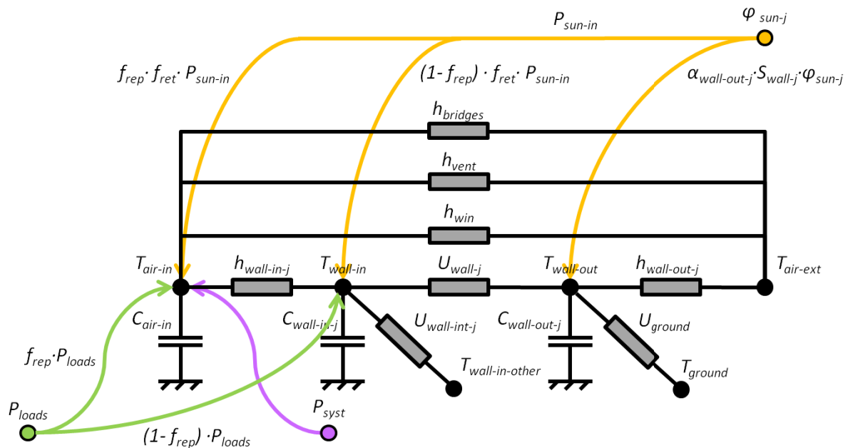
Figure 2.7. Schématisation de la modélisation thermique d'une zone thermique quelconque par analogie électrique.
