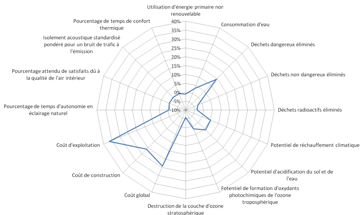
Figure 4.12. Variation en pourcentage des indicateurs de performance dû à la présence de la configuration de base de la façade double peau vitrée.
