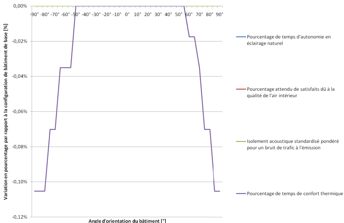
Figure 4.6. Variation en pourcentage des indicateurs de confort des usagers pour la configuration de bâtiment de base en fonction de l'angle d'orientation.
