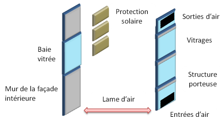
Figure 1.13. Composants principaux d'une façade double peau vitrée.
