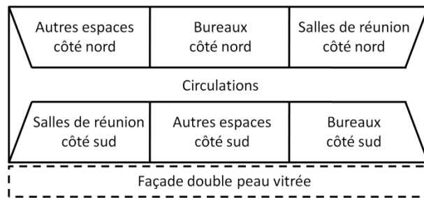
Figure 2.5. Modèle de répartition des zones thermiques.
