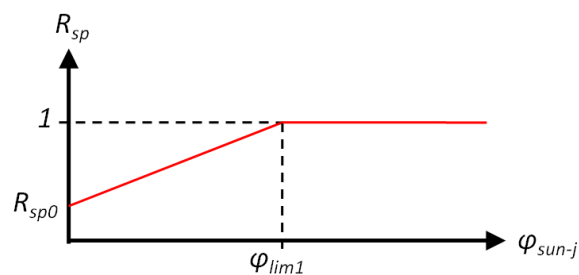
Figure A.7. Comportement du ratio surfacique fermeture des protections solaires de type store enroulable en fonction du flux thermique solaire surfacique.
