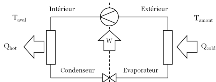
Figure A.9. Schéma d'une pompe à chaleur en mode chauffage.
