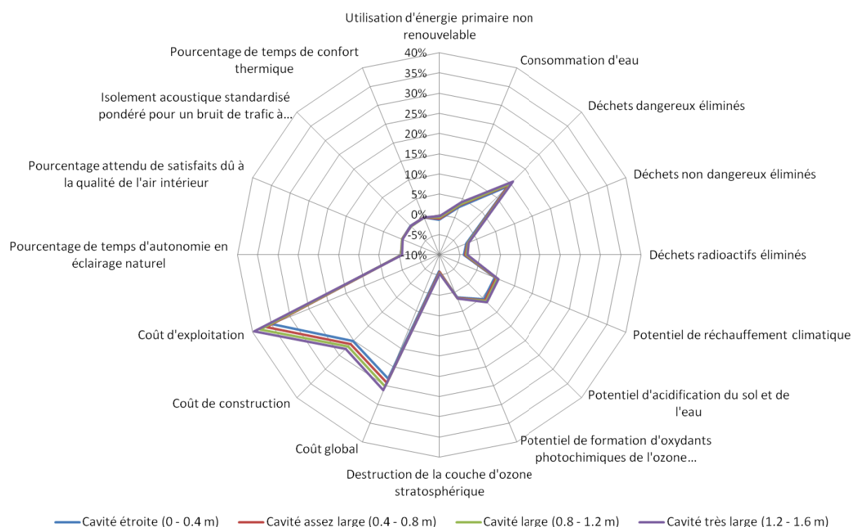
Figure 4.15. Variation en pourcentage des indicateurs de performance en fonction de l'épaisseur de la cavité d'air entre façades.
