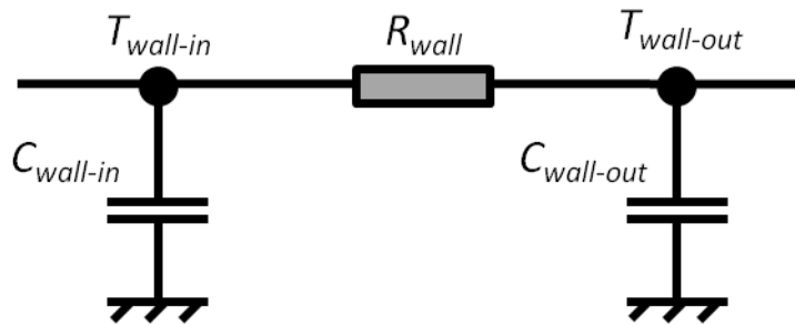
Figure 2.6. Modèle thermique d'une paroi opaque selon le principe de l'analogie électrique.
