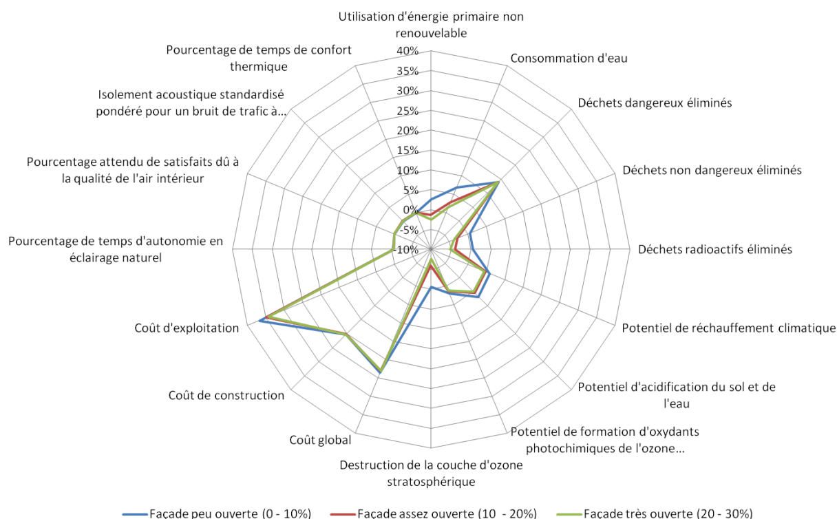
Figure 4.17. Variation en pourcentage des indicateurs de performance en fonction du pourcentage d'ouverture de la façade vitrée.
