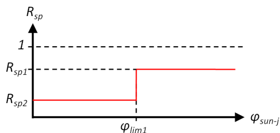
Figure A.8. Comportement du ratio surfacique fermeture des protections solaires de type store vénitien extérieur en fonction du flux thermique solaire surfacique.
