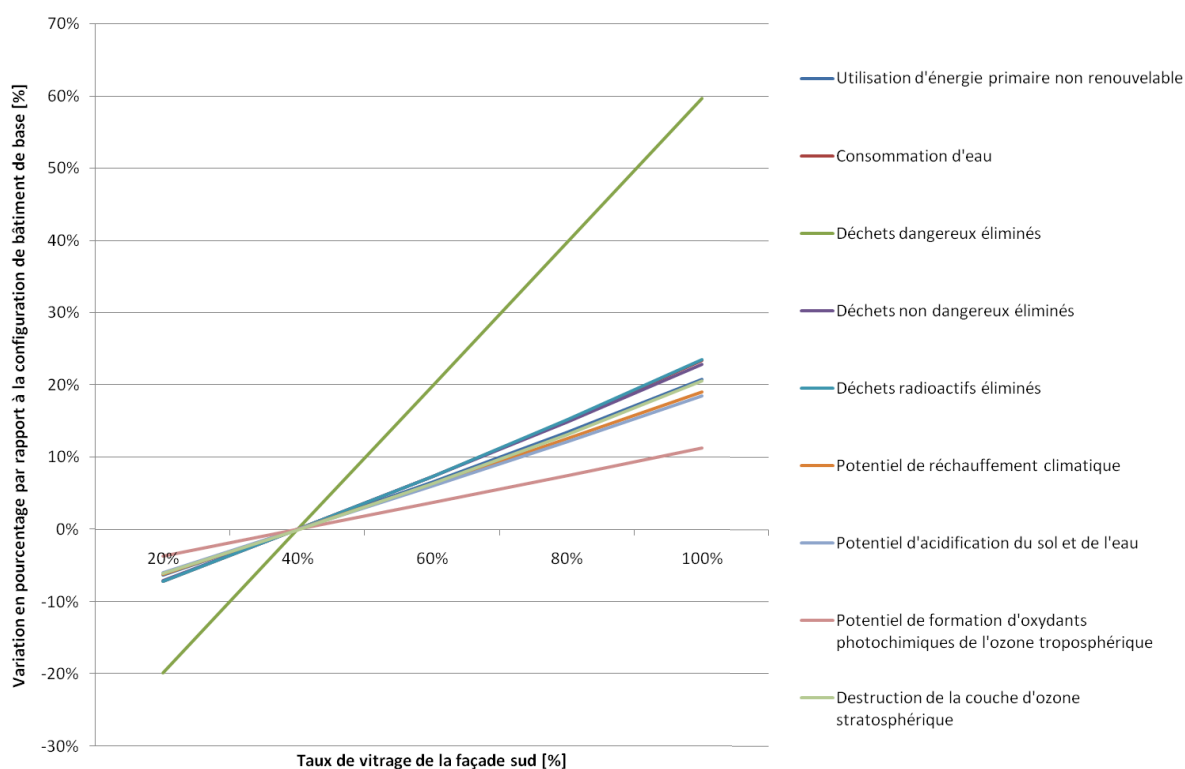
Figure 4.8. Variation en pourcentage des indicateurs environnementaux en fonction du taux de vitrage de la façade sud.
