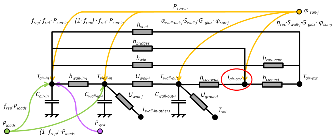
Figure 2.8. Schématisation de la modélisation thermique pour une zone thermique en contact avec une cavité d'une façade double peau vitrée.
