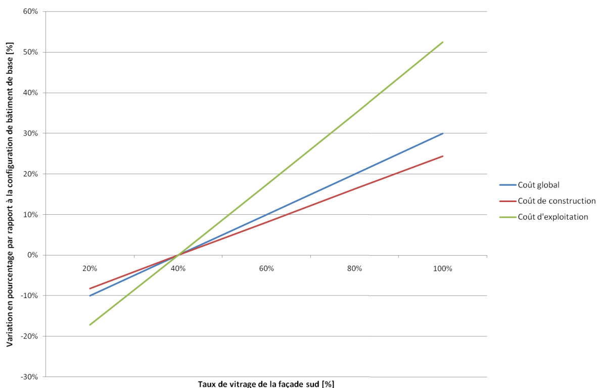
Figure 4.9. Variation en pourcentage des indicateurs économiques en fonction du taux de vitrage de la façade sud.
