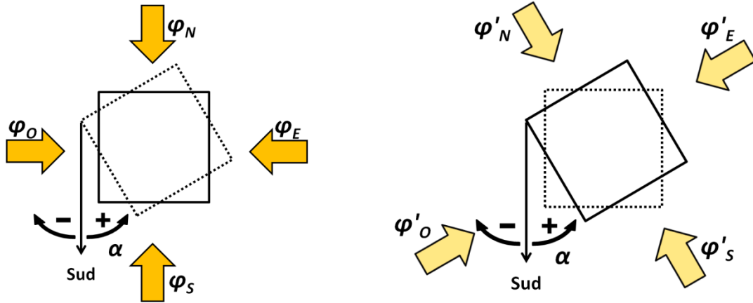
Figure A.11. Correction des valeurs de rayonnement solaire due à une variation de l'angle d'orientation du bâtiment.
