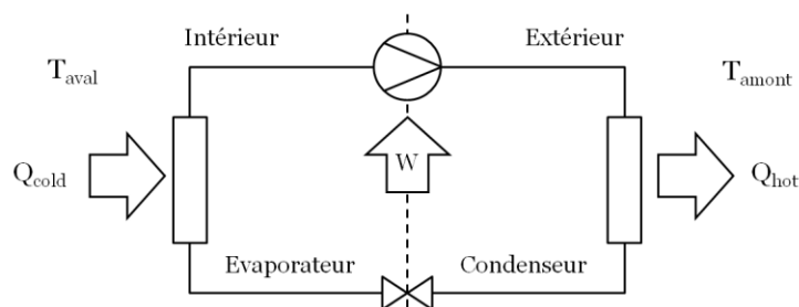
Figure A.10. Schéma d'une pompe à chaleur en mode refroidissement.
