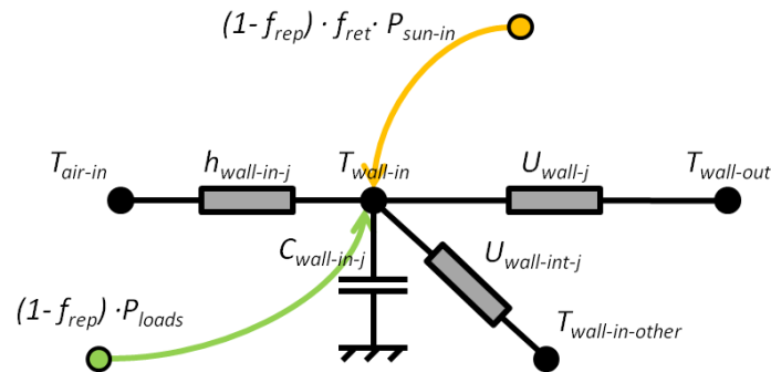
Figure A.3. Bilan thermique du nœud représentant la surface intérieure des parois opaques de la zone thermique.
