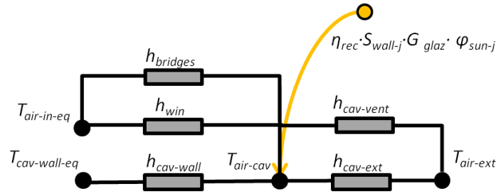
Figure A.6. Echanges thermiques du nœud représentant l'air à l'intérieur de l'espace tampon.
