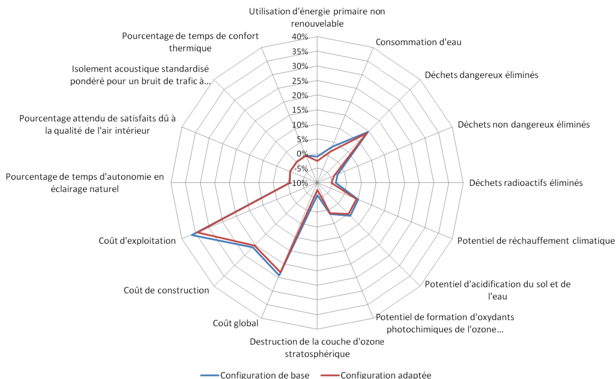
Figure 4.18. Comparaison en variation en pourcentage des indicateurs de performance entre la configuration de façade double peau vitrée de base et son adaptation au contexte de l'exemple du scénario de conception.
