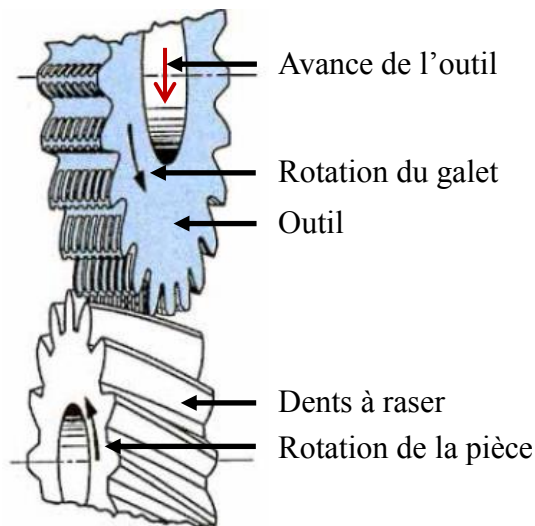
Figure 1.22. Principe du procédé de rasage (d'après [73]).
