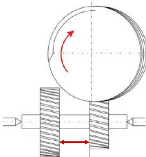
Figure 1.19. Illustration de la longueur maximale utilisable par la meule-mère, indiquée par la double-flèche rouge [72].
