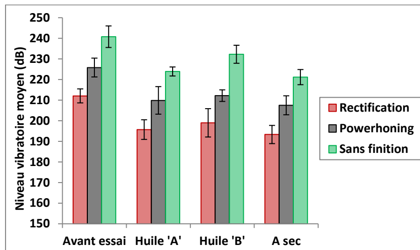
Figure 3.19. Niveaux vibratoires moyens en dB, par rapport à une référence de 1.10^{-6} mm.s 2 , pour des mesures réalisées à une vitesse de 10 mm.s -1 .
