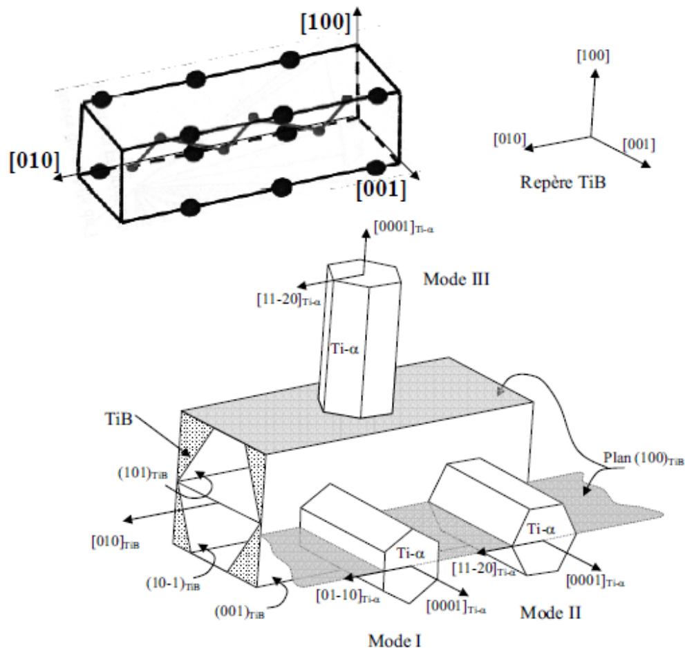
Figure 1-31 : Relations d'orientation entre le TiB et Ti - \alpha et cellule B27 du TiB (Dartigues, 2004)
