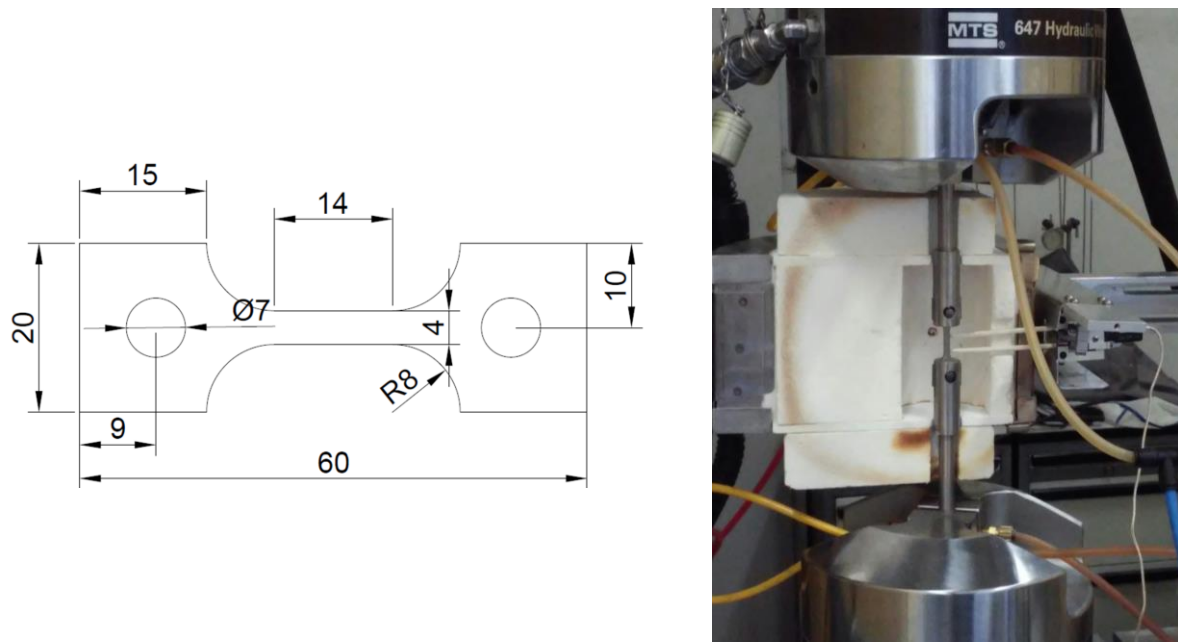
Figure 2-9 : Géométrie des éprouvettes utilisées durant l'étude.
