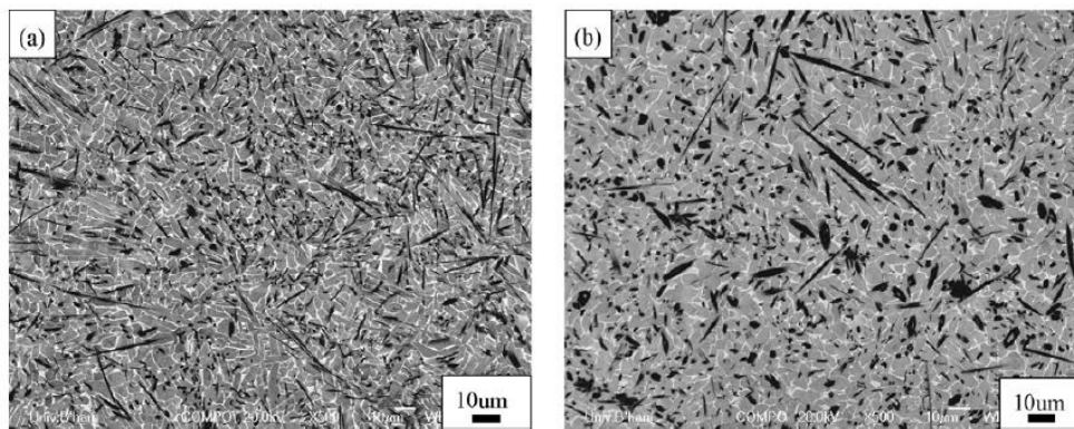
Figure 1-56 : Composites TiB / Ti-6Al-4V obtenus par fusion laser de poudre projetée : (a) 5 % TiB 2 , (b) 10 % TiB 2 (Wang & al., 2008)
