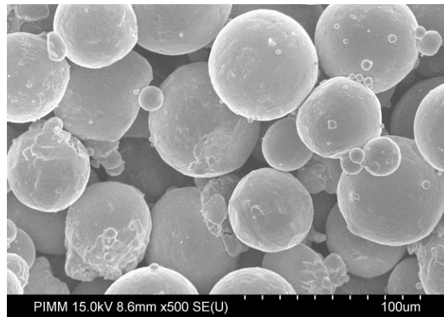
Figure 2-11 : Poudre sphérique de Ti-6Al-4V
