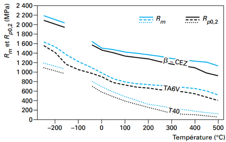
Figure 1-21 : Comportement des alliages de titane (Combres, 1999)
