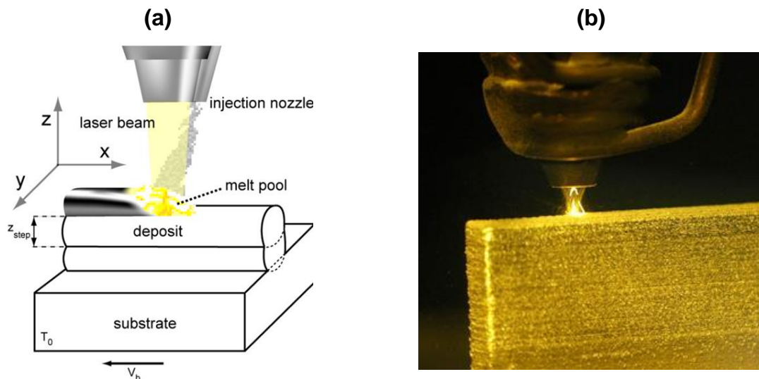
Figure 1-4 : Procédé de fabrication directe par projection laser : (a) schéma du procédé (Mokadem, 2004), (b) procédé en cours (OPTOMECC)
