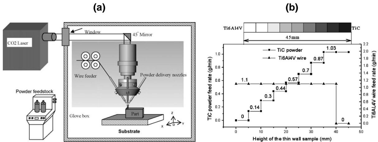
Figure 1-54 : Fabrication Directe de composites TiC / Ti-6Al-4V par fusion laser de fil: (a) dispositif expérimental, (b) Schéma de mise en œuvre du matériau à gradient par variation du débit massique de poudre TiC (Wang & al., 2007)
