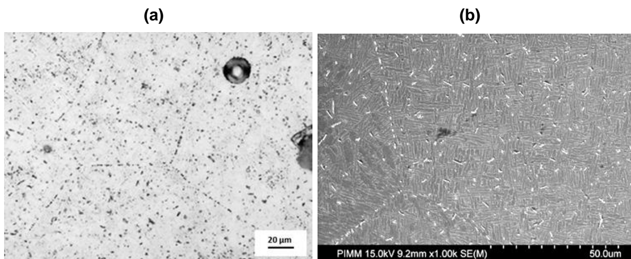
Figure 3-11 : Microstructures Ti-6Al-4V + 10 % TiC (< 10 μm): (a) Microscopie optique, (b) MEB
