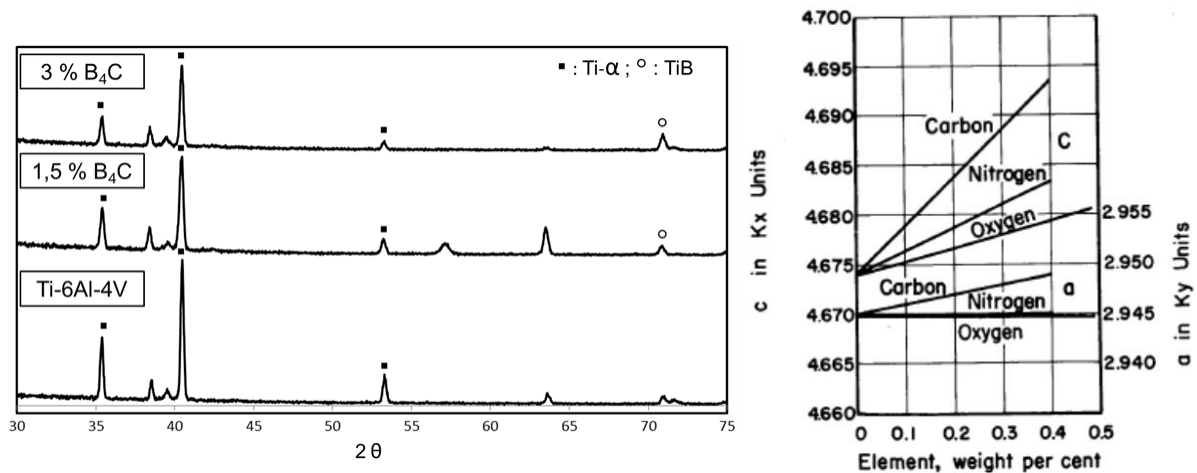
Figure 4-27 : Spectrogramme des différents matériaux réalisés (anticathode de cuivre, \lambda = 1.54 \text{ nm} ) et influence des éléments O, C et N sur les paramètres de mailles (Ogden & Jaffee, 1955)
