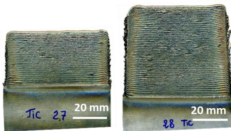
Figure 3-10 : Murs composites Ti-6Al-4V + 10 % TiC (P500V400)
