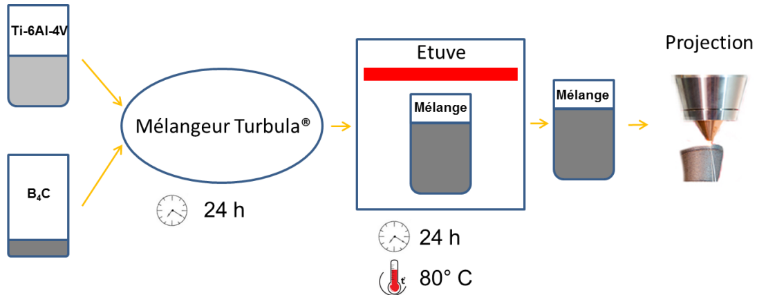
Figure 2-17 : Illustration du principe de mélange Ti-6Al-4V + B_4C
