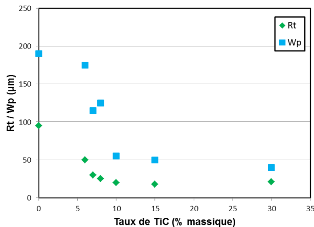
Figure 3-6: Evolution des paramètres d'ondulation W_p et de rugosité R_t en fonction du taux de TiC (P400V200)
