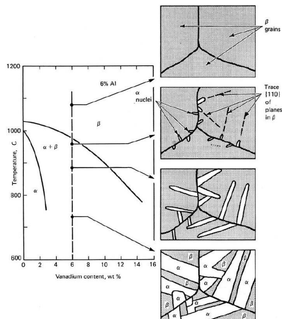
Figure 1-17 : Formation d'une microstructure de Widmanstätten \alpha + \beta lors d'un refroidissement lent depuis le domaine \beta
