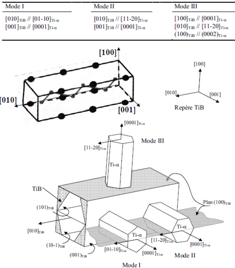
Figure 1-31 : Relations d'orientation entre le TiB et Ti - α et cellule B27 du TiB (Dartigues, 2004)
