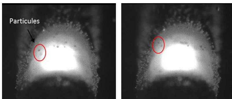
Figure 3-2 : Mouvements centrifuges ( V_p \sim 0.5 m/s) des particules TiC dans les ZF (15 % TiC, particules 100 \mu\text{m} , P400V200 (vue de face, f = 3 kHz)
