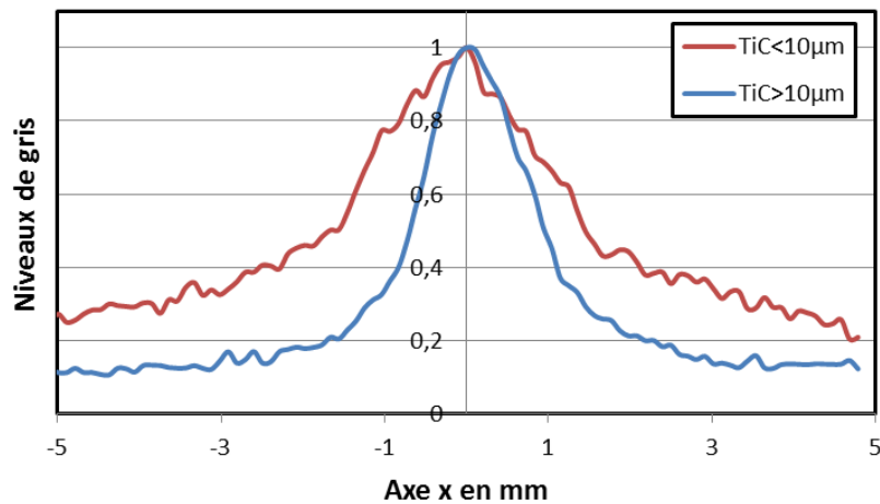
Figure 2-30 : Comparaison par analyse d'image des jets pour des TiC < 10 \mu m et des TiC > 10 \mu m
