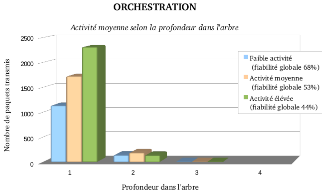
FIGURE 3.14 L'orchestration entraîne un usage intensif des routeurs situés tout en haut de l'arbre, puisque tous les messages remontent au point central, puis redescendent vers un nœud.
