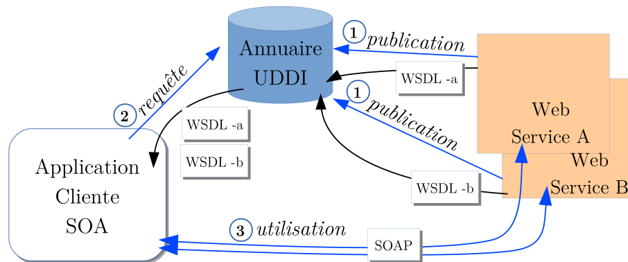
FIGURE 2.2 L'Architecture Orientée Service (SOA). Les services web sont recensés dans un annuaire UDDI qui stocke la description WSDL du service offert. Les applications clientes, après avoir identifié le service recherché, peuvent l'invoquer grâce au format SOAP.
