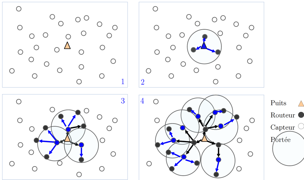
FIGURE 3.8 Notre algorithme pour construire l'arbre se déroule de la façon suivante : le puits (au centre) recherche ses voisins à portée (cercle gris) et les enregistre. À leur tour, ceux-ci cherchent les voisins à portée, et ainsi de suite. Chaque nœud mémorise ses fils, et l'arbre se construit par propagation.
