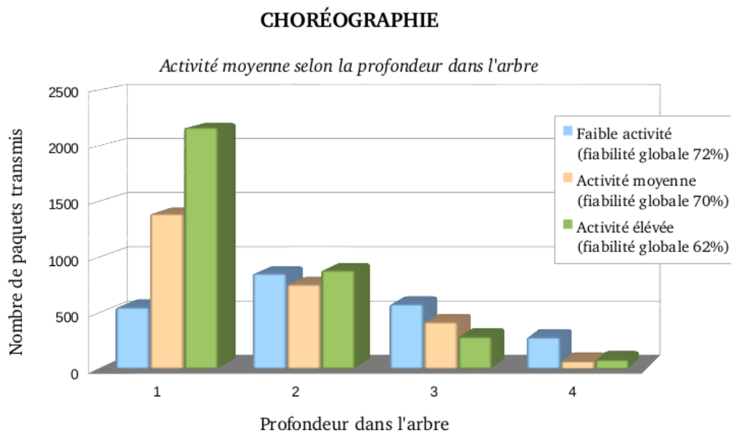
FIGURE 3.15 Dans une chorégraphie, le trafic est mieux réparti sur l'ensemble des profondeurs de l'arbre. La diversité des chemins empruntés par les messages permet d'atteindre un niveau de fiabilité supérieur, car cette architecture favorise moins la formation de goulets d'étranglement.
