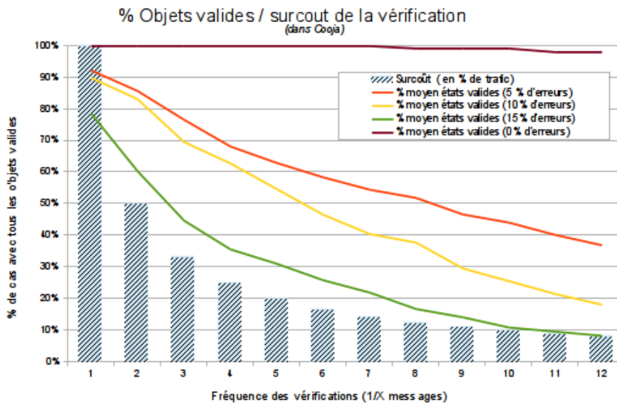
FIGURE 4.18 Les courbes représentent le pourcentage de cas dans lesquelles tous les nœuds ont les bonnes valeurs. Selon le taux d'erreur et la fréquence des vérifications (d'1 vérification par message à 1 pour 12 messages), la courbe donne la précision des valeurs de l'application. Pour obtenir un taux de réponses exactes proche de 70%, une vérification tous les 3 messages est nécessaire si le taux d'erreur est de 10%. Dans les 30% restants, la réponse obtenue cependant reste très proche de la bonne valeur. L'histogramme en bâtons trace le coût de la vérification.
