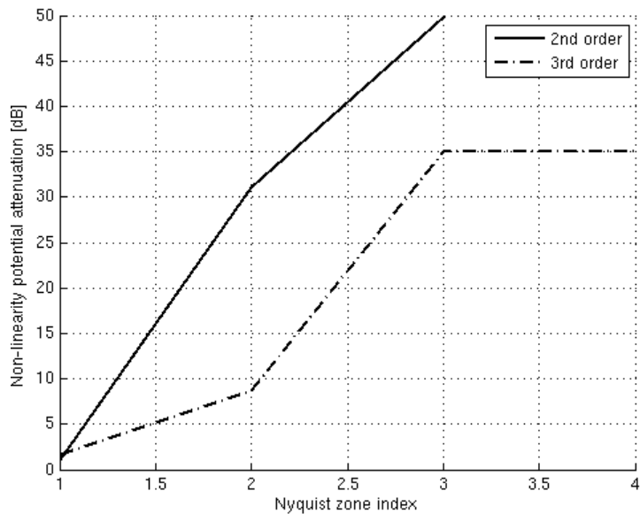
Fig 10. Amélioration potentielle de distorsion non-linéaire, en fonction de la stratégie d'échantillonnage
