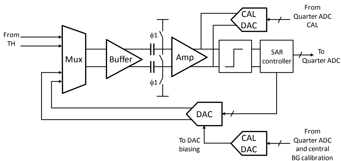
Fig 33. Architecture du convertisseur à approximations successives, et interface avec les échantillonneurs
