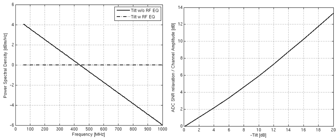
Fig 23. Amplitude des canaux en fonction de l'égalisation RF (gauche, -10dB d'inclinaison). Relâchement de la spécification du SNR d'un CAN grâce à un égaliseur RF (droite)
