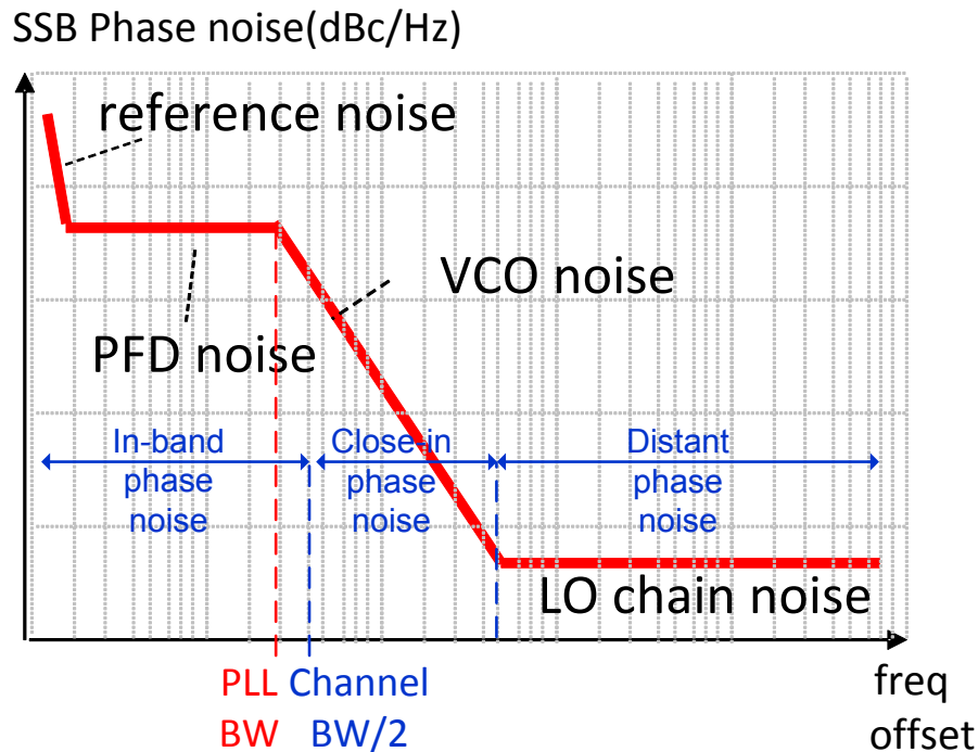
Fig 16. Profil typique de bruit de phase sur une horloge
