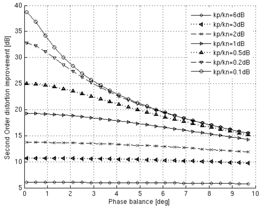
Fig 12. Impact des déséquilibres de gain et de phase sur la distorsion non-linéaire du second ordre
