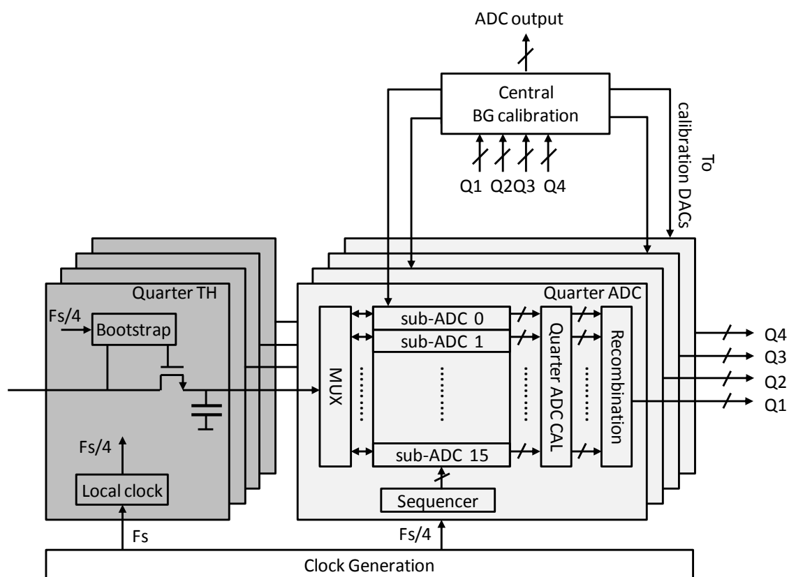
Fig 32. Schéma bloc du CAN
