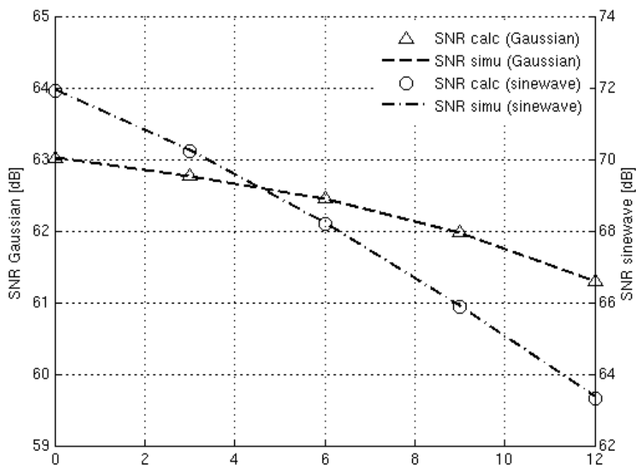
Fig 9. SNR calculé et simulé en fonction de la dégradation de bruit à forts signaux (gauche: signal sinusoïdal; droite: signal gaussien)
