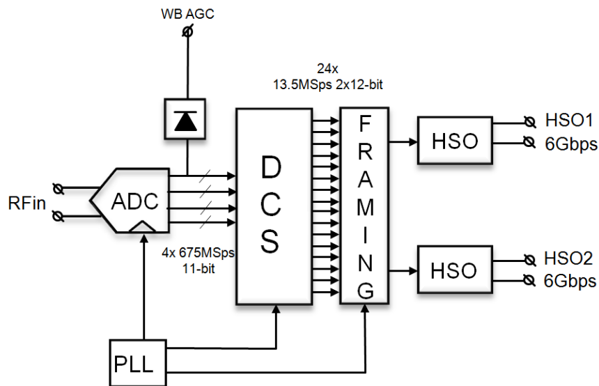
Fig 31. Schéma bloc du frontal à signaux mixtes
