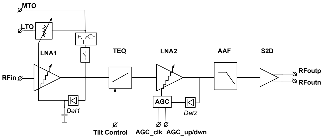
Fig 25. Schéma conceptuel du chemin de réception multi-canaux du frontal RF
