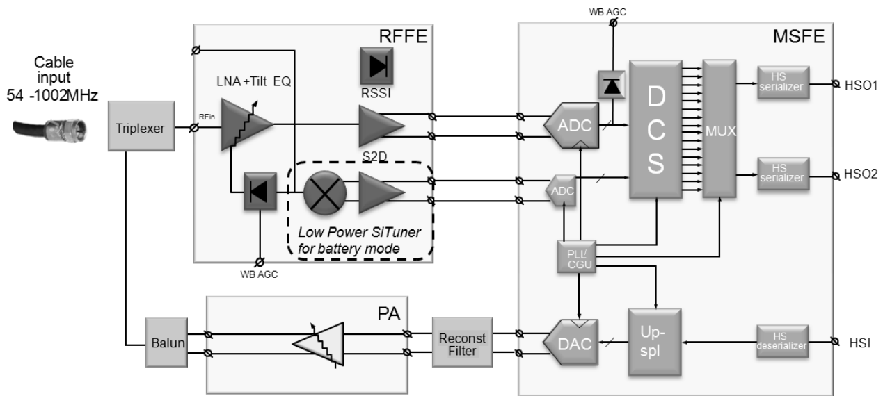
Fig 24. Schéma-bloc du récepteur multi-canaux câble
