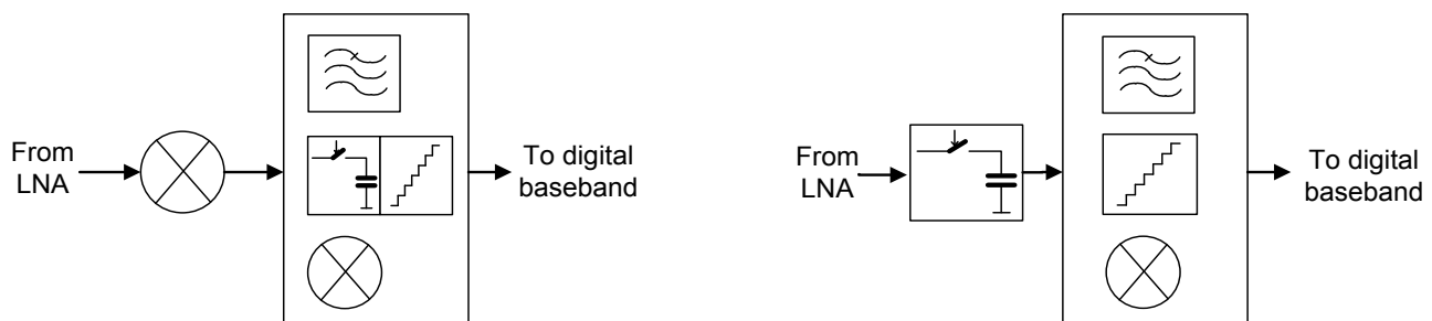
Fig 3. Gauche: récepteur à temps continu, droite: récepteur à temps discret
