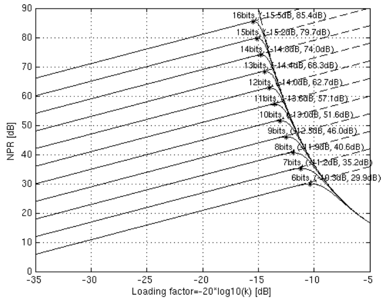
Fig 6. Rapport signal à bruit & facteur de charge optimum pour différentes résolutions de CAN (signal Gaussien)
