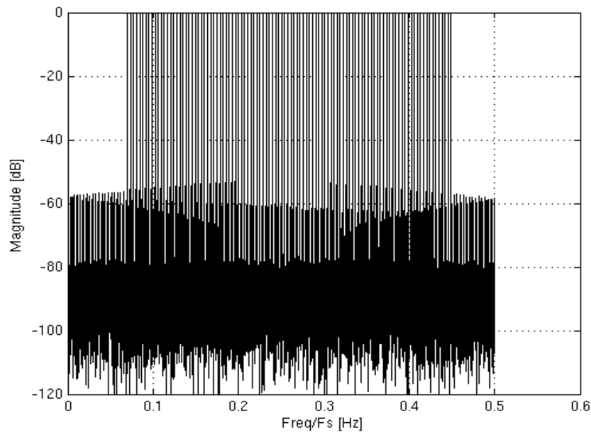
Fig 14. Numérisation d'un signal multi-tons large bande, avec un CAN à 4 canaux, et \sigma_{\text{skew}}=3.5 \times 10^{-4} \times F_s
