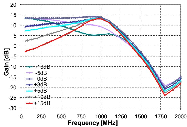
Fig 29. Mesure des fonctions de transfert du frontal RF pour plusieurs programmations d'égaliseur
