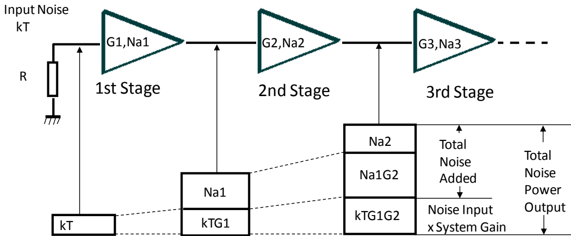
Fig 24. Friis formula
