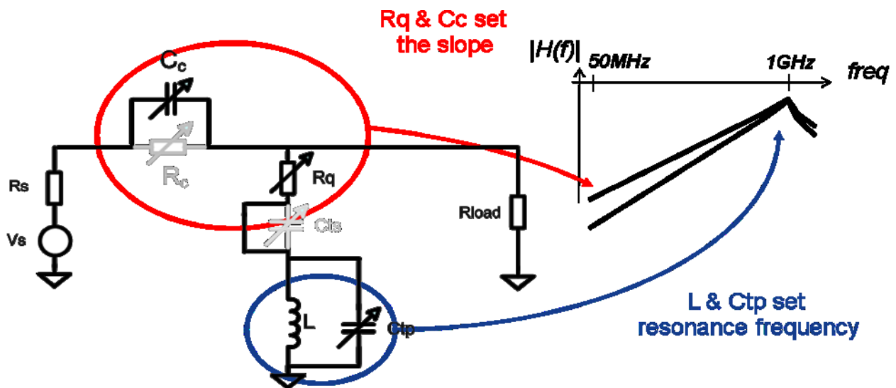
Fig 27. Egaliseur RF configuré dans un résonateur parallèle
