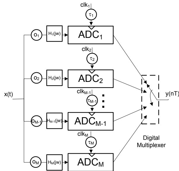
Fig 13. CAN à entrelacement temporel avec désappariage des canaux
