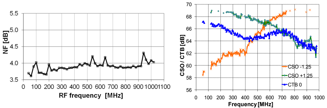
Fig 30. Facteur de bruit du frontal RF (gauche), et CSO/CTB (droite)
