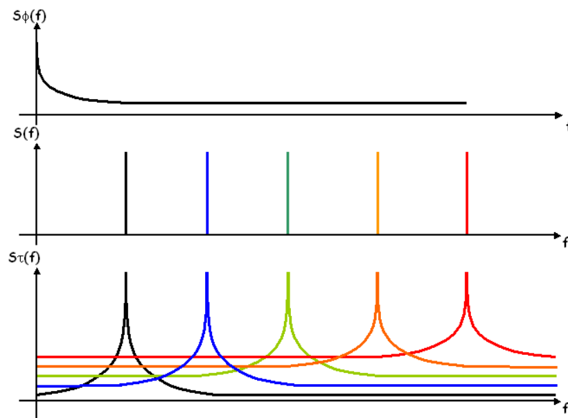
Fig 15. Convolution entre le spectre du bruit de phase de l'horloge et le spectre du signal d'entrée multi-tons
