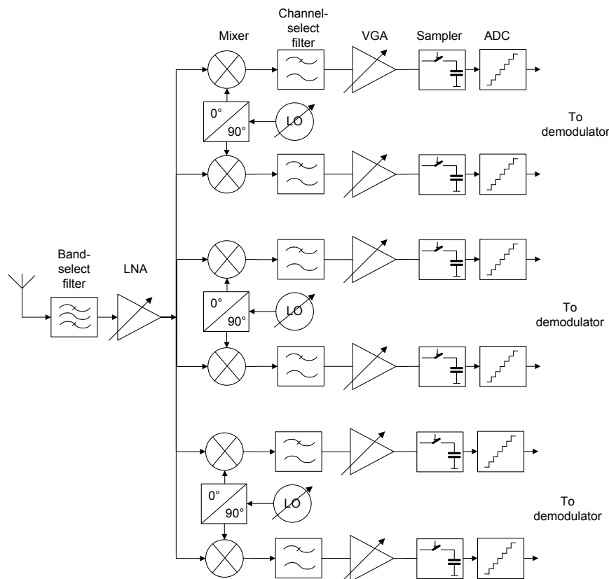
Fig 4. Découpe en sous-bandes avec des mélangeurs et utilisant des signaux analytiques
