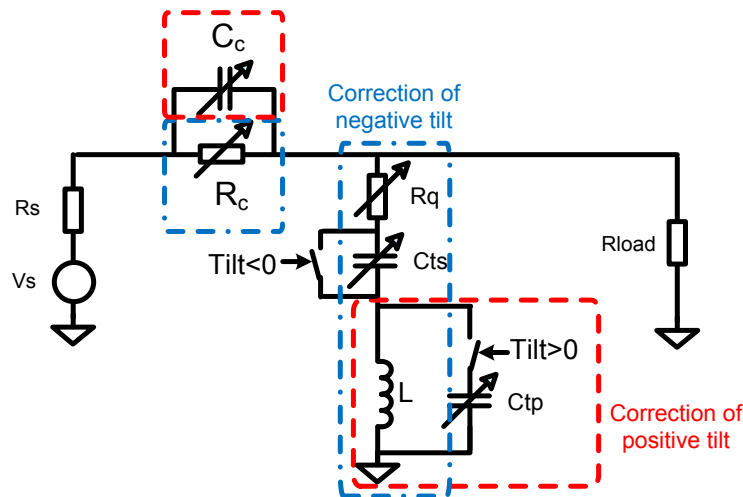
Fig 26. Topologie de l'égaliseur RF
