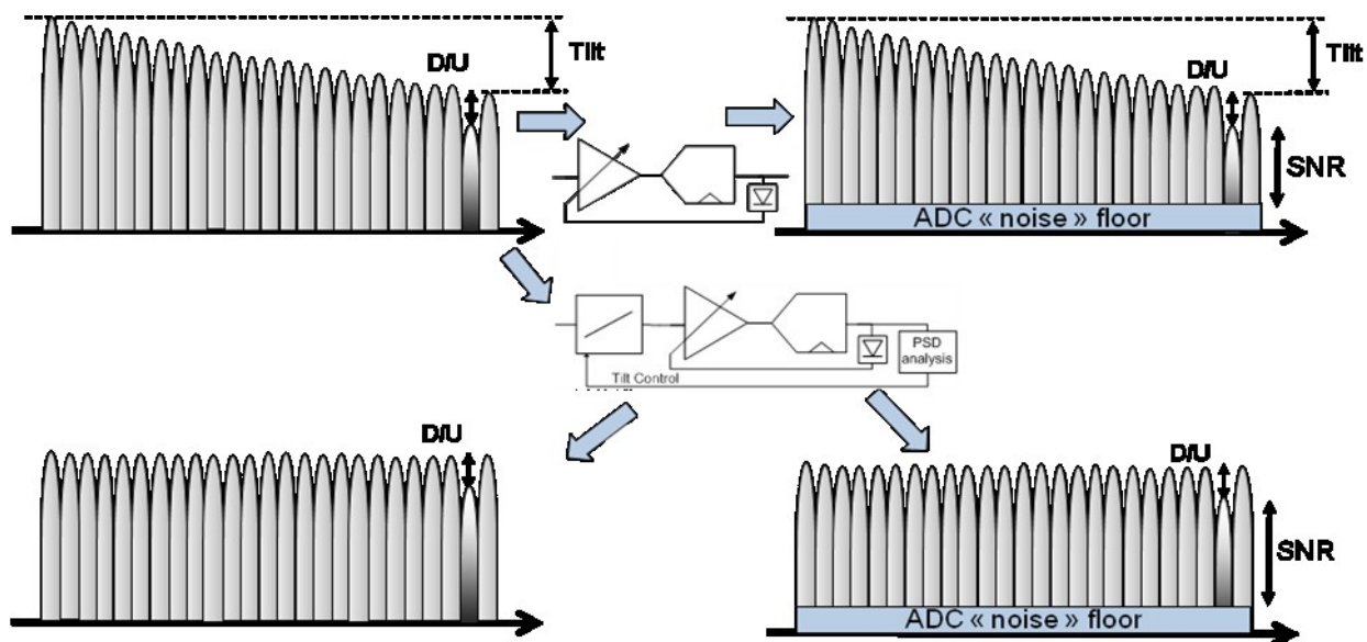
Fig 22. Récepteur à numérisation directe classique (haut), Récepteur avec égaliseur RF (bas)
