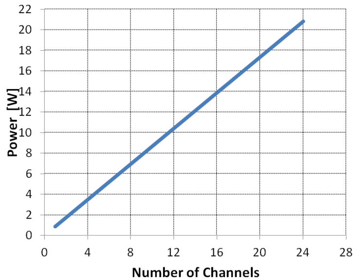
Fig 20. Puissance consommée par un frontal RF de passerelle domestique basée sur des récepteurs mono-canal
