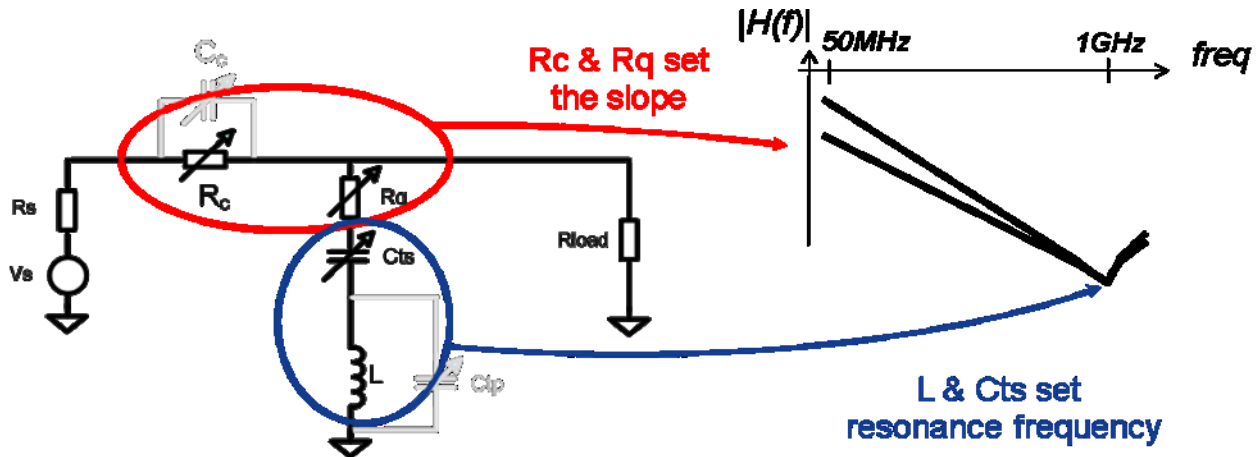
Fig 28. Egaliseur RF configuré dans un résonateur série
