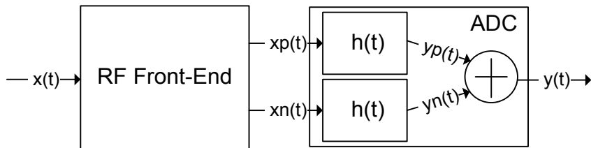
Fig 11. Interface entre le frontal RF et l'échantillonneur
