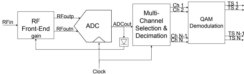
Fig 21. Récepteur à échantillonnage et numérisation directs
