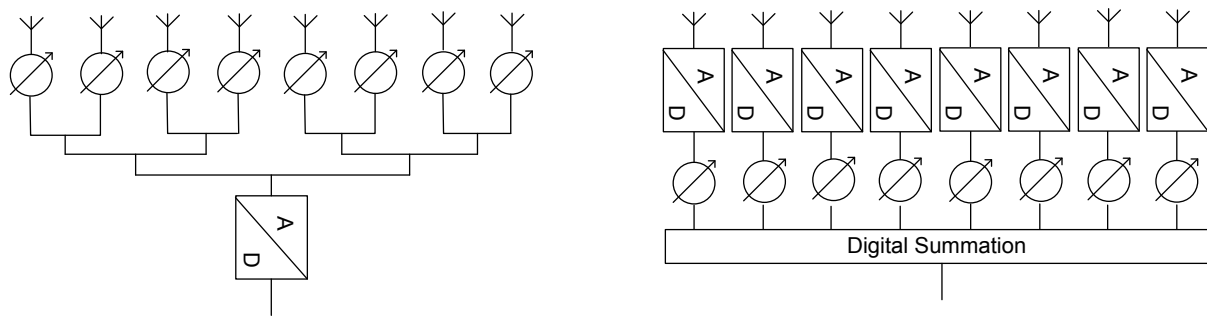
Fig 2. Gauche: Formation analogique de faisceaux. Droite: Formation numérique de faisceaux
