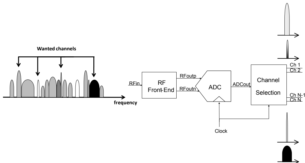
Fig 5. Récepteur à numérisation directe RF
