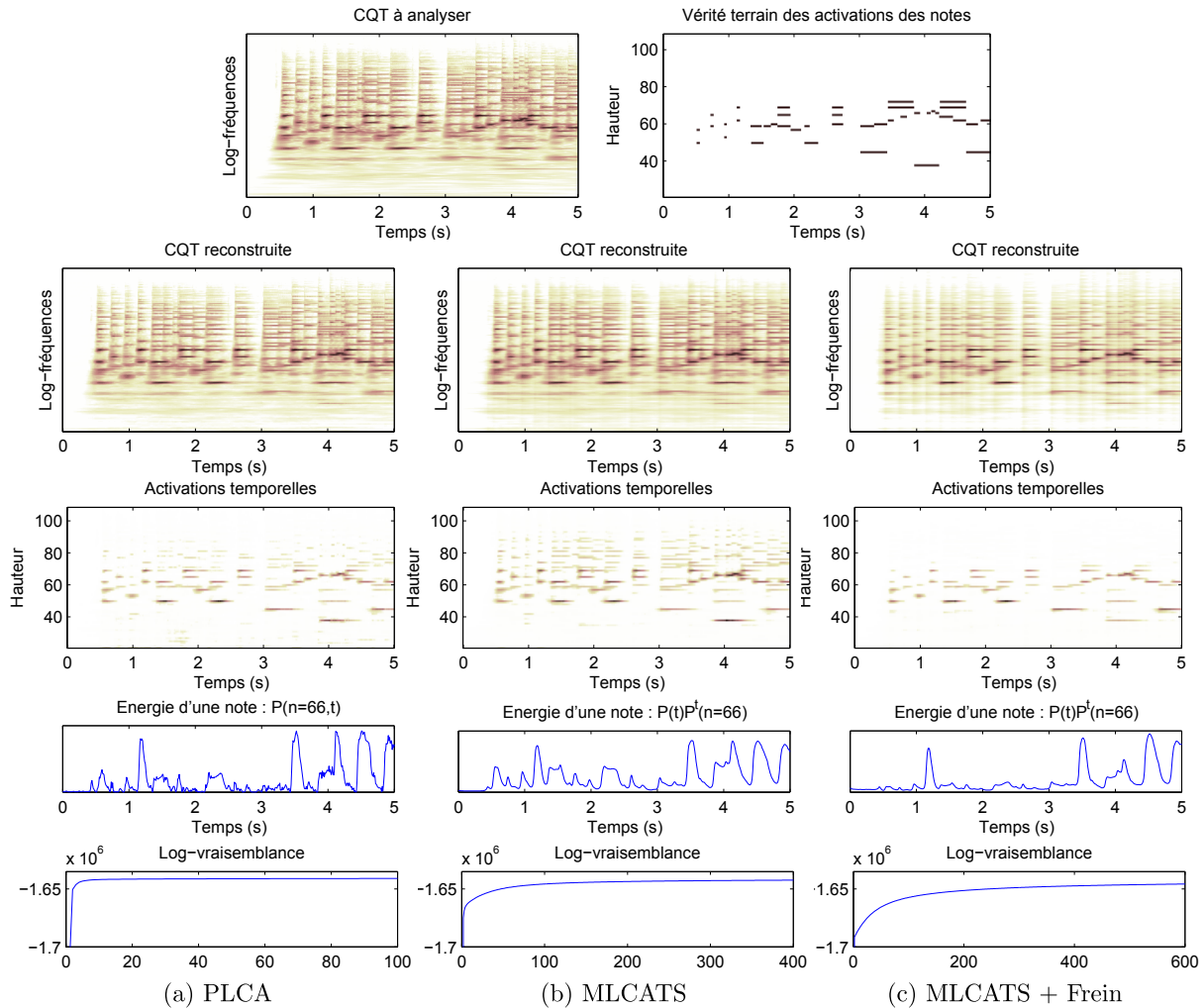
Figure 5.4 – Activations temporelles des notes obtenues avec la MLCATS et la PLCA ainsi que la log-vraisemblance au fil des itérations. Le signal d'entrée correspond à un extrait de 5 secondes de la Suite bergamasque (Menuet) de C. Debussy, joué au piano. Les activations des atomes fixes de bruit ne sont pas illustrées ici.
