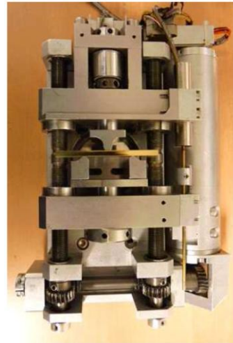
Figure I.38 – Présentation de la machine de flexion in-situ 3 points utilisée avec le MEB [8].
