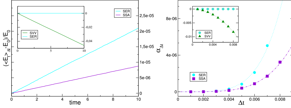
Figure 2 | Étude des propriétés de préservation d'énergie des schémas SVV, SER et SSA. Gauche: énergie moyennée sur toutes les trajectoires en fonction du temps. Droite: coefficients de dérive par rapport au temps de l'énergie moyennée sur toutes les trajectoires en fonction du pas de temps.
