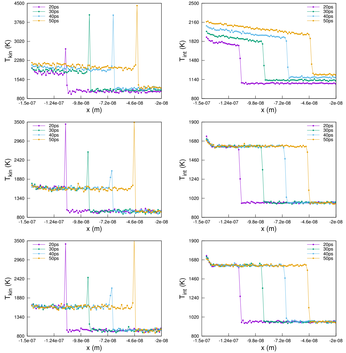
Figure 5 | Profils des températures cinétiques (gauche) et internes (droite) moyennées sur des tranches normales à la direction de propagation du choc pour un pas de temps \Delta t = 10^{-15} s. Haut : profils obtenus avec des simulations SEM. Milieu : profils obtenus avec des simulations Hybrid. Bas : profils obtenus avec des simulations SER.
