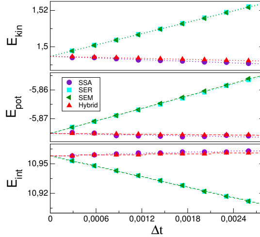
Figure 3 | Estimations numériques de biais sur les moyennes des composantes de l'énergie en fonction du pas de temps. Haut : composante cinétique de l'énergie. Milieu : composante potentielle de l'énergie. Bas : composante interne de l'énergie.
