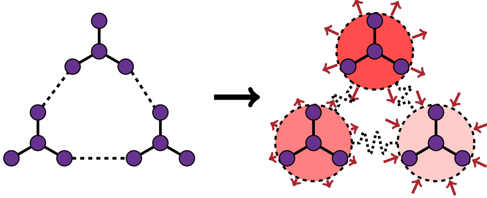
Figure 1 | Illustration du procédé de modélisation de la DPDE: chacune des trois molécules (en violet) interagissant entre elles par des forces conservatives (lignes droites: continues pour les interactions à courte portée et en pointillées pour les interactions à longue portée) est représentée par une seule macroparticule DPDE (cercles en pointillés). Chacune de ces macroparticules interagit avec les autres via des interactions conservatives, dissipatives et aléatoires: les interactions entre particules DPDE ne sont donc plus déterministes mais stochastiques. En plus de sa position et de son moment, chaque macroparticule DPDE est décrite par une variable supplémentaire qui est l'énergie interne (plus la particule est rouge, plus cette variable est grande) représentant les degrés de liberté internes de sa molécule associée. L'équilibration des degrés de liberté internes/externes est faite par des transferts d'énergie liés aux interactions de fluctuation/dissipation (flèches rouges).
