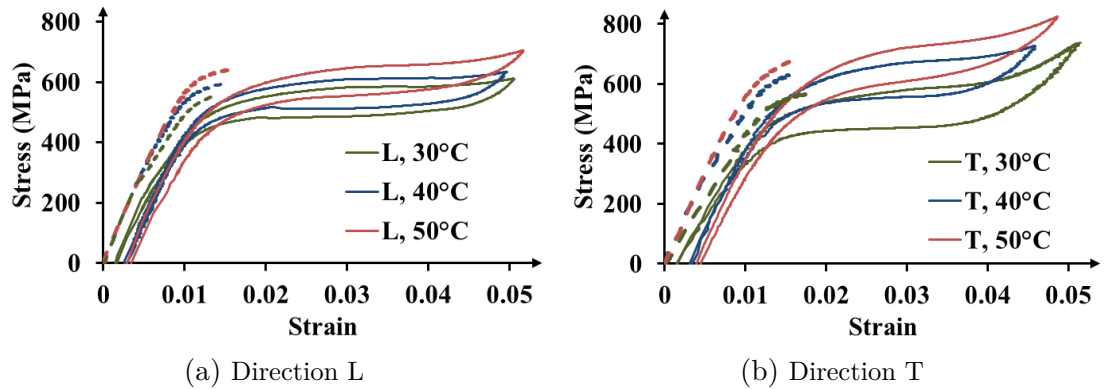
FIGURE 2.2 – Courbes contrainte-déformation pour le 1er (lignes en pointillés) et le 32ème cycle (lignes continues) pour le chargement en directions (a) 0^\circ (L) et (b) 90^\circ (T).
