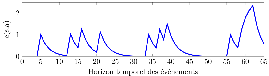
(b) Profil de la trace d'éligibilité accumulative
