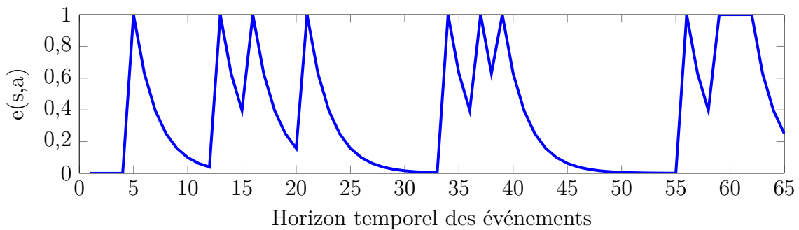
(c) Profil de la trace d'éligibilité avec réinitialisation
