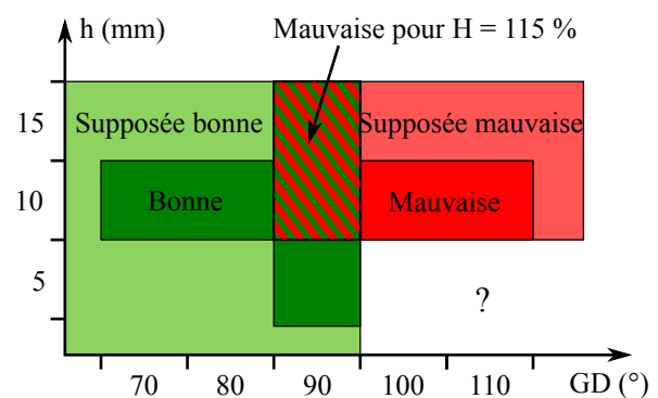
FIGURE 3.31 – Zones de bonne et de mauvaise fragmentation pour le douglas ( H = 40 et 115 \% , b = 10 mm). Les zones claires vertes et rouges sont les zones supposées de bonne et mauvaise coupes. Les points d'interrogation sont les zones non testées où l'on ne peut présumer de rien.
