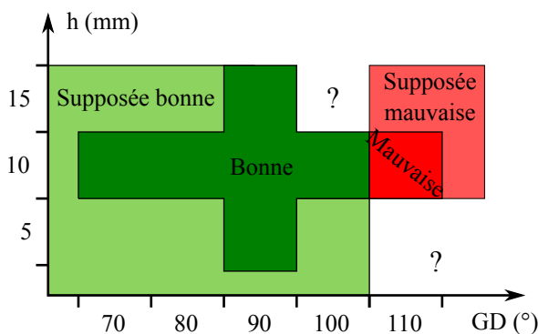
FIGURE 3.30 – Zones de bonne et de mauvaise fragmentation pour le hêtre ( H = 60 et 130 \% , b = 10 mm). Les zones claires vertes et rouges sont les zones supposées de bonne et mauvaise coupes. Les points d'interrogation sont les zones non testées où l'on ne peut présumer de rien.
