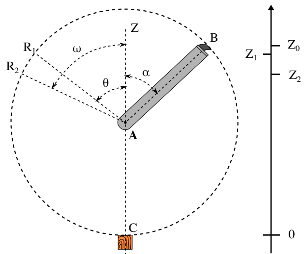
FIGURE 3.9 – Schéma de principe du pendule de Chardin [Chardin 58].
