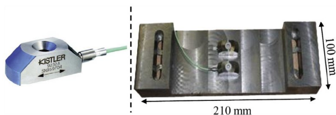
FIGURE 3.13 – Extensomètre utilisé et fixation sur l'enclume [Abdallah 14].
