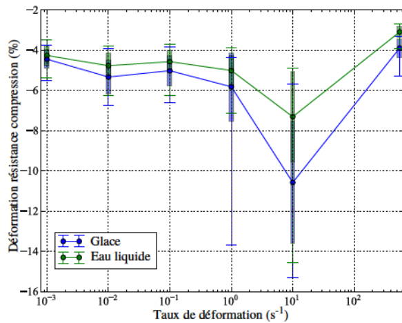
(a) Déformation résistance à la compression
