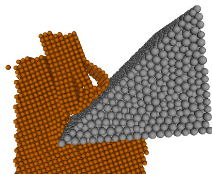
FIGURE 5.15 – Simulation de la coupe du bois dans le fil ( GD = 70^\circ ).
