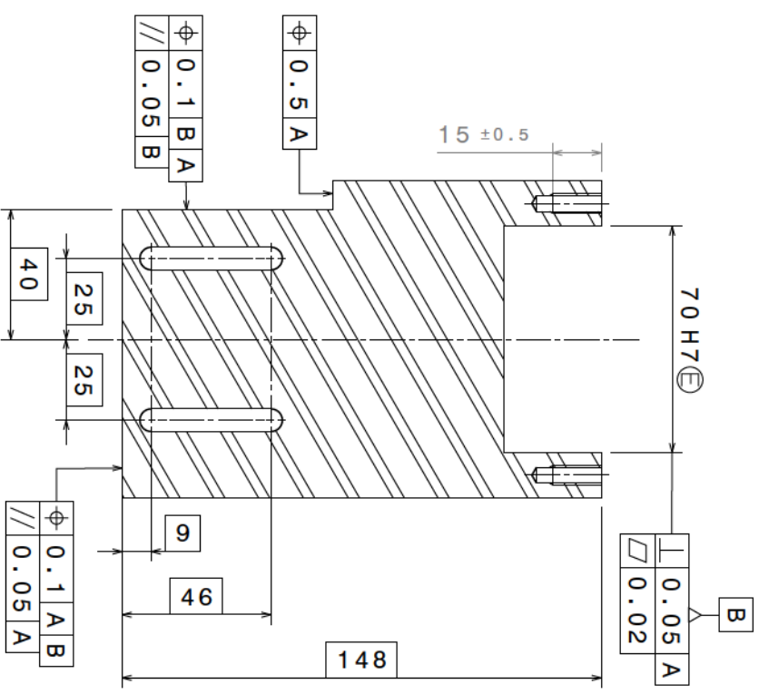
Coupe B-B
