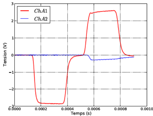
FIGURE D.3 – Tension de sortie des ponts de Wheatstone, image des déformations mesurées en fonction du temps.
