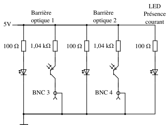
FIGURE D.12 – Schéma électrique du cablage des barrières optiques.
