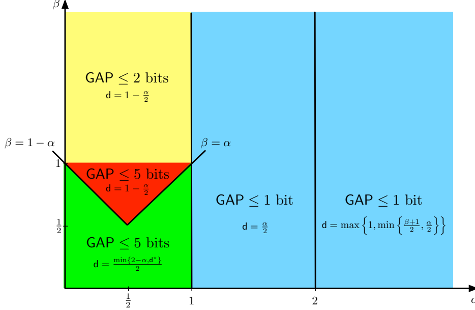
Figure 7.5: Différent régimes dépendant de valeurs \alpha et \beta , avec d^* := \max\{\alpha, 1 - \alpha\} + \max\{\alpha, 1 + \beta - \max\{\alpha, \beta\}\} .
