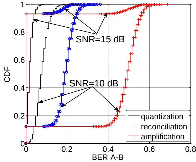
Figure 25 Le BER des clés légitimes durant les différentes étapes de la SKG
