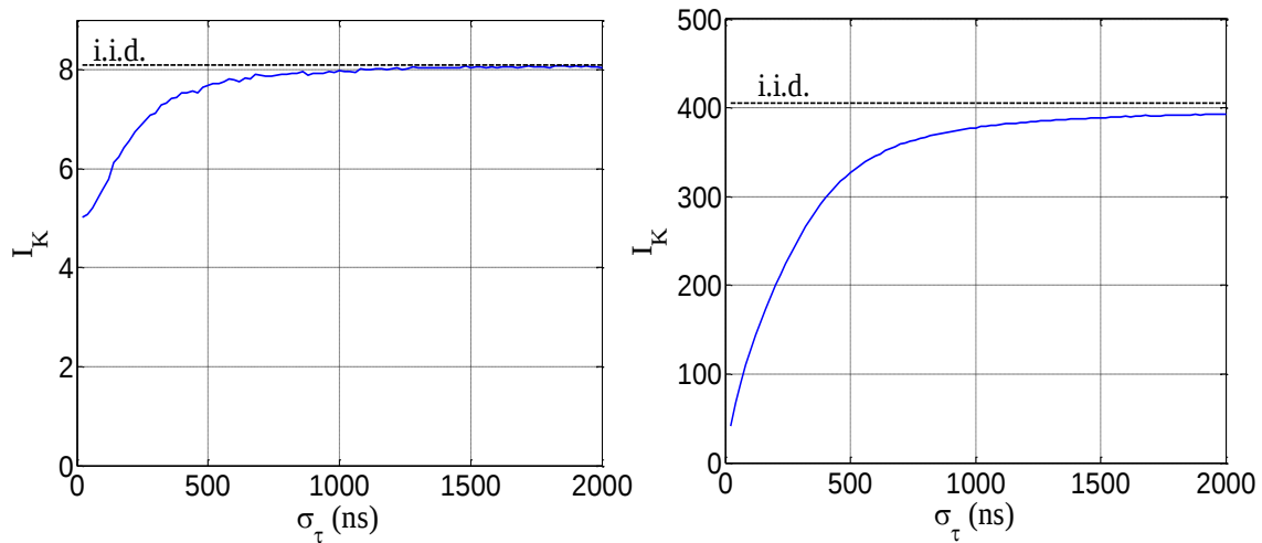
Figure 7 I_K en fonction de l'étalement temporel \sigma_\tau pour N_f = 2 (gauche) et N_f = 100 (droite)
