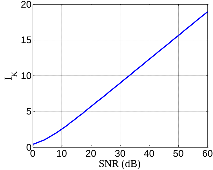
Figure 4 I_K en fonction du SNR
