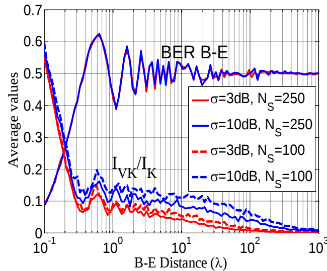
Figure 9 La vulnérabilité ( I_{VK}/I_K et BER) en fonction de la distance Bob-Eve
