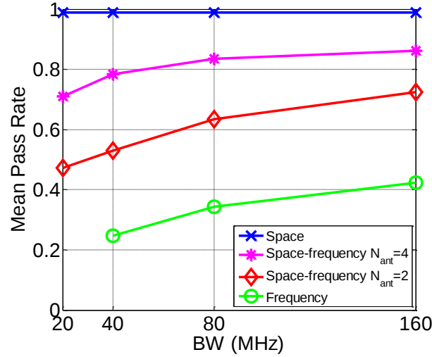
Figure 22 Comparaison de l'aléa fourni par les différents degrés de liberté
