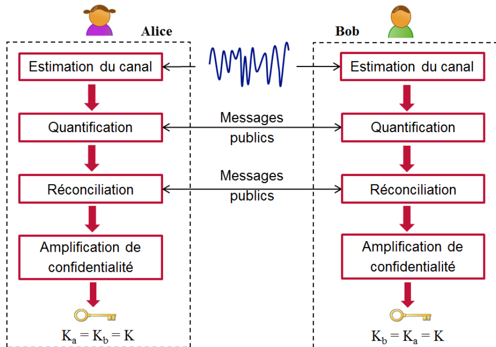
Figure 3 La stratégie complète de la SKG
