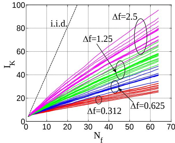
Figure 23 I_K en fonction de N_f
