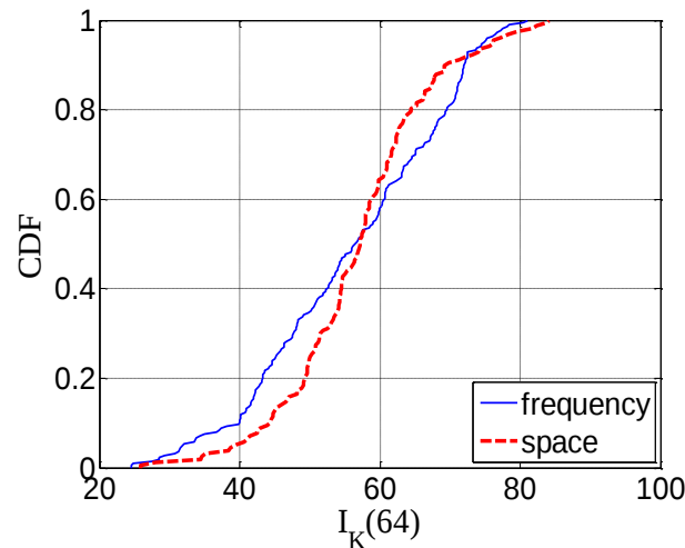
Figure 13 I_K dans les domaines spatiaux et fréquentiels
