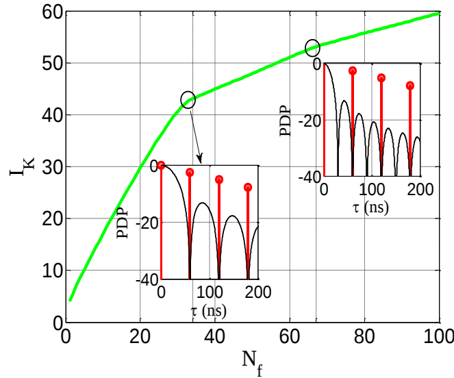
Figure 6 L'évolution de I_K en fonction du nombre de sous-porteuses
