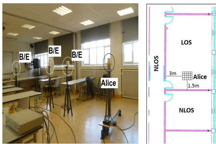
Figure 15 Mesures en salles de classe
