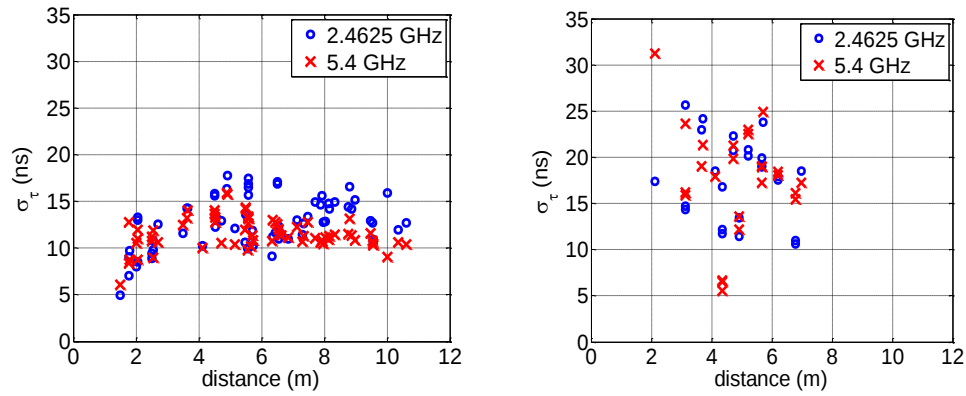
Figure 21 \sigma_\tau en fonction de la distance Alice-Bob pour LOS (gauche) et NLOS (droite)
