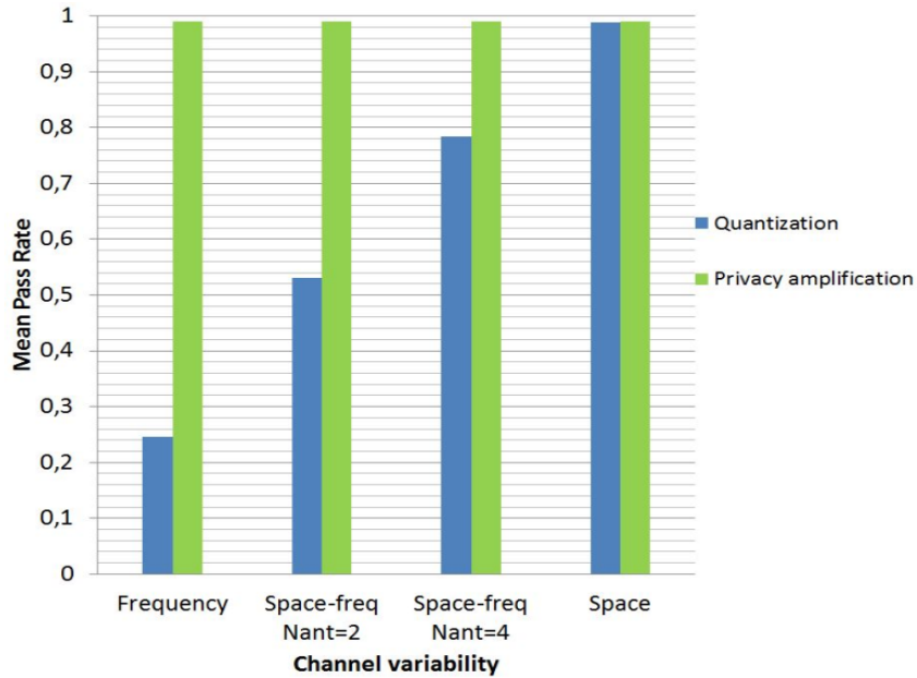
Figure 26 Le caractère aléatoire des clés durant les étapes de la SKG
