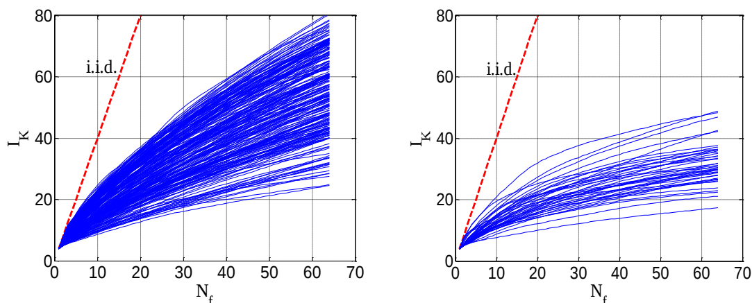
Figure 10 I_K en fonction de N_f : avec diffusion (gauche) et sans diffusion (droite)
