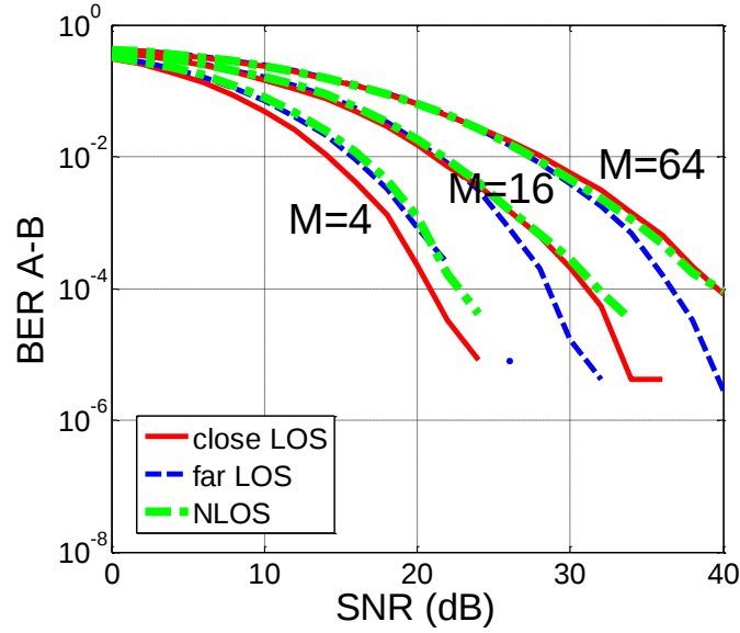
Figure 17 Le BER entre les clés d'Alice et de Bob en fonction du SNR
