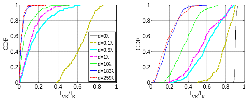
Figure 14 I_{VK}/I_K en fonction de la distance Bob-Eve et pour N_f=1 (gauche) et N_f=32 (droite)
