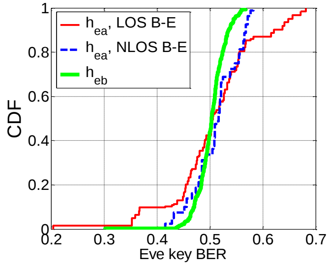
Figure 18 Taux d'erreur binaire par rapport à l'espion
