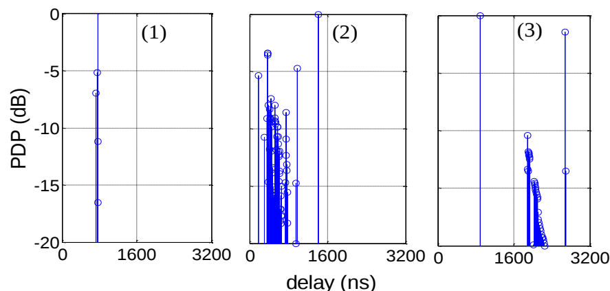
Figure 11 Des exemples de profils de puissance-délai
