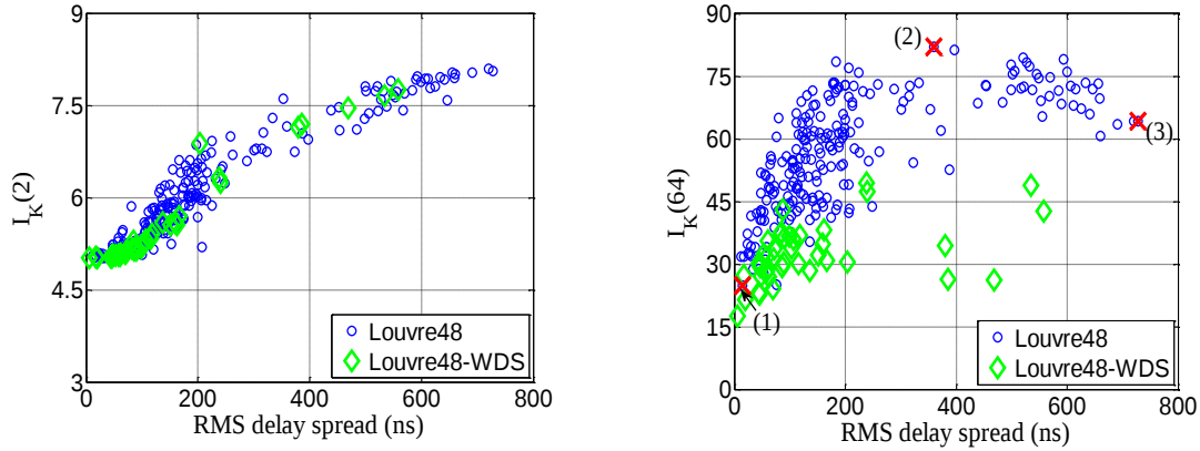
Figure 12 I_K en fonction de delay spread: N_f=2 (gauche) et N_f=64 (droite)
