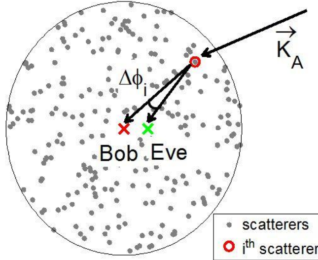
Figure 8 Modèle stochastique et géométrique
