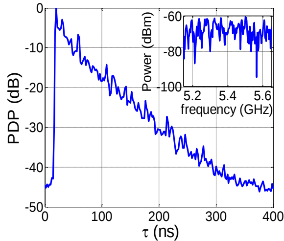
Figure 24 Un exemple de réponse impulsionnelle en environnement à l'intérieur
