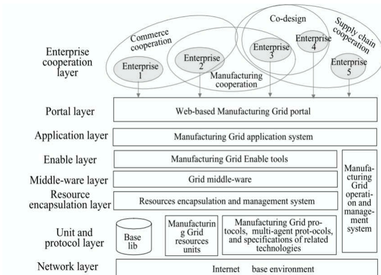
FIGURE 3.1 – L'architecture d'une MGrid selon [Fan 04]
