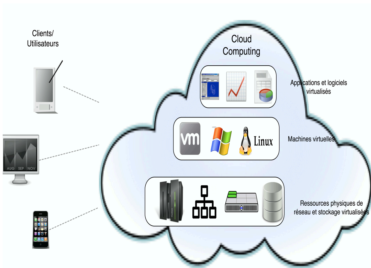
FIGURE 1.5 – Le CC et la virtualisation
