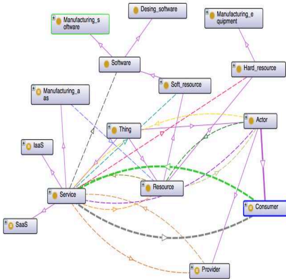
FIGURE 6.15 – Elaboration du modèle de connaissance du système étudié à partir du Modèle générique de connaissance
