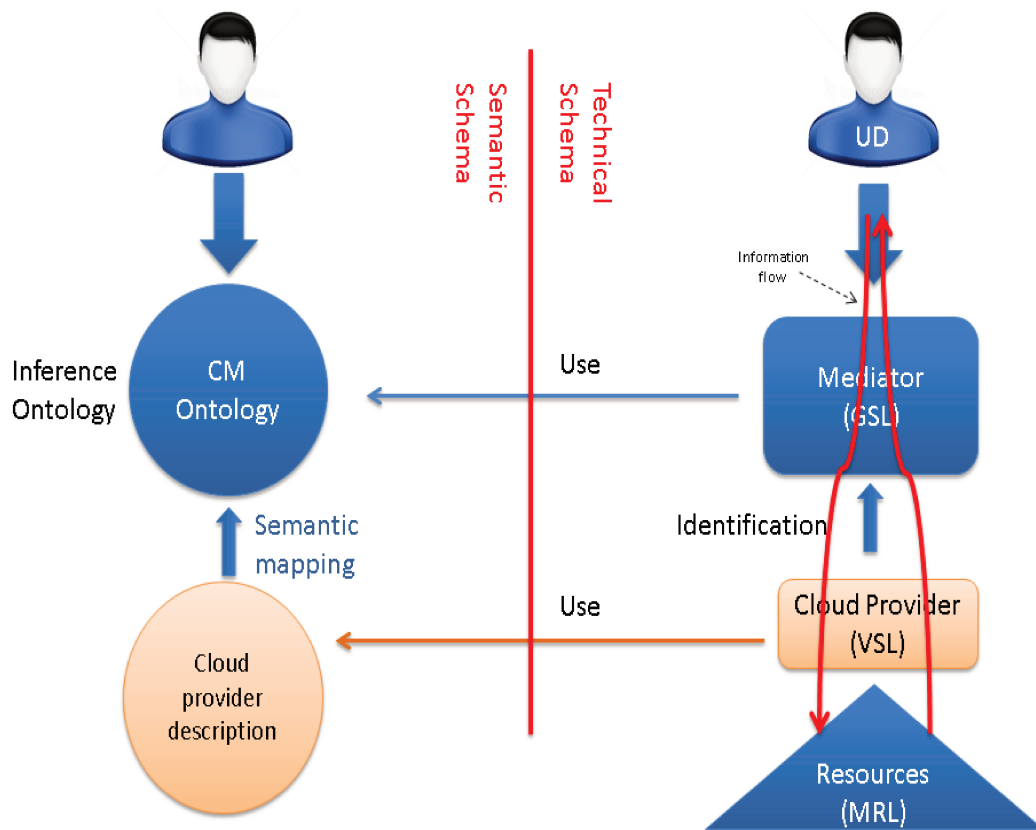
FIGURE 6.2 – Lien entre schéma sémantique et schéma technique
