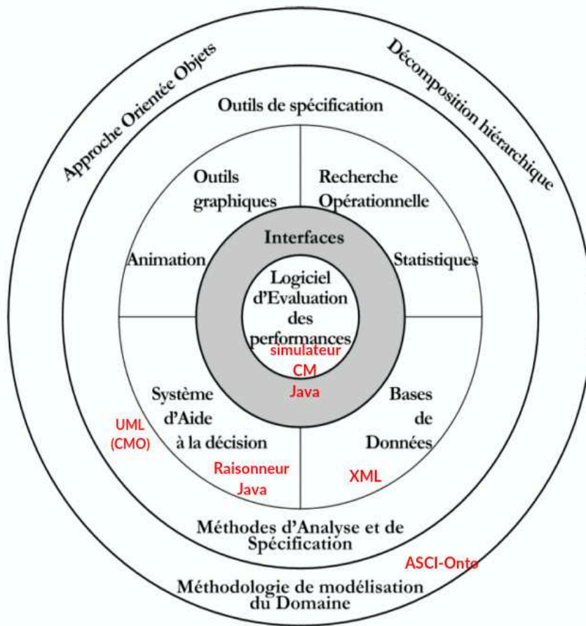
FIGURE 6.11 – Environnement logiciel ASCII-Onto
