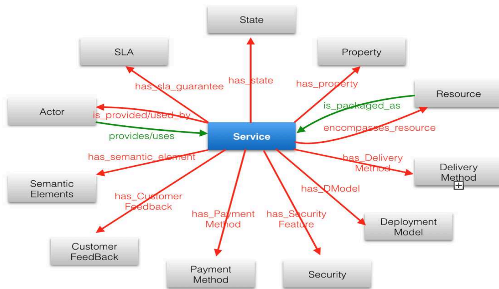
FIGURE 5.5 – Les liens sémantiques entre les concepts génériques
