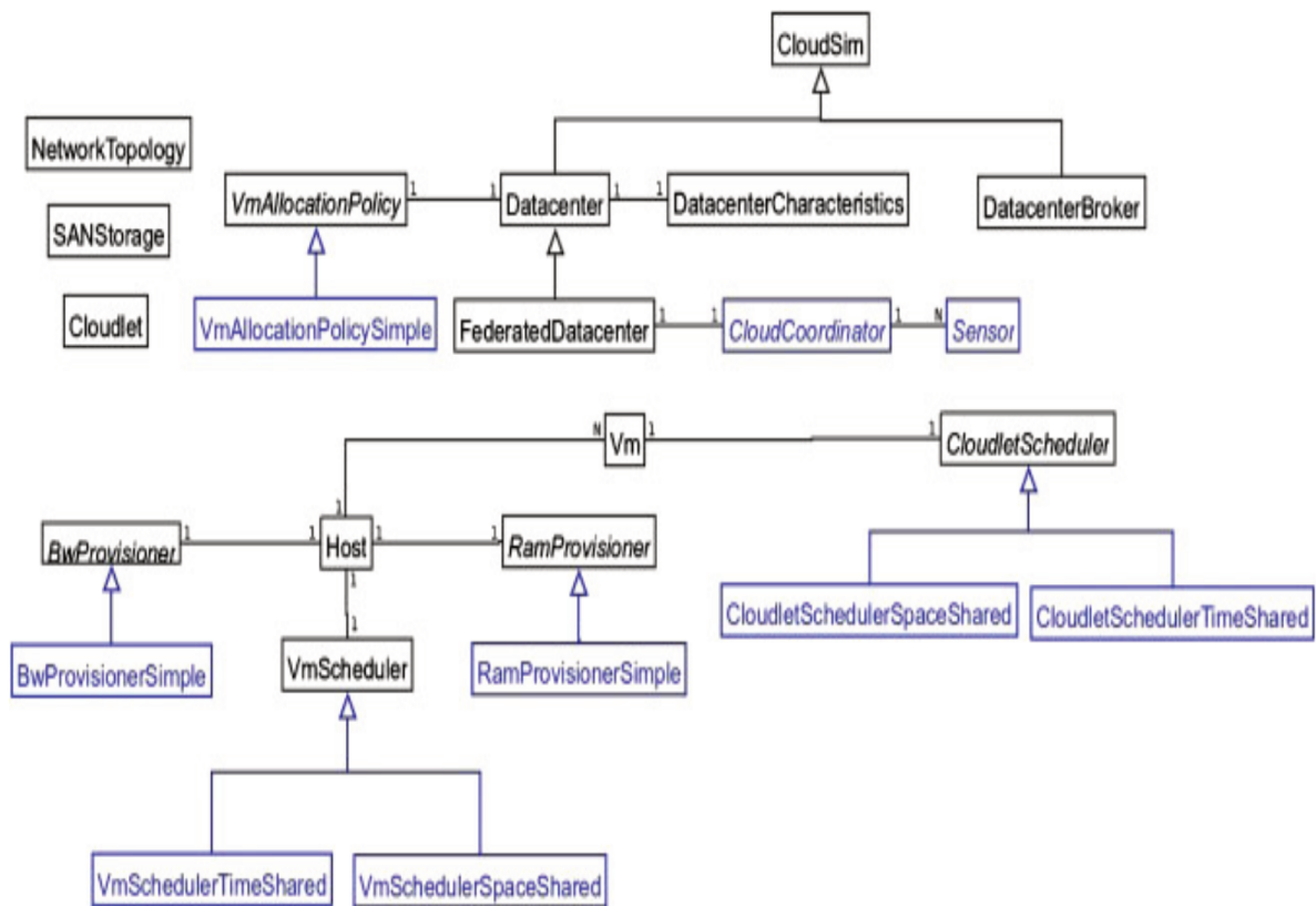
FIGURE 6.6 – Le diagramme de classe de CloudSim [Calheiros 11]
