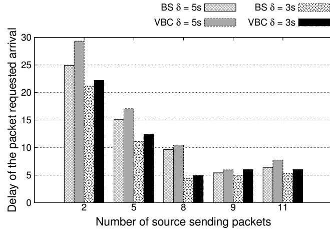
(b) Delay (FPVB)
