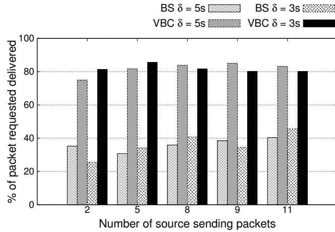
(a) Taux de paquets délivrés (EPCC)
