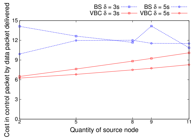
(a) Coût-bénéfice (EPCC)
