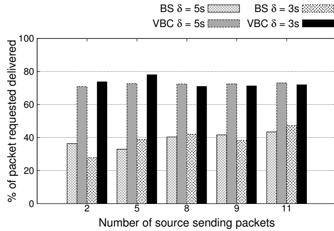
(b) Taux de paquets délivrés (FPVB)
