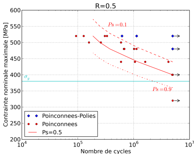
Figure III-8 : Courbes S-N relatives aux éprouvettes poinçonnées et poinçonnées-polies pour R=0,5 (Température ambiante, Modèle de Stromeyer)
