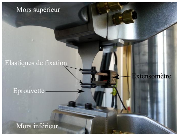
Figure II-22 : Échantillon monté sur la machine servo-hydraulique lors d'un essai d'érouissage cyclique
