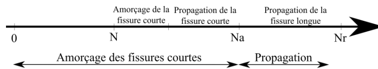
Figure I-2 : Différents stades de fissuration
