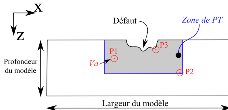
Figure IV-22 : Définition de la zone de post-traitement (ZPT) autour du défaut et du volume de moyennation V_a en chaque point P de cette zone
