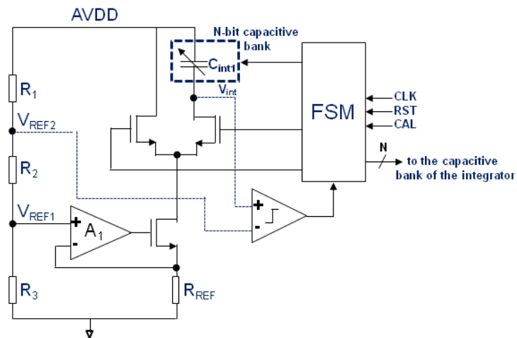
Figure 10. Circuit utilisé pour corriger les variations des constantes de temps des intégrateurs [14].
