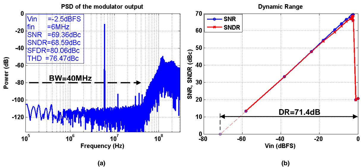
Figure 23. (a) Densité Spectrale de Puissance (DSP) en sortie du modulateur, (b) Mesure du SNR et du SNDR en fonction du signal d'entrée ( f_{\text{input}}=6\text{MHz} ).
