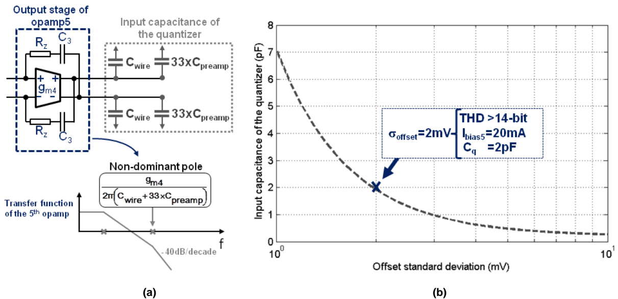
Figure 17. (a) Charge capacitive du dernier intégrateur, (b) Compromis entre l'offset et la capacité d'entrée du préamplificateur qui doit être pilotée par le filtre de boucle.
