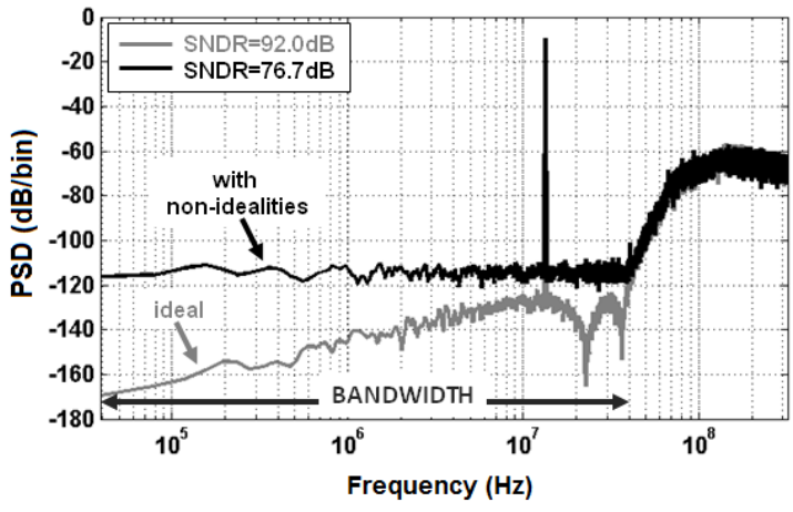
Figure 7. Densité spectrale de puissance en sortie du modulateur avec et sans les imperfections du modulateur \Delta\Sigma ( V_{in}=-1.8dBFS et f_{in}=13.32MHz ).
