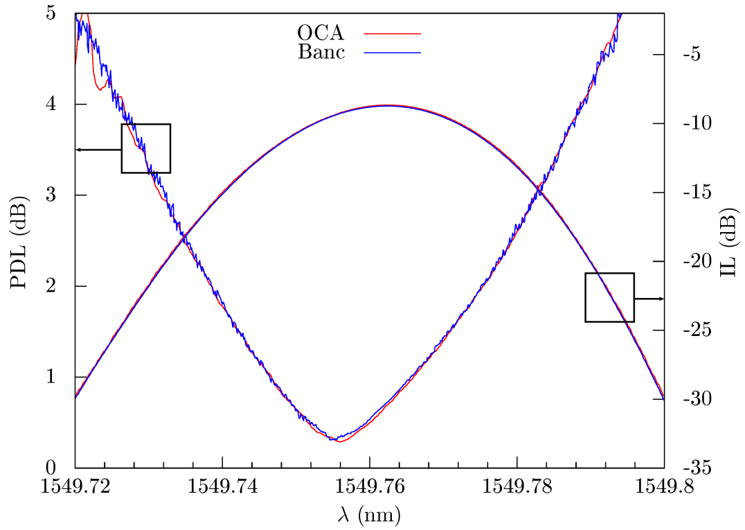
FIGURE 8.13 – PDL et IL de l'XTx-32 avec une bande passante de 30 pm.
