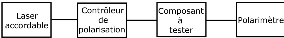
FIGURE 5.2 – Montage expérimental simplifié pour la méthode de Jones. On génère trois états prédéterminés avec le contrôleur de polarisation et la réponse du composant à tester est mesurée à l'aide d'un polarimètre.
