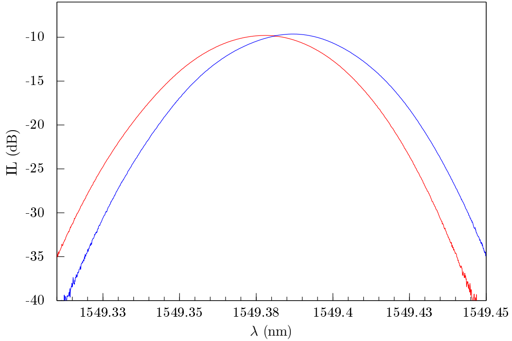
FIGURE 8.11 – Sous-filtres propres de l’XTx-50 n° 2 avec une bande passante de 45 pm. On constate un décalage en longueur d’onde centrale encore plus prononcé que dans la cas de l’XTx-50 n° 1.
