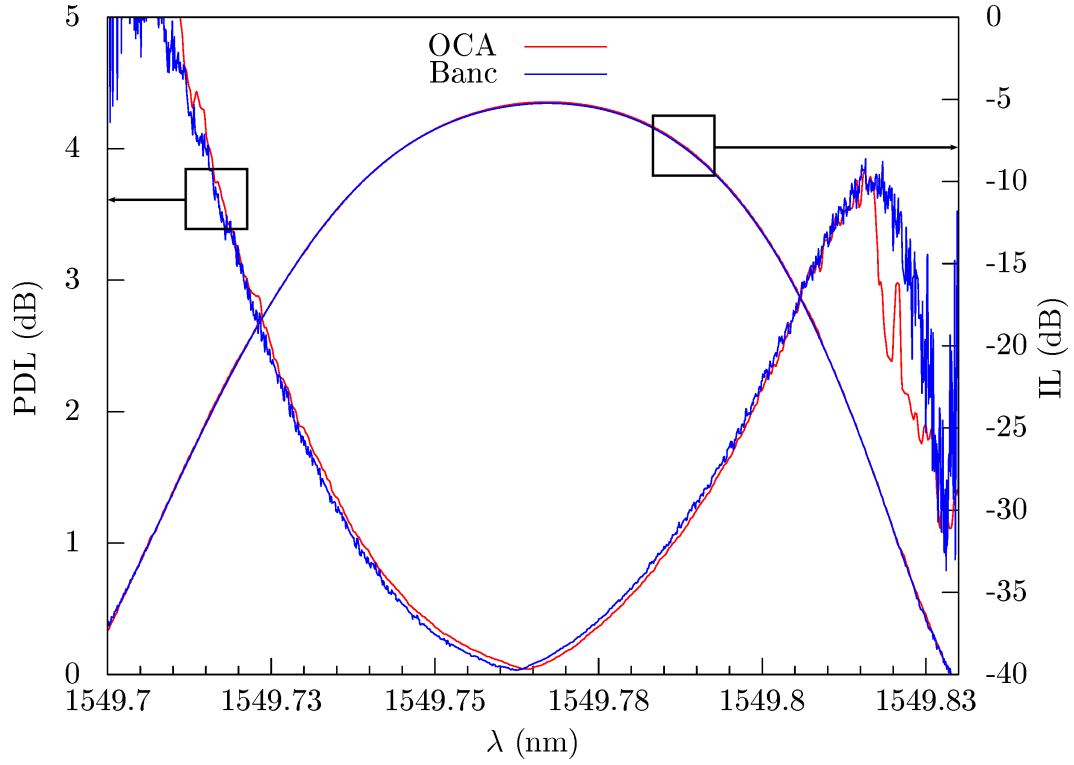
FIGURE 8.9 – PDL et IL de l'XTx-32 avec une bande passante de 45 pm.
