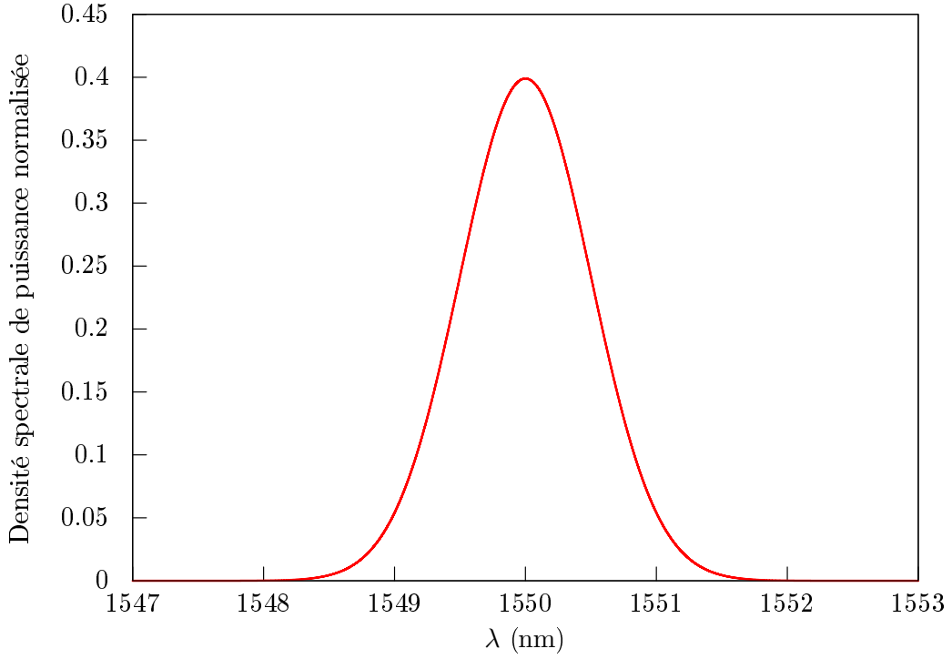
FIGURE 2.3 – Un paquet d'onde gaussien est une superposition d'OPPM dont les poids relatifs sont répartis selon une loi normale.
