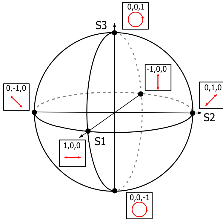
FIGURE 3.8 – Localisation des états de Stokes canoniques sur la sphère de Poincaré.
