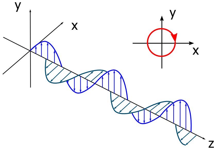
FIGURE 3.5 – Dans le cas d’une polarisation circulaire, le champ possède deux composantes selon les axes x et y de même amplitude et en quadrature de phase. La trajectoire décrite par le vecteur au cours de sa propagation est donc circulaire.
