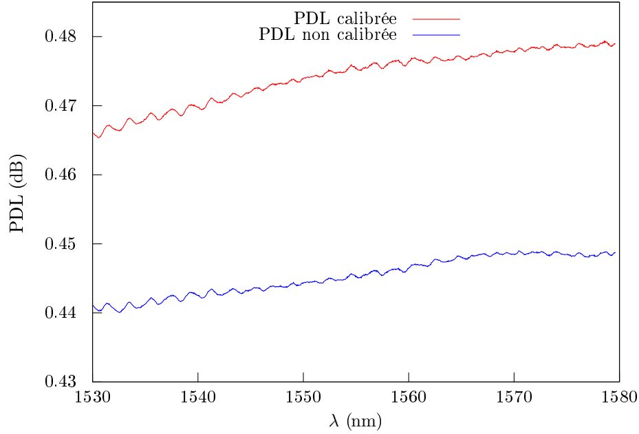
FIGURE 7.3 – Étalon à 0,5 dB. Comparaison entre la PDL calibrée et non calibrée. La PDL non calibrée correspond à la pseudo-PDL en présence du DUT, c'est à dire qu'elle intègre le déséquilibre en PDL des voies de mesure en plus de la PDL vraie du DUT. Ici, la PDL non calibrée tend à sous-estimer la PDL vraie de quelques centièmes de dB.
