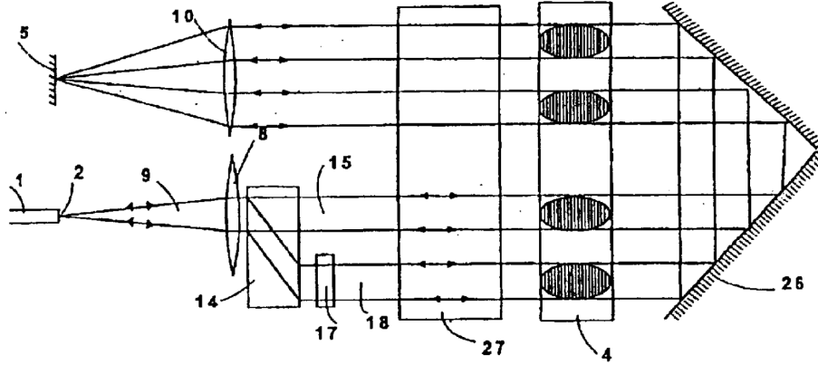
FIGURE 8.1 – US Patent 6,832,022 [33]. Trajet optique dans un filtre XTx. Le faisceau incident est séparé en ses deux composantes orthogonales à l'aide d'un bloc de calcite (14). Elles voient donc un chemin optique physiquement distinct. Une lame à retard \lambda/2 (17) permet d'obtenir finalement deux polarisations identiques de manière à ce que les deux faisceaux subissent les mêmes effets sur le réseau de diffraction (4).
