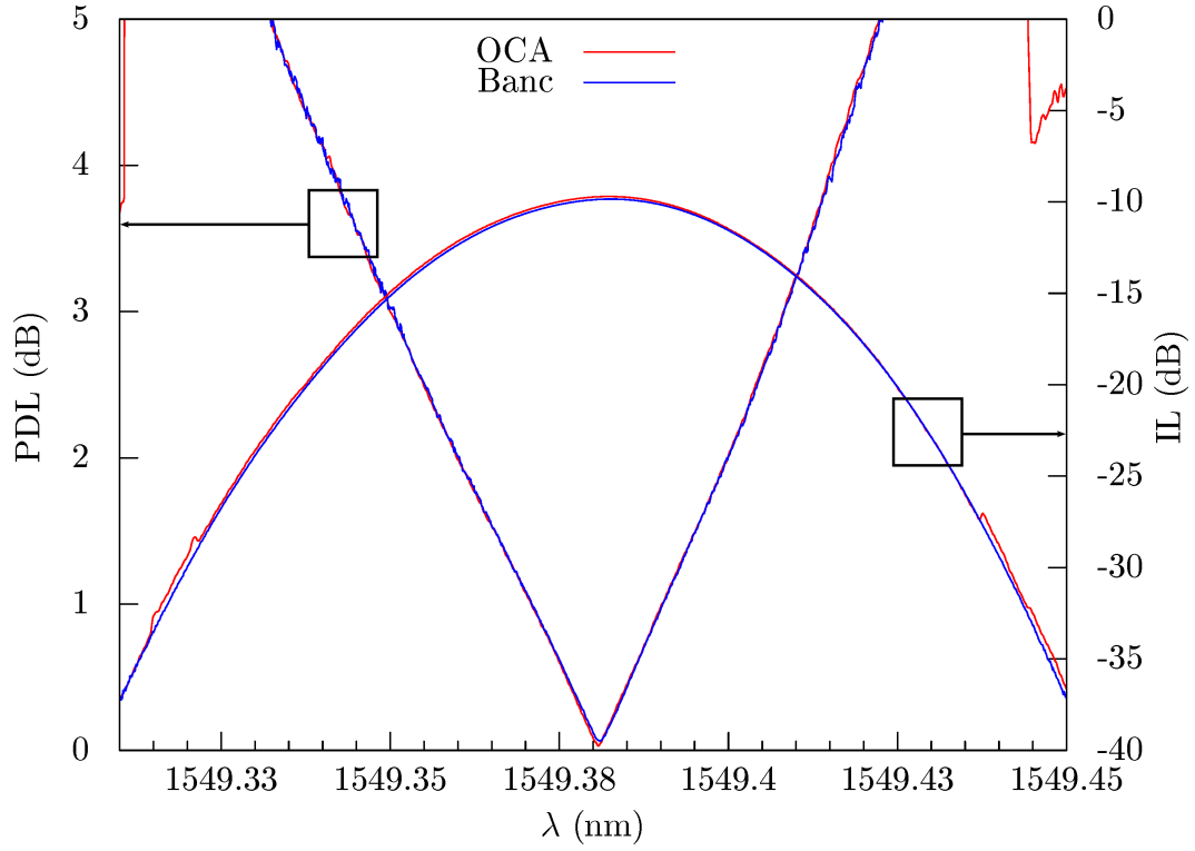
FIGURE 8.8 – PDL et IL de l'XTx-50 n° 2 avec une bande passante de 45 pm.
