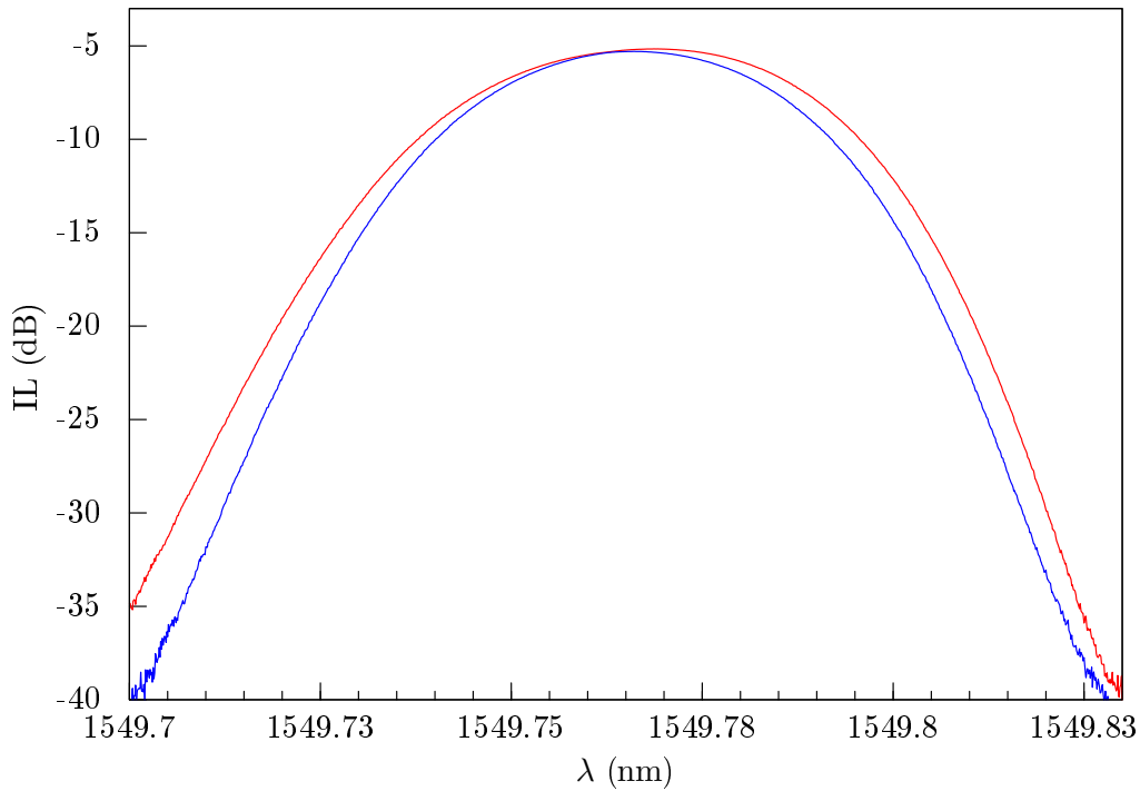
FIGURE 8.12 – Sous-filtres propres de l'XTx-32 pour une largeur de 45 pm. Cette fois, on a affaire à un écart en bande passante entre les deux sous-filtres.
