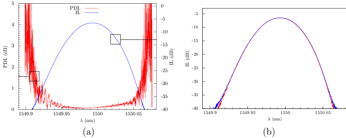
FIGURE 8.18 – (a) PDL et IL de l'XTx wide avec une bande passante de 48 pm. La PDL conserve une valeur inférieure à quelques dixièmes de dB sur l'intégralité de la bande passante. (b) Filtres propres de l'XTx wide avec une bande passante de 48 pm. Visuellement, les sous-filtres propres semblent superposés.
