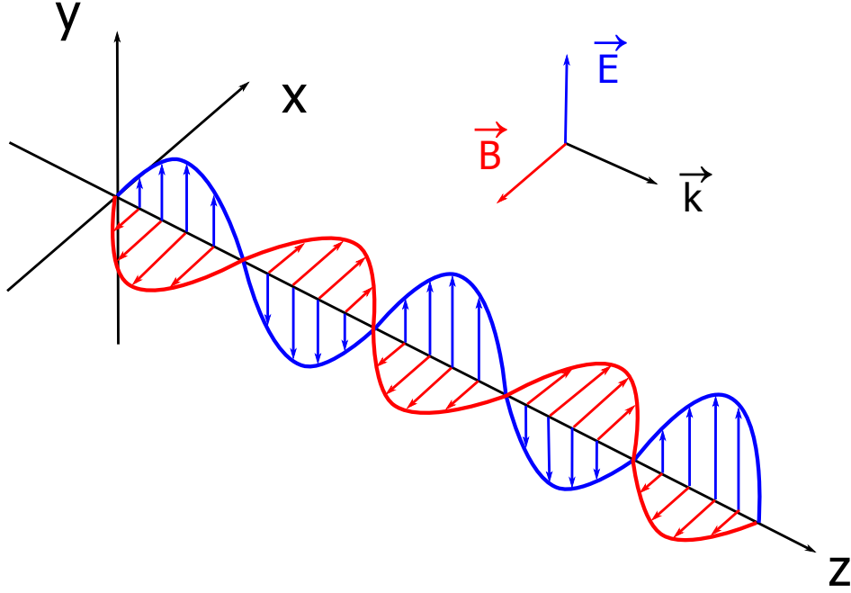
FIGURE 2.1 – Propagation du champ électromagnétique dans un milieu diélectrique linéaire, homogène et isotrope. Le champ électrique \vec{E} et le champ magnétique \vec{B} sont contenus dans le plan transverse à la direction de propagation. \vec{k} , le vecteur d'onde, \vec{E} et \vec{B} forment un trièdre direct.
