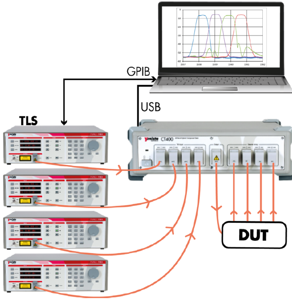
FIGURE 9.1 – Configuration typique de fonctionnement du CT400.
