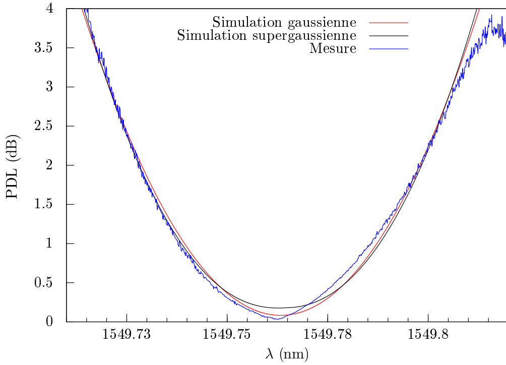
FIGURE 8.17 – Comparaison entre la PDL simulée et la PDL mesurée pour l'XTx-32. Le modèle retranscrit plutôt bien le profil mesuré avec un petit bémol proche du minimum.
