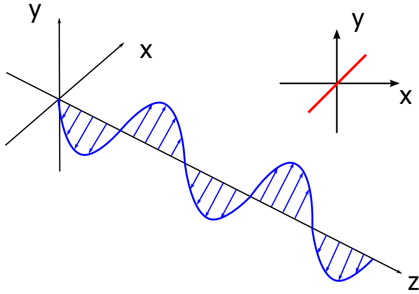
FIGURE 3.4 – Dans le cas d’une polarisation diagonale, le champ possède deux composantes selon les axes x et y de même amplitude et en accord de phase. La trajectoire décrite par le vecteur au cours de sa propagation est donc rectiligne avec un angle de 45^\circ par rapport à l’axe x .
