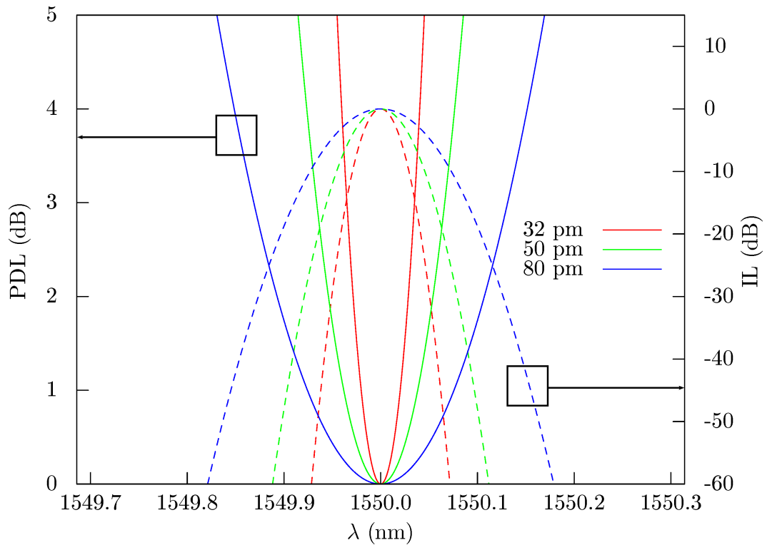
FIGURE 8.6 – PDL simulées pour 3 largeurs de filtre en considérant un écart en bande passante des sous-filtres propres de 1 pm. Une nouvelle fois, la croissance de la PDL est d'autant plus rapide que le filtre est étroit.
