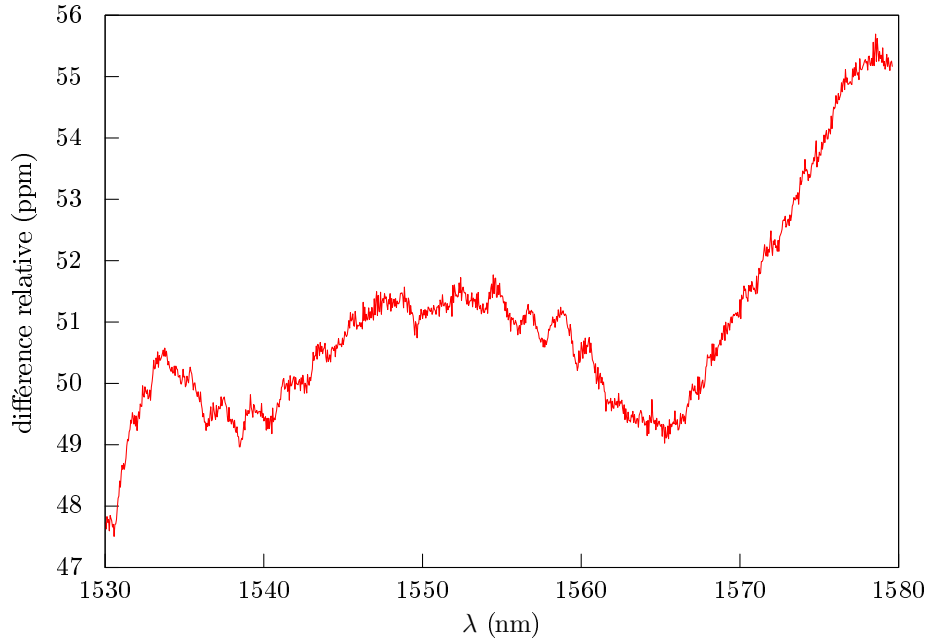
FIGURE 7.5 – Étalon à 0,5 dB. Différence relative entre la PDL calculée dans le cas matriciel et le cas vectoriel. L'écart est de l'ordre de la cinquantaine de ppm.
