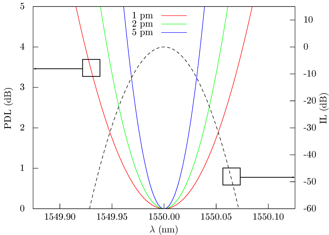
FIGURE 8.5 – PDL simulées pour différents écarts en bande passante des sous-filtres propres dans le cas d'un filtre d'une largeur de 32 pm. Encore une fois, plus l'écart est important, plus la PDL croît rapidement autour du minimum.
