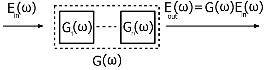
FIGURE 2.5 – Modélisation de l'action d'un composant linéaire sur une composante scalaire du champ électrique. La fonction de transfert G(\omega) du système est le produit des fonctions de transfert des parties qui le composent.
