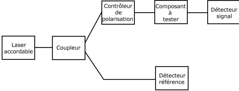
FIGURE 6.1 – Montage expérimental simplifié pour la méthode alternative de Mueller. Le détecteur de référence ne voit plus les états générés par le contrôleur de polarisation.
