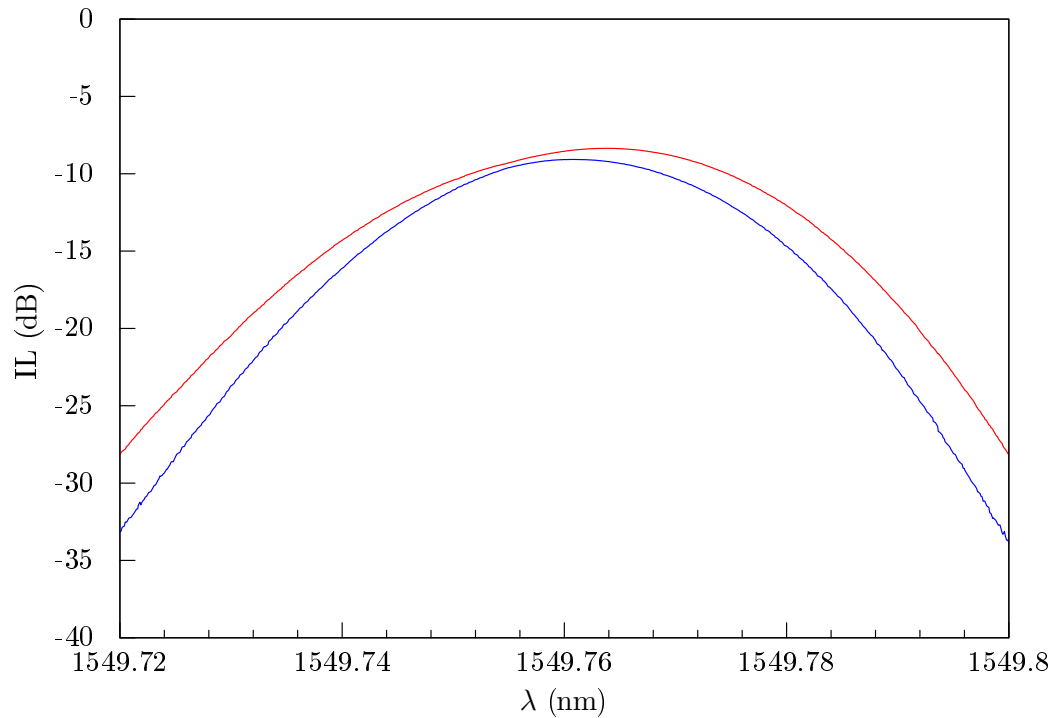
FIGURE 8.14 – Sous-filtres propres de l'XTx-32 pour une largeur de 30 pm. L'écart en bande passante apparaît sans ambiguïté.
