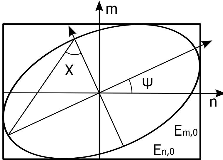
FIGURE 3.1 – L'ellipse de polarisation est la représentation géométrique de la trajectoire décrite par le champ électrique au cours de sa propagation.
