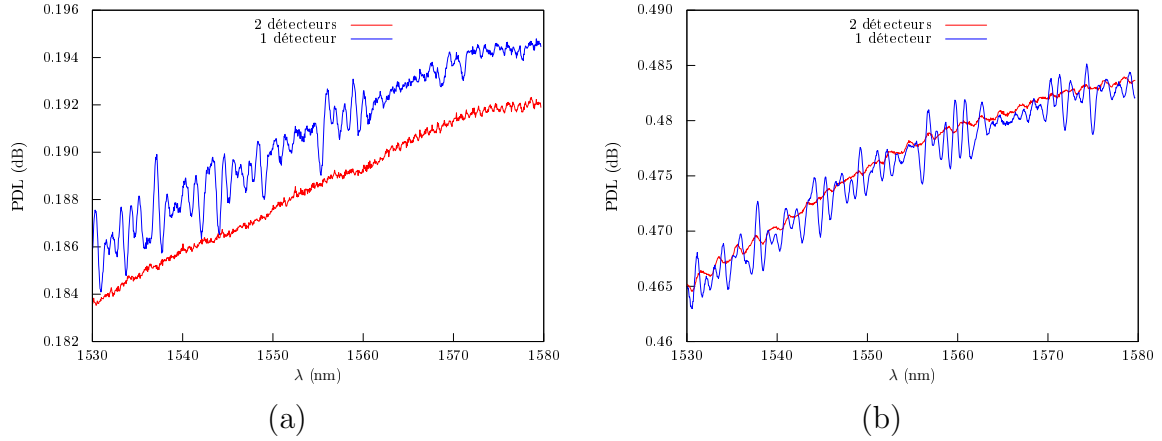
FIGURE 7.10 – PDL obtenue avec le protocole à 1 détecteur. (a) Étalon à 0,2 dB. (b) Étalon à 0,5 dB. Le bruit de la mesure est significativement augmenté quand on utilise qu’un seul détecteur. On observe aussi un léger biais respectivement de 0,02 dB et 0,01 dB dans le cas de l’étalon à 0,2 dB et 0,5 dB.
