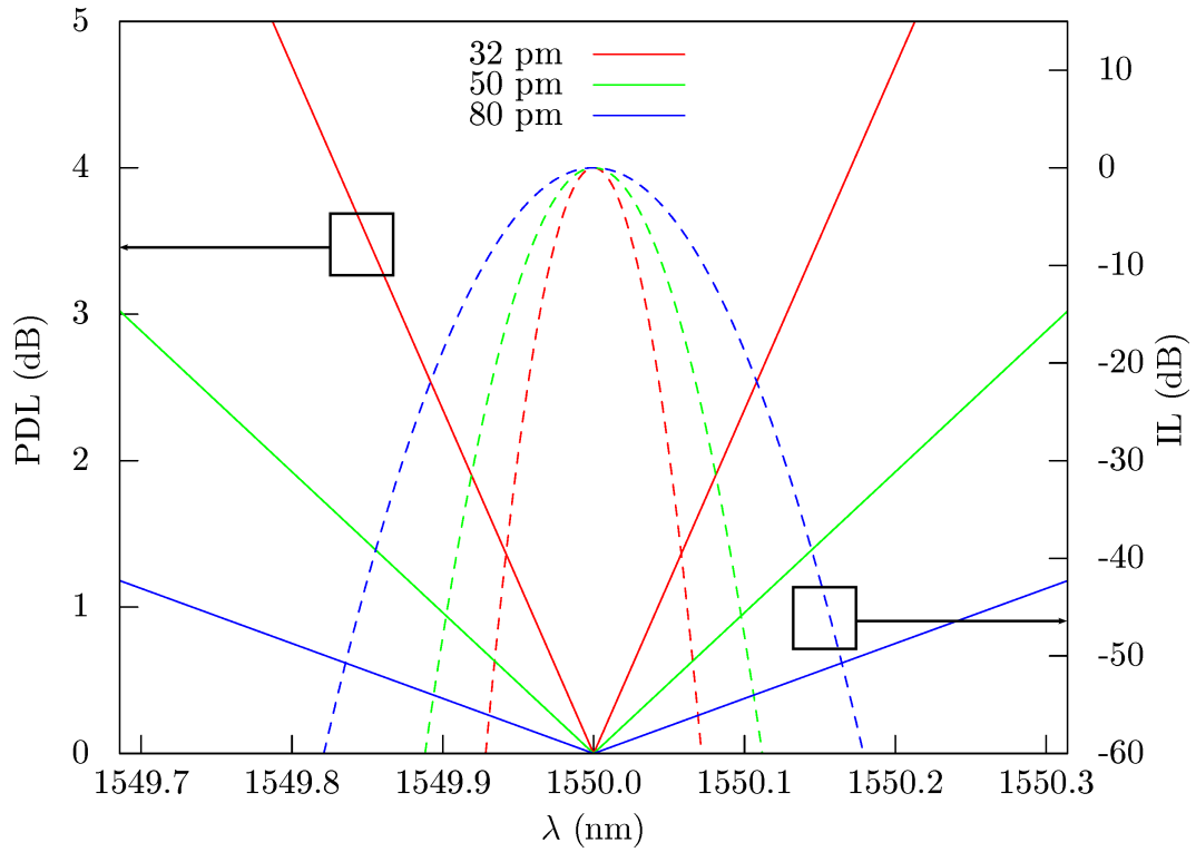
FIGURE 8.4 – PDL simulées pour 3 largeurs de filtre en considérant un décalage de la longueur d'onde centrale des sous-filtres propres de 1 pm. La croissance de la PDL est d'autant plus rapide que le filtre est étroit.
