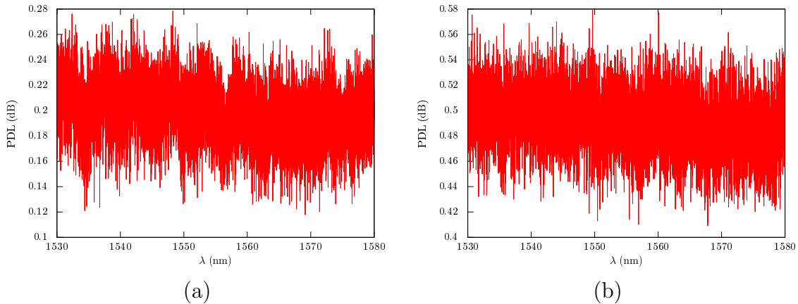
FIGURE 9.2 – (a) Mesure de la référence de PDL à 0,2 dB avec le CT400 PDL. (b) Mesure de la référence de PDL à 0,5 dB avec le CT400 PDL. Par rapport au banc de mesure, le bruit est significativement augmenté, mais la valeur moyenne du résultat reste très proche de la valeur vraie.
