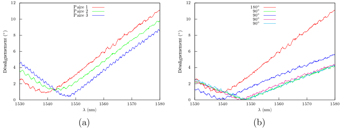
FIGURE 7.17 – (a) Désalignement angulaire des 3 paires d'états à 180^\circ générées par le contrôleur de polarisation. (b) Étant donné un état, désalignement angulaire relativement aux 5 autres. Le comportement est à chaque fois similaire : l'angle attendu n'est vérifié que pour une plage très restreinte de longueurs d'onde et l'erreur angulaire croît linéairement quand on s'en éloigne. On peut remarquer que le point de fonctionnement optimal est différent pour chaque paire considérée.
