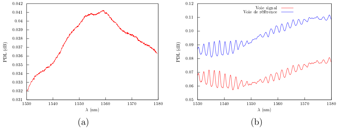
FIGURE 7.1 – Étalon à 0,5 dB. (a) Pseudo-PDL obtenue lors de la calibration. Elle correspond à la norme d'un vecteur fictif qui serait la différence des vecteurs de PDL associés à chacune des voies de mesure. On constate qu'elle est non nulle et présente des variations de l'ordre du centième de dB sur la bande d'analyse. (b) PDL totale des deux voies mesurées à la calibration. On peut remarquer des fluctuations sinusoïdales fortement corrélées entre les deux voies, ce qui tend à nous indiquer qu'elles proviennent de la voie commune. En pratique, elles sont issues du contrôleur de polarisation.
