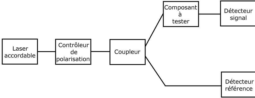
FIGURE 5.3 – Montage expérimental simplifié de la méthode de Mueller. On génère quatre ou six états prédéterminés avec le contrôleur de polarisation et la puissance transmise est mesurée à l’aide d’un puissance-mètre. Un détecteur de référence permet de s’affranchir des fluctuations de puissance du laser.
