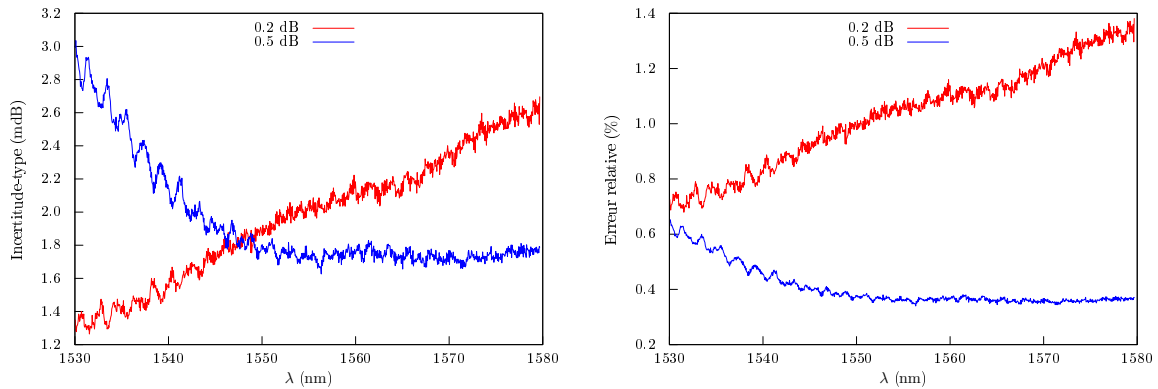
FIGURE 7.16 – Dispersion de la mesure dans des conditions de reproductibilité pour le protocole à 6 états. Contrairement au cas du protocole à 4 états, on ne détecte pas vraiment de tendance pour l’incertitude-type. Elle ne paraît pas non plus corrélée à la PDL mesurée.
