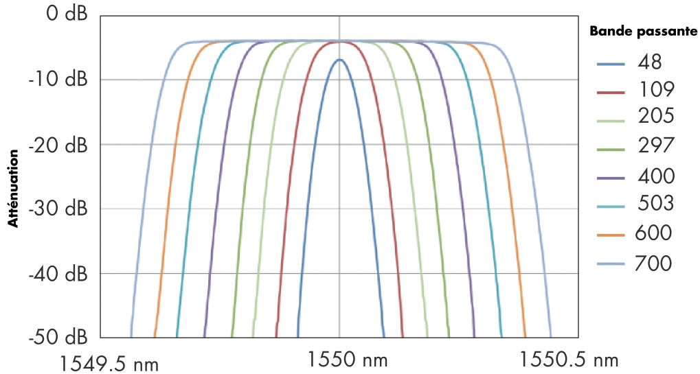
FIGURE 1.3 – Profil en transmission d'un filtre XT x pour différentes bandes passantes
