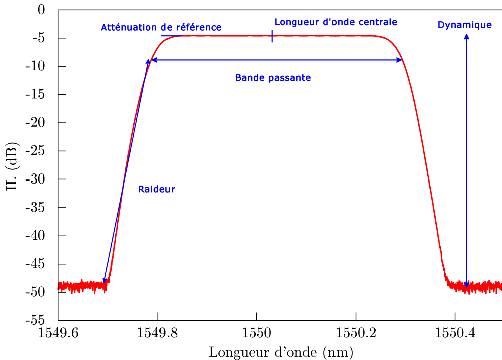
FIGURE 1.1 – Profil spectral d'un filtre optique passe-bande.
