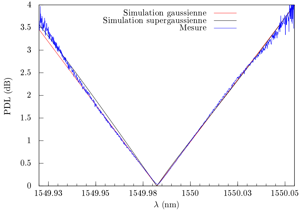
FIGURE 8.15 – Comparaison entre la PDL simulée et la PDL mesurée pour l'XTx-50 n° 1. Les simulations approximent correctement les résultats de la mesure.
