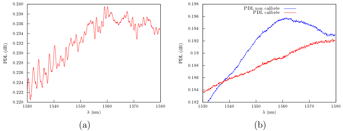
FIGURE 7.7 – Étalon à 0,2 dB. (a) PDL totale de la voie signal en présence du DUT. On retrouve une PDL proche de la PDL attendue. (b) Comparaison entre la PDL calibrée et non calibrée.
