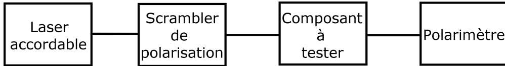
FIGURE 5.1 – Montage expérimental simplifié pour la méthode de balayage en polarisation. La PDL est déduite de la variation de puissance relevée sur le puissancemètre quand le scrambler balaie la sphère de Poincaré. En faisant varier la longueur d'onde du laser accordable, on caractérise spectralement le composant à tester.
