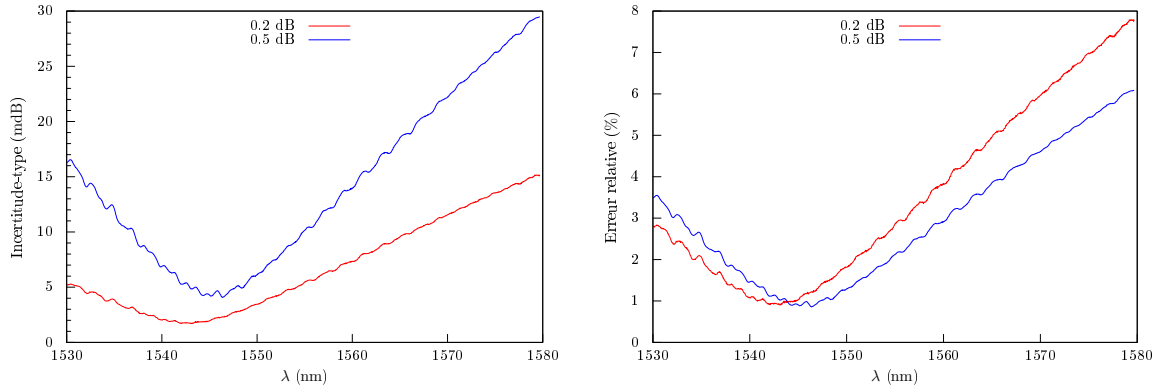
FIGURE 7.15 – Dispersion de la mesure dans des conditions de reproductibilité pour le protocole à 4 états. On observe très nettement la symétrie de l’incertitude-type de part et d’autre d’un minimum. On constate aussi que l’erreur relative est très proche pour les deux étalons à 0,2 dB et à 0,5 dB.
