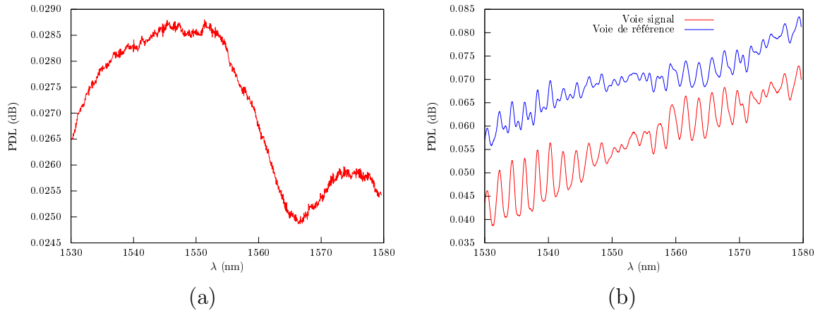
FIGURE 7.6 – Étalon à 0,2 dB. (a) Pseudo-PDL obtenue lors de la calibration. On obtient un profil différent par rapport à celui trouvé dans le cas de l'étalon à 0,5 dB. (b) PDL totale des deux voies mesurées à la calibration. On retrouve des fluctuations sinusoïdales similaires mais pas strictement identiques à celles mesurées dans cas de l'étalon à 0,5 dB.
