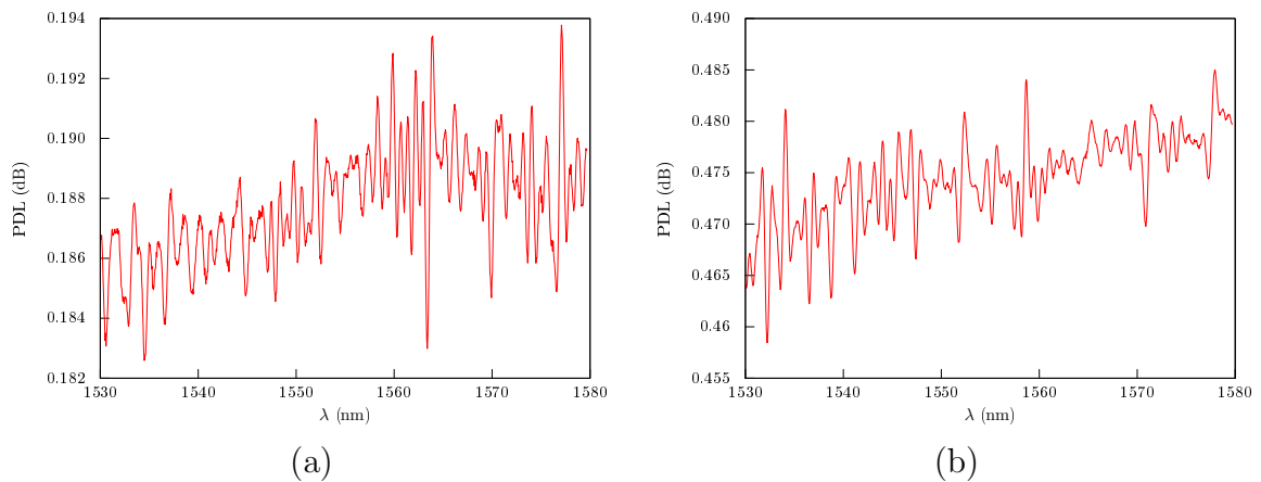
FIGURE 7.11 – PDL obtenue avec le protocole alternatif. (a) Étalon à 0,2 dB. (b) Étalon à 0,5 dB. On observe un comportement similaire au cas à 1 détecteur. On retrouve en moyenne le bon résultat, mais avec une très mauvaise reproductibilité
