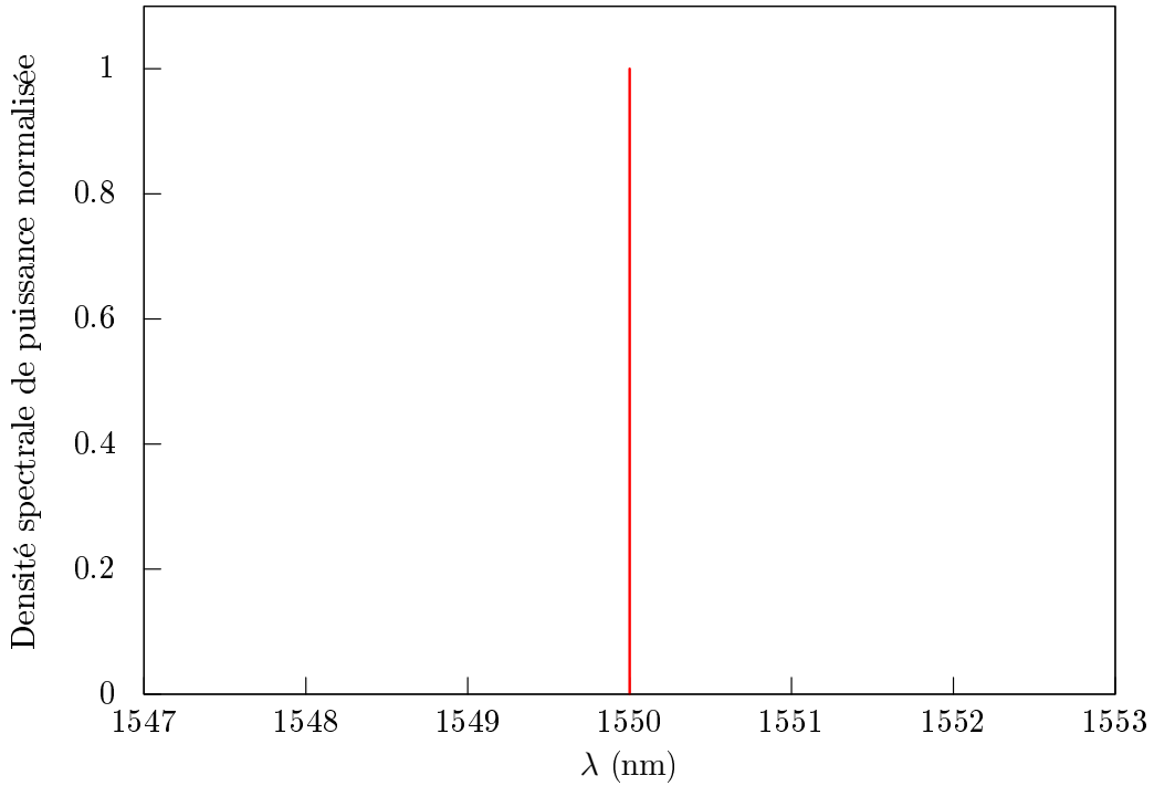
FIGURE 2.2 – Le spectre d'une OPPM est un \delta de Dirac. Toute l'énergie de l'onde est concentrée dans une bande spectrale infiniment fine, ce qui est physiquement irréaliste.
