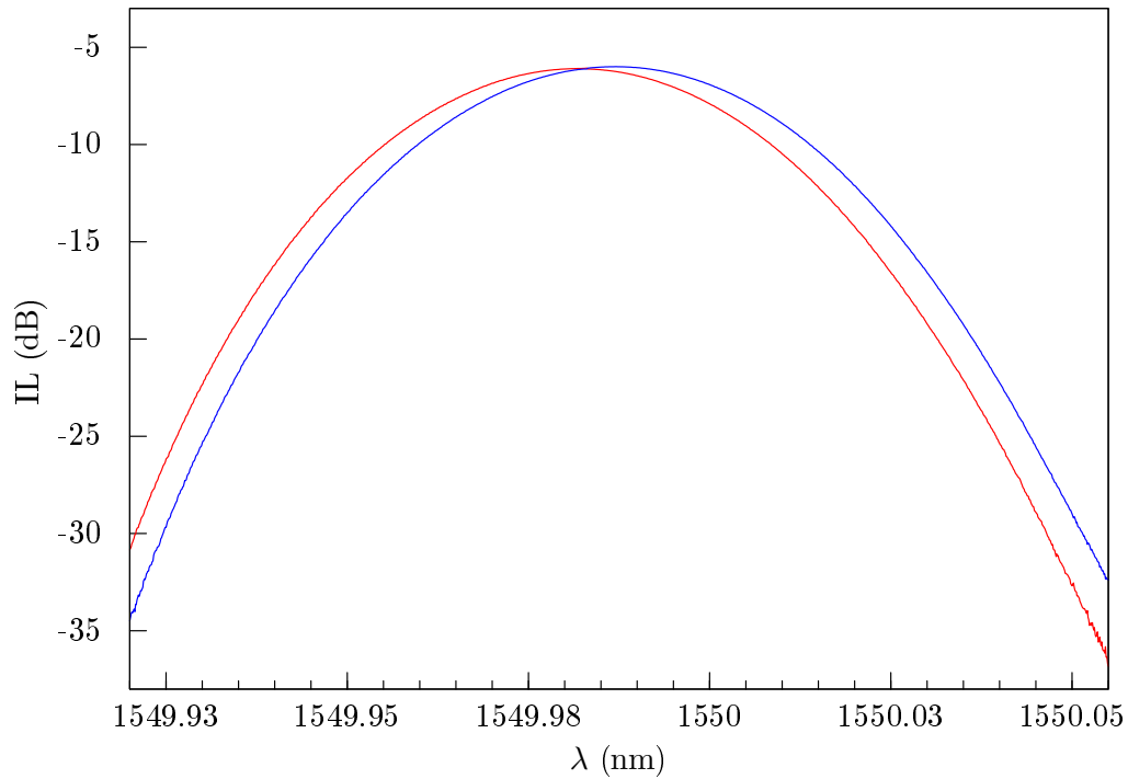
FIGURE 8.10 – Sous-filtres propres de l’XTx-50 n° 1 avec une bande passante de 45 pm. On observe clairement un décalage de la longueur d’onde centrale.
