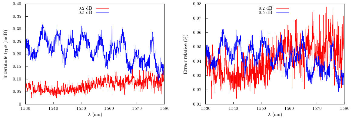
FIGURE 7.12 – Dispersion de la mesure dans des conditions de répétabilité avec le protocole à 6 états. On observe que l’erreur commise est grossièrement constante sur toute la bande de mesure. L’erreur relative est essentiellement identique pour une PDL mesurée de 0,2 dB et 0,5 dB.
