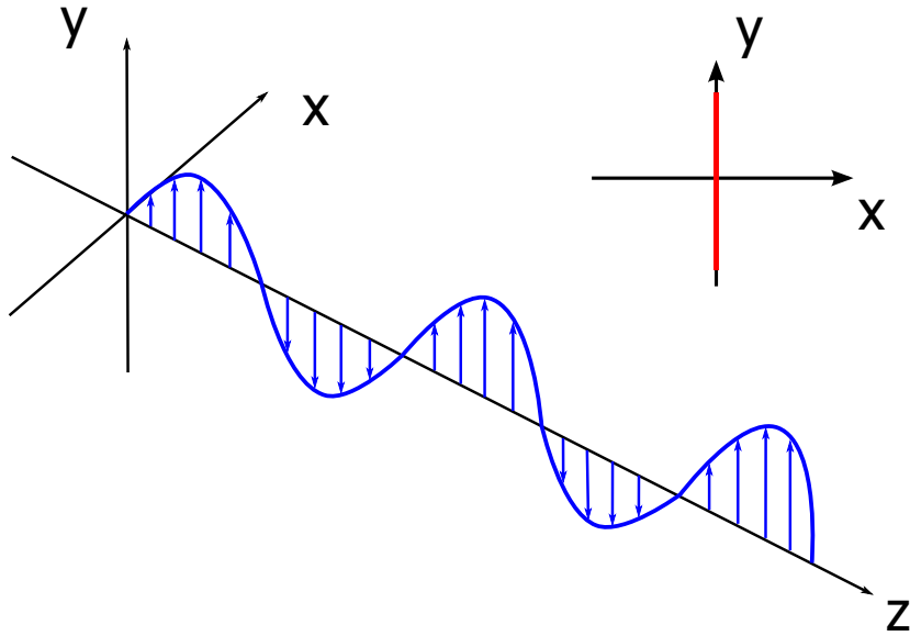
FIGURE 3.3 – Dans le cas d’une polarisation horizontale, l’oscillation du champ électrique décrit une trajectoire rectiligne selon l’axe y .
