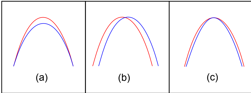
FIGURE 8.2 – Configurations canoniques des sous-filtres propres. (a) Différence d'atténuation. (b) Décalage en longueur d'onde centrale. (c) Différence de bande passante.
