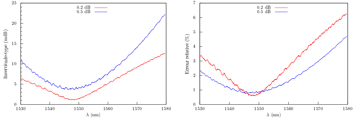
FIGURE 7.19 – Dispersion de la mesure pour le protocole à 4 états avec des états d’entrée variables. On retrouve un comportement similaire à celui déjà observé dans le cadre de l’analyse de la reproductibilité, mais avec une erreur un peu moindre. Par comparaison au protocole à 6 états, l’erreur est entre 2 et 3 fois plus importante.
