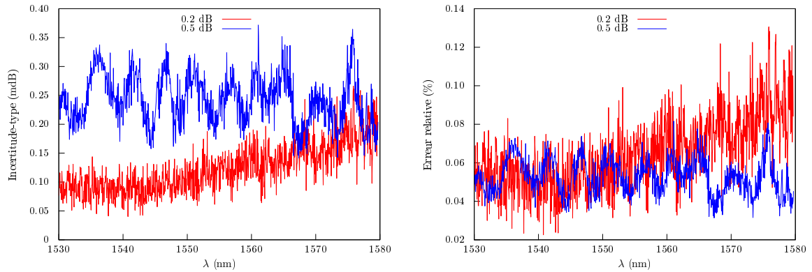
FIGURE 7.13 – Dispersion de la mesure dans des conditions de répétabilité avec le protocole à 4 états. L’erreur commise est de nouveau grossièrement constante sur toute la bande de mesure. L’erreur relative est encore essentiellement identique pour une PDL mesurée de 0,2 dB et 0,5 dB.
