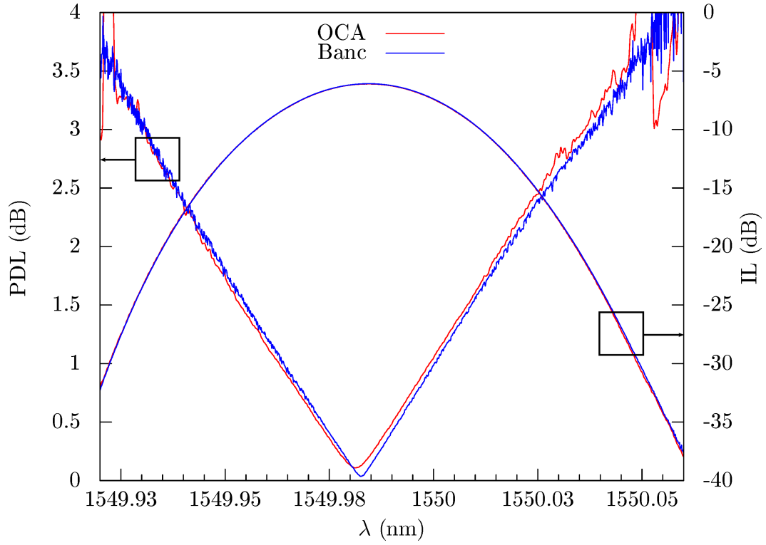
FIGURE 8.7 – PDL et IL de l'XTx-50 n° 1 avec une bande passante de 45 pm. On note le bon accord entre les résultats obtenus avec l'OCA et notre banc, aussi bien au niveau de l'IL que de la PDL.
