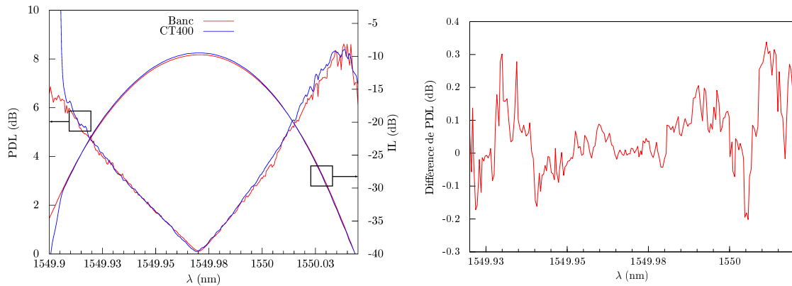
FIGURE 9.3 – (a) Mesure d'un filtre ultrafin de bande passante 32 pm avec le CT400 PDL et comparaison avec le banc de mesure. (b) Différence des PDL mesurées. Compte tenu des incertitudes de mesure propres à chaque dispositif, les résultats sont comparables. Grâce à sa très bonne répétabilité en longueur d'onde, le CT400 permet la mesure de filtres ultrafins.
