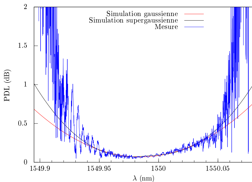
FIGURE 8.19 – Comparaison entre la PDL simulée et la PDL mesurée pour l'XTx wide. Les simulations retranscrivent bien la PDL mesurée. Le modèle supergaussien est plus efficace sur les bords.
