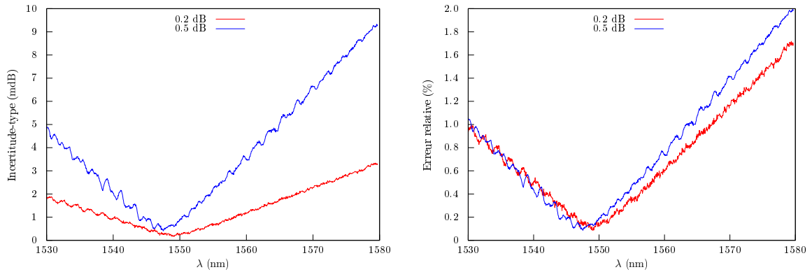
FIGURE 7.18 – Dispersion de la mesure pour le protocole à 6 états avec des états d'entrée variables. Contrairement au cas de l'analyse de la reproductibilité, on retrouve l'influence du désalignement angulaire du PSG. L'erreur commise est clairement corrélée à la PDL mesurée.
