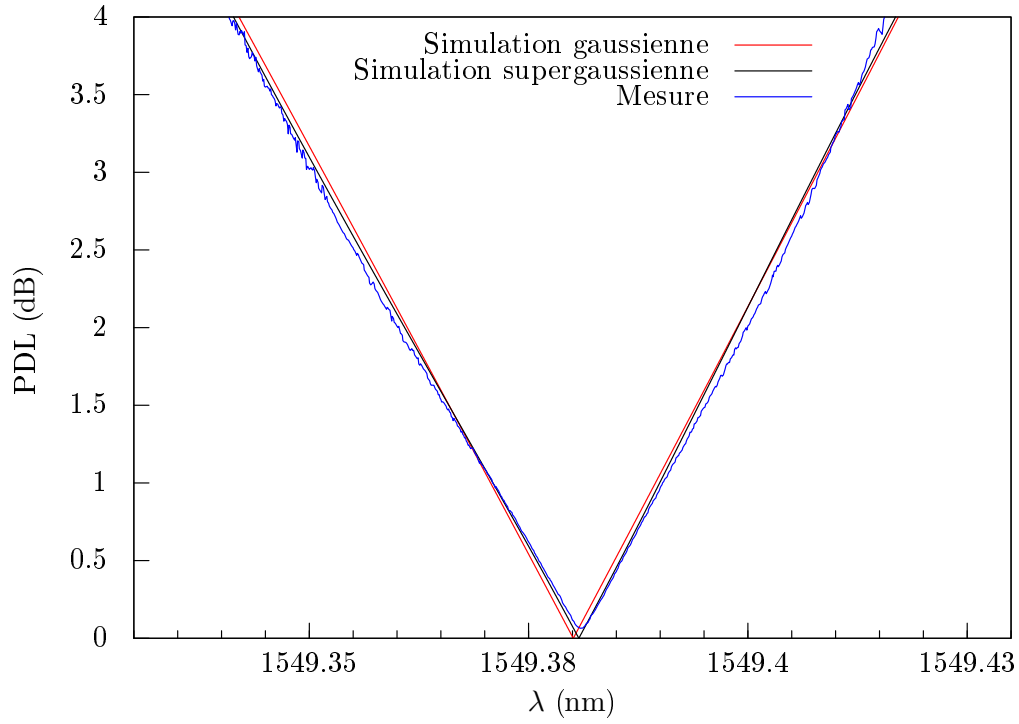
FIGURE 8.16 – Comparaison entre la PDL simulée et la PDL mesurée pour l'XTx-50 n° 2. La simulation et la mesure coïncident encore.
