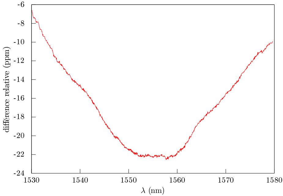
FIGURE 7.9 – Étalon à 0,2 dB. Différence relative entre la PDL calculée dans le cas matriciel et le cas vectoriel. L'écart est de l'ordre de la vingtaine de ppm, c'est à dire du même ordre de grandeur que celui relevé dans le cas de l'étalon à 0,5 dB.
