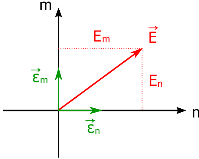
FIGURE 2.4 – Décomposition du vecteur champ électrique de dimension 2 sur une base formée de deux vecteurs unitaires orthogonaux du plan transverse à la direction de propagation.
