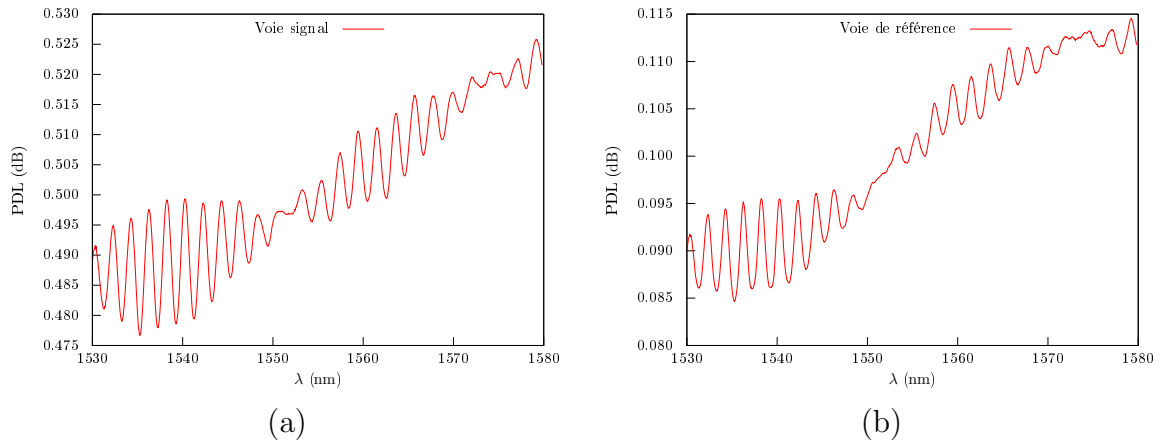
FIGURE 7.2 – Étalon à 0,5 dB. (a) PDL totale de la voie signal en présence du DUT. Elle est de l'ordre de la PDL attendue et on retrouve des variations très similaires à celles qui existaient déjà sur la voie signal en l'absence du DUT. (b) PDL totale de la voie de référence en présence du DUT. Elle est sensiblement identique à celle obtenue lors de la calibration, l'écart pouvant être mis sur le compte de la reproductibilité de la mesure.
