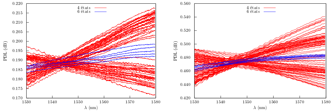
FIGURE 7.14 – Reproductibilité de la mesure pour l'étalon à 0,2 dB et 0,5 dB. Dans le cas du protocole à 4 états, on observe que la dispersion est minimale pour une longueur d'onde située entre 1540 nm et 1550 nm puis tend à augmenter de façon symétrique de part et d'autre. La dispersion est nettement plus faible avec le protocole à 6 états et paraît grossièrement indépendante de la longueur d'onde.
