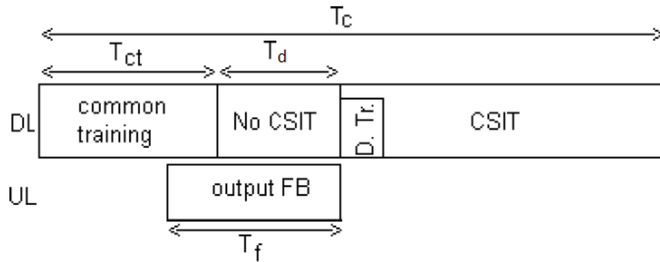
(b) Topologie d'un bloc pour étude de net DoF.
