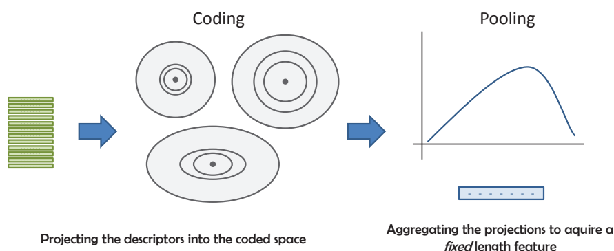
FIGURE B.4: Codage et agrégation des caractéristiques de bas niveau pour générer un descripteur résumé de l'image.
