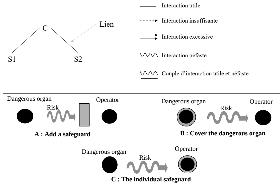
Figure 14. Exemple de modèle substance-champ (en haut) et solutions de prévention proposées par TRIZ (Hasan et al., 2004)
