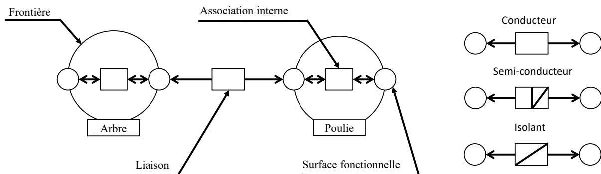
Figure 19. Modèle fonctionno-structural d'un système arbre-poulie
