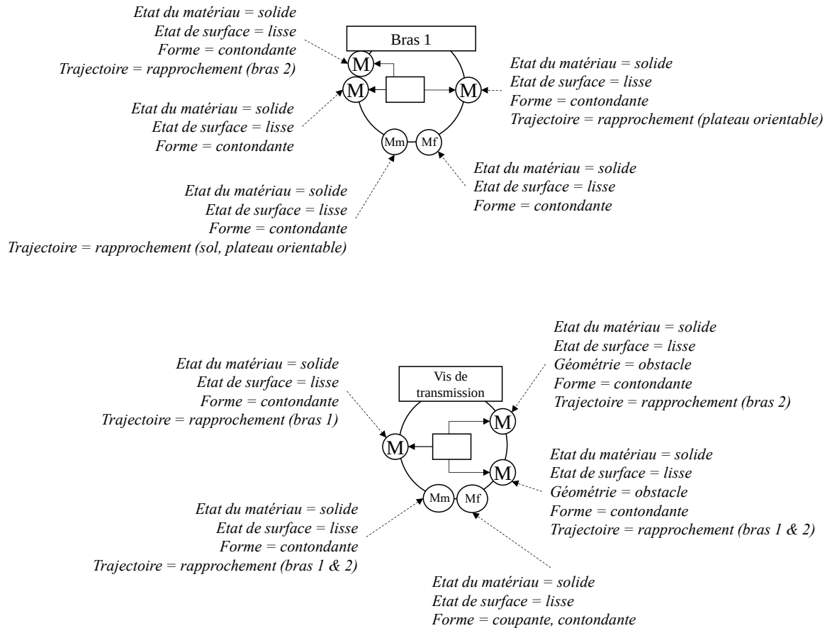
Figure 35. Paramètres complémentaires des éléments « Vis de transmission » et « Bras 1 » du cric mécanique
