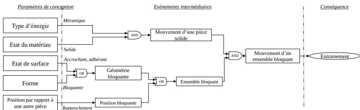
Figure 49. Extrait de l'arbre des causes
