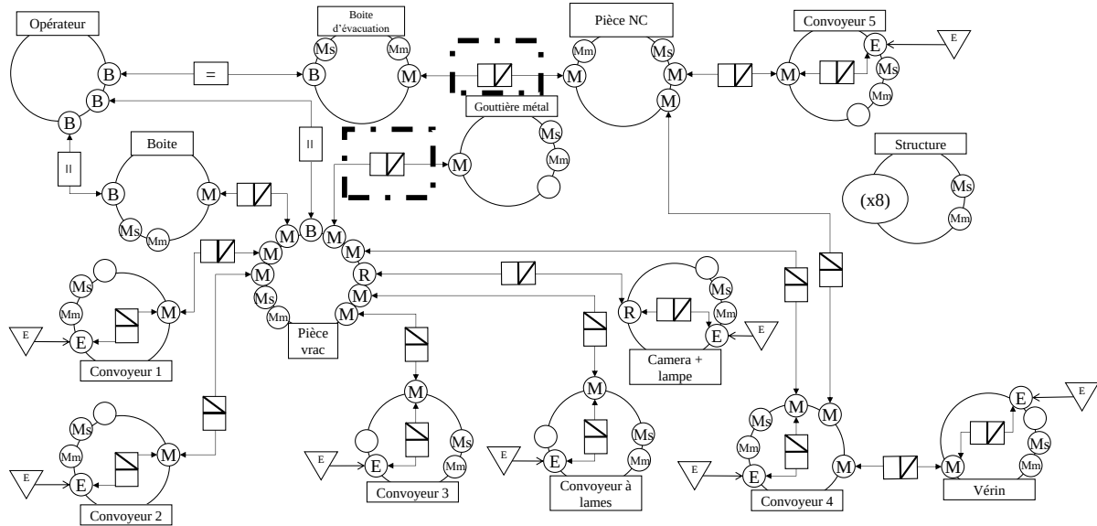
Figure 48. MFS de la ligne d'approvisionnement basée sur le visuel de la solution (pour la phase de vie d'utilisation de la machine)
