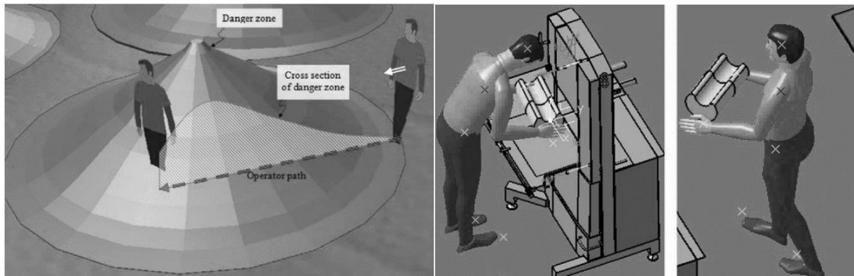
Figure 11. Calcul du niveau de risque auquel est exposé un opérateur en fonction de sa trajectoire (à gauche) et de son activité (à droite)
