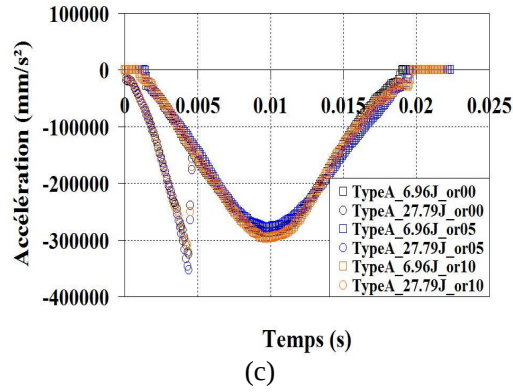
Figure A.10 Réponses caractéristiques avec pré-tension des renforts et l'inclinaison de l'éprouvette en déplacement et ses dérivées pour l'éprouvette Type A : (a) Courbes : déplacement - temps, (b) Courbes : vitesse d'impact - temps, (c) Courbes : accélération - temps
