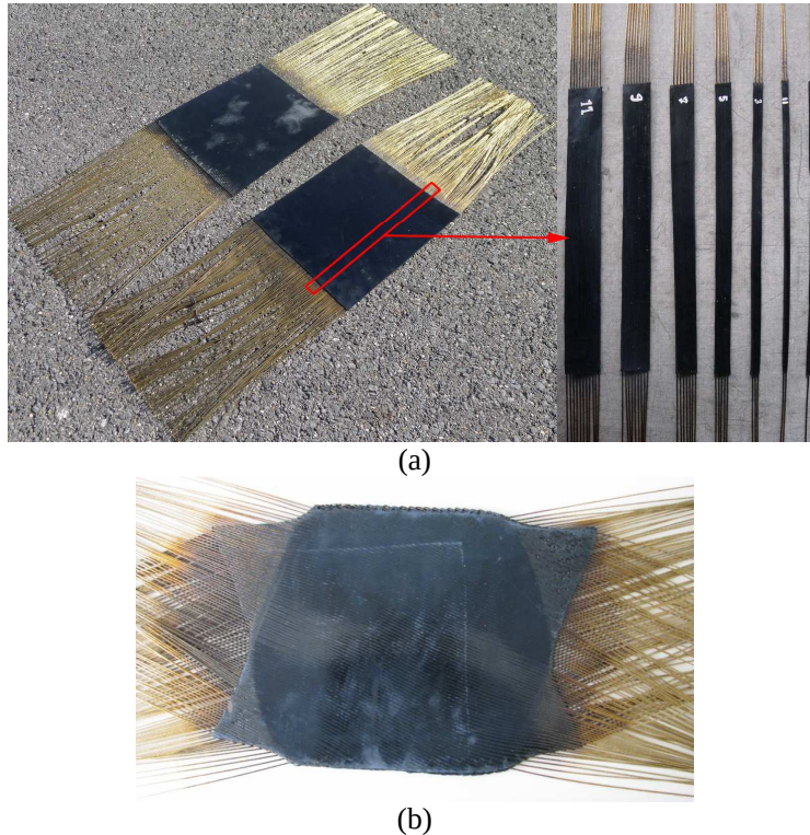
Figure VI.1 Eprouvettes pour essais d'indentation avec les câbles nus en bout de plaque : (a) Avec plusieurs brins de renforts, (1 à 11 brins), et (b) Une bi-nappe croisée de type A
