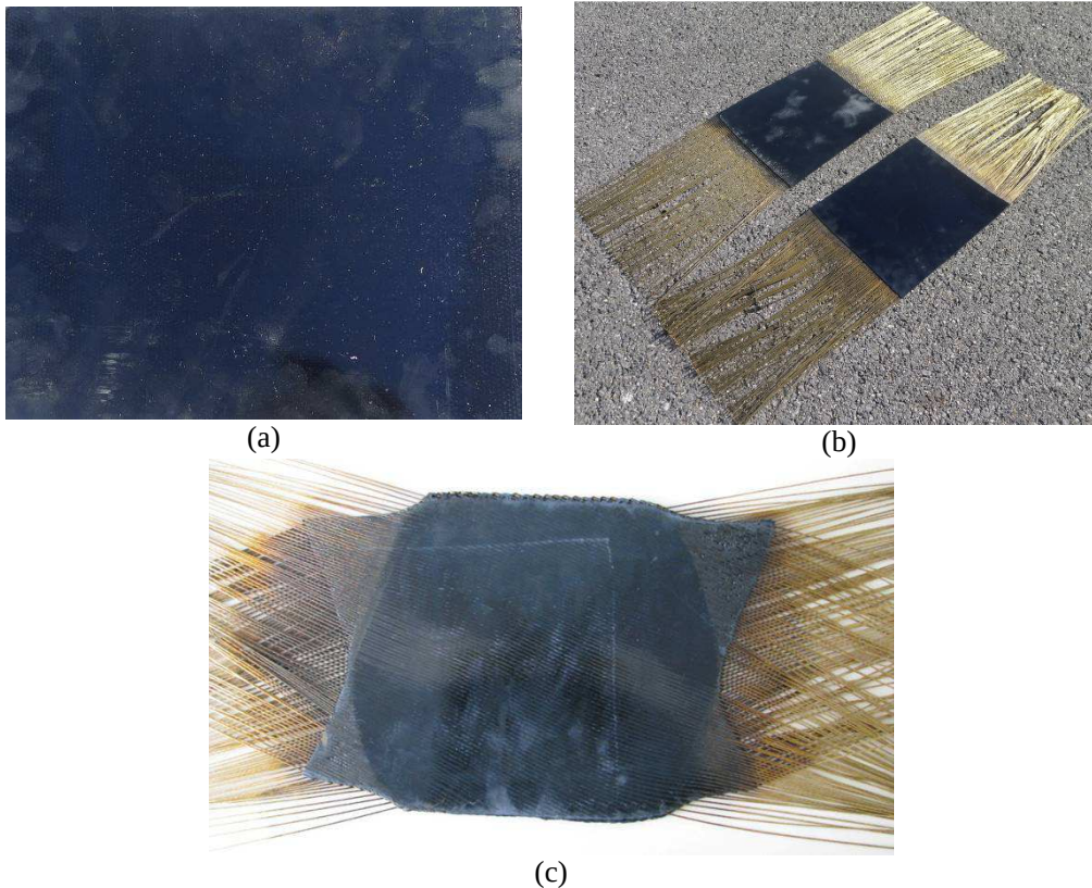
Figure V.10 Eprouvettes pour essai d'impact par masse tombante et pour essai d'indentation : (a) Mono-nappe sans et (b) Avec les câbles nus en bout de plaque, (c) Bi-nappe croisée [+20°,-20°] avec les câbles nus en bout de plaque
