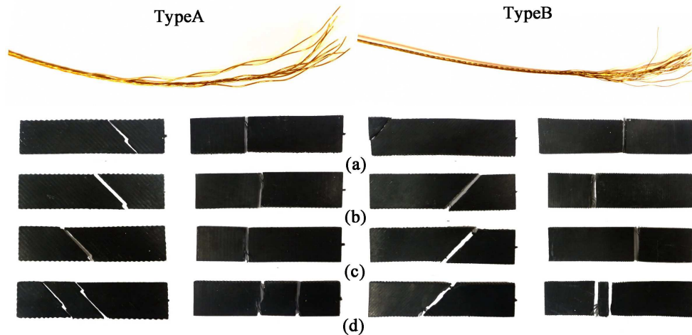
Figure III.29 Endommagement des éprouvettes pour différentes vitesses de déformation : (a) 3,3 \times 10^{-3} \text{ s}^{-1} , (b) 1,2 \text{ s}^{-1} , (c) 26 \text{ s}^{-1} , (d) 131 \text{ s}^{-1}
