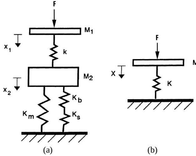
Figure V.2 Schéma des modèles pour une réponse sous l'impact [Abrate, 2001] : (a) Modèle d'ordre 2 ; (b) Modèle d'ordre 1
