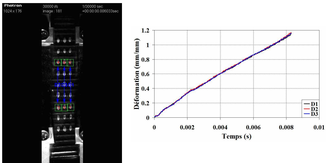
Figure III.13 Champ de déformation pour une vitesse de déformation de 131 \text{ s}^{-1} (l'éprouvette de Type A à 90^\circ )
