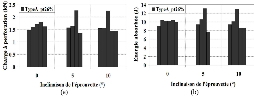
Figure V.25 Résistances à la perforation en fonction de l'angle de l'inclinaison de l'éprouvette avec une pré-tension initiale de 650 N/renfort : (a) Charge maximale, (b) Energie absorbée
