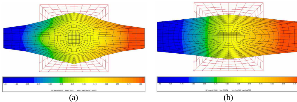
Figure IV.17 Déformation des maillages pour l'éprouvette dans la direction transverse à la déformation de 1,05 : (a) Aucun d'endommagement (b) Endommagement équivalent
