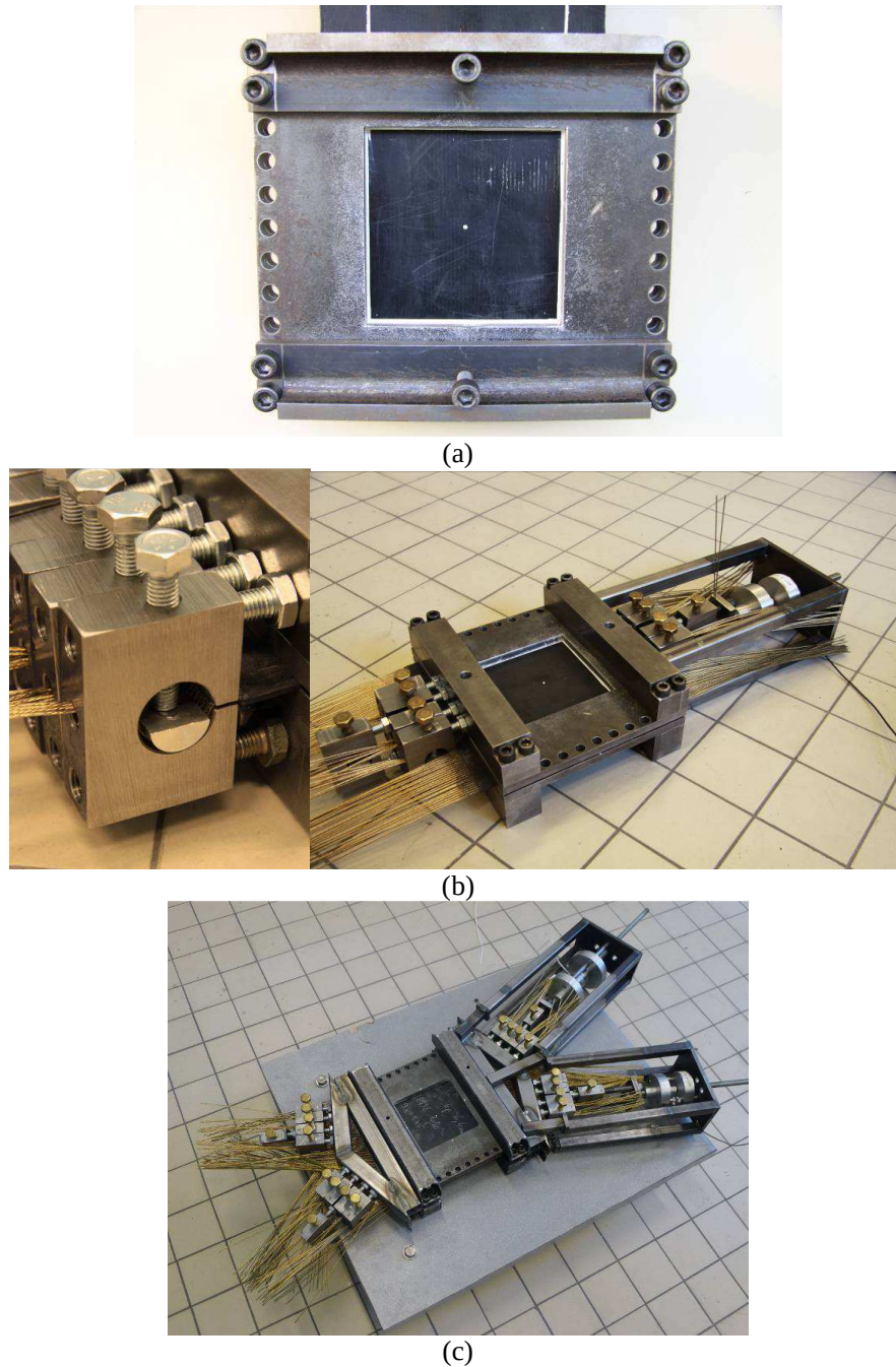
Figure V.13 Encastrement pour : (a) Les essais d'impact sans pré-tension des renforts, (b) Avec pré-tension des renforts sur une mono nappe et (c) Avec pré-tension des renforts sur une binappe croisée [+20^{\circ}, -20^{\circ}]
