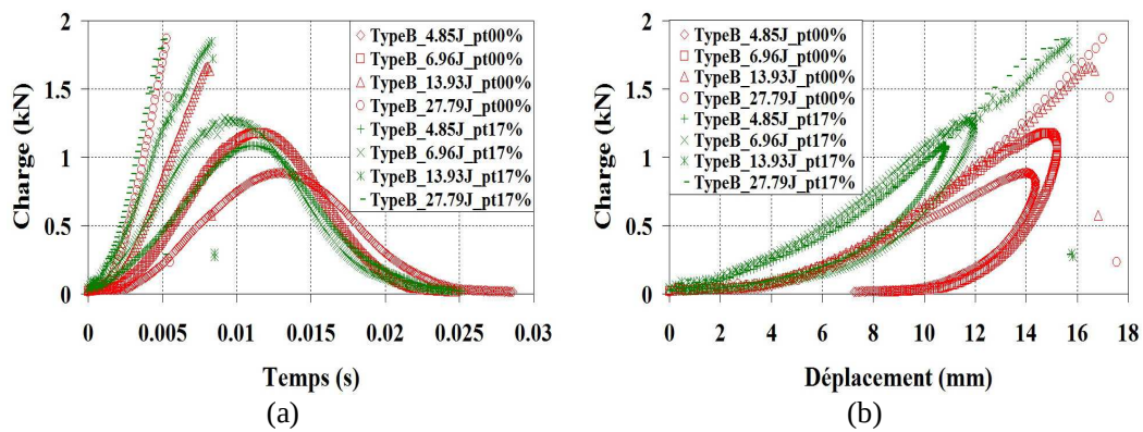
Figure A.7 Réponses caractéristiques avec pré-tension des renforts en charge pour l'éprouvette Type B : (a) Courbes : charge - temps, (b) Courbes : charge - déplacement
