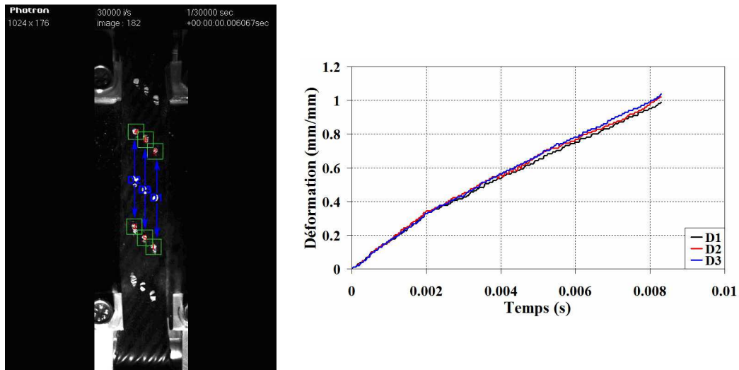
Figure III.12 Champ de déformation pour une vitesse de déformation de 131 \text{ s}^{-1} (l'éprouvette de Type A à 45^\circ )
