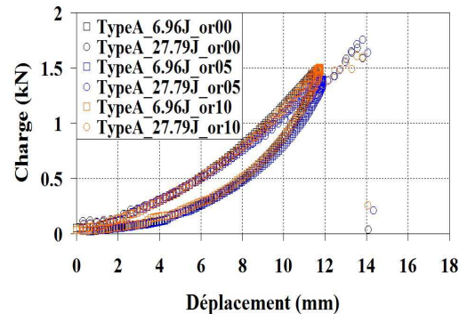
Figure V.21 Courbes : charge - déplacement pour l'éprouvette de type A avec pré-tension et inclinaison des éprouvettes
