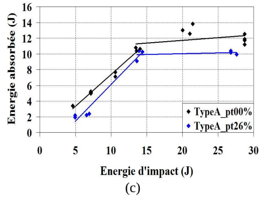
Figure V.24 Résistance à la perforation avec et sans pré-tension initiale de 650 N/renfort : (a) Courbe : charge maximale - énergie d'impact, (b) Courbe : déplacement maximal - énergie d'impact, (c) Courbe : énergie absorbée - énergie d'impact
