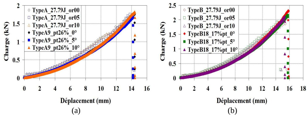
Figure VI.10 Comparaisons des résultats expérimentaux d'essais d'impact par masse tombante et d'essais d'indentation : (a) Echantillons mono-couche sans pré-tension des renforts, (b) Echantillons bi-couche croisés et échantillons mono-couche avec des brins de renfort en nombre suffisant
