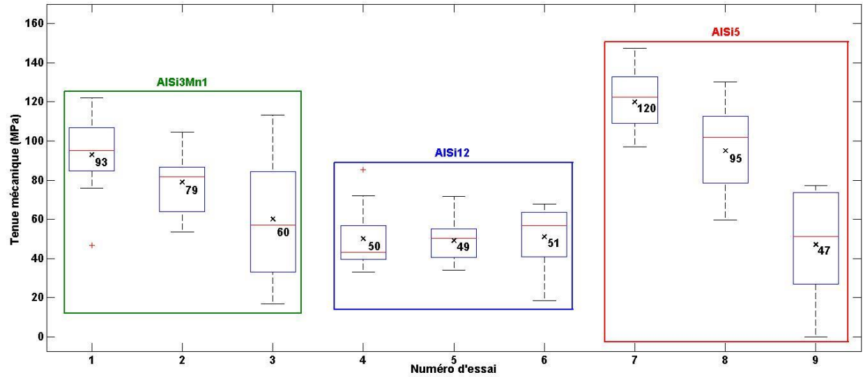
Figure III.9 – Tenue mécanique (MPa) pour chacun des essais. Les moyennes sont représentées par les croix noires et leurs valeurs sont inscrites également en noir directement sur la figure, les médianes sont représentées par les traits rouges et les valeurs extrêmes par les traits noirs. Les rectangles bleus représentent les intervalles où sont situées entre 25 et 75% des valeurs.
