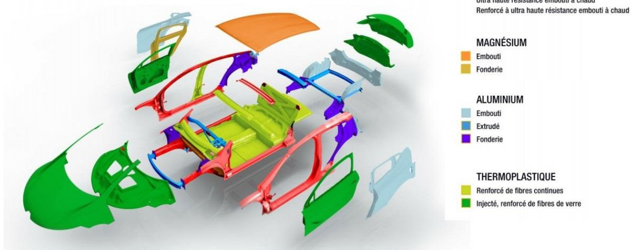
Figure 1-Répartition des matériaux sur la caisse du prototype EOLAB de l'entreprise Renault [3].
