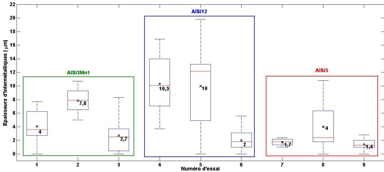
Figure III.10 – Epaisseurs d'intermétalliques (µm) pour chacun des essais. Les moyennes sont représentées par les croix noires et leurs valeurs sont inscrites également en noir directement sur la figure, les médianes sont représentées par les traits rouges et les valeurs extrêmes par les traits noirs. Les rectangles bleus représentent les intervalles où sont situées entre 25 et 75% des valeurs.
