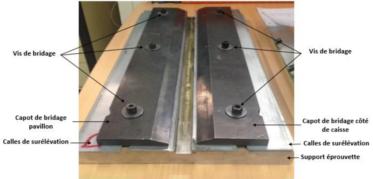
Figure II.8 – Photo du support éprouvette.
