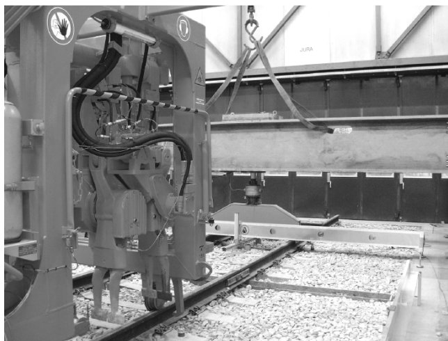
Figure III.6 : Dispositif d'essai – Bloc bourroir 1x et poutre de sollicitation (Paderno 2010)
