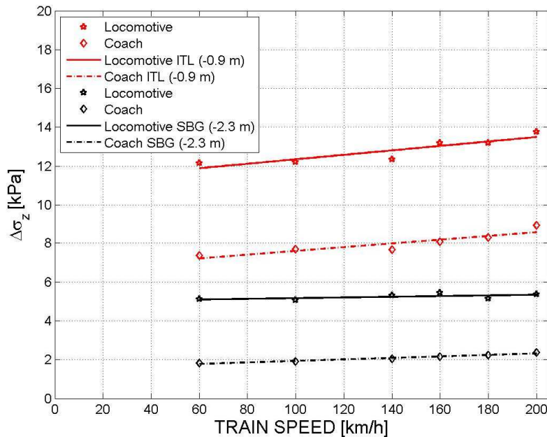
Figure V.16 : Contrainte maximale mesurée en fonction de la vitesse et de la masse du mobile (Lamas-Lopez, 2016)
