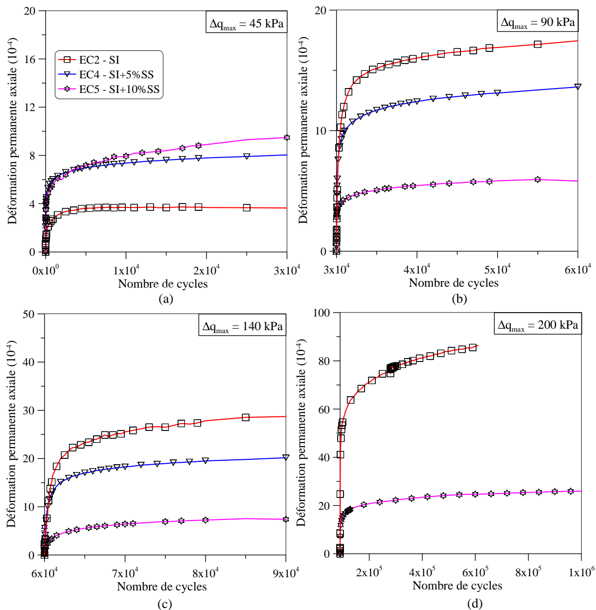
Figure IV.24 : Essais EC2, EC4 et EC5 – Déformation permanente axiale en fonction du nombre de cycles : (a) 1 er palier (b) 2 e palier (c) 3 e palier (d) 4 e palier (Trinh, 2011)
