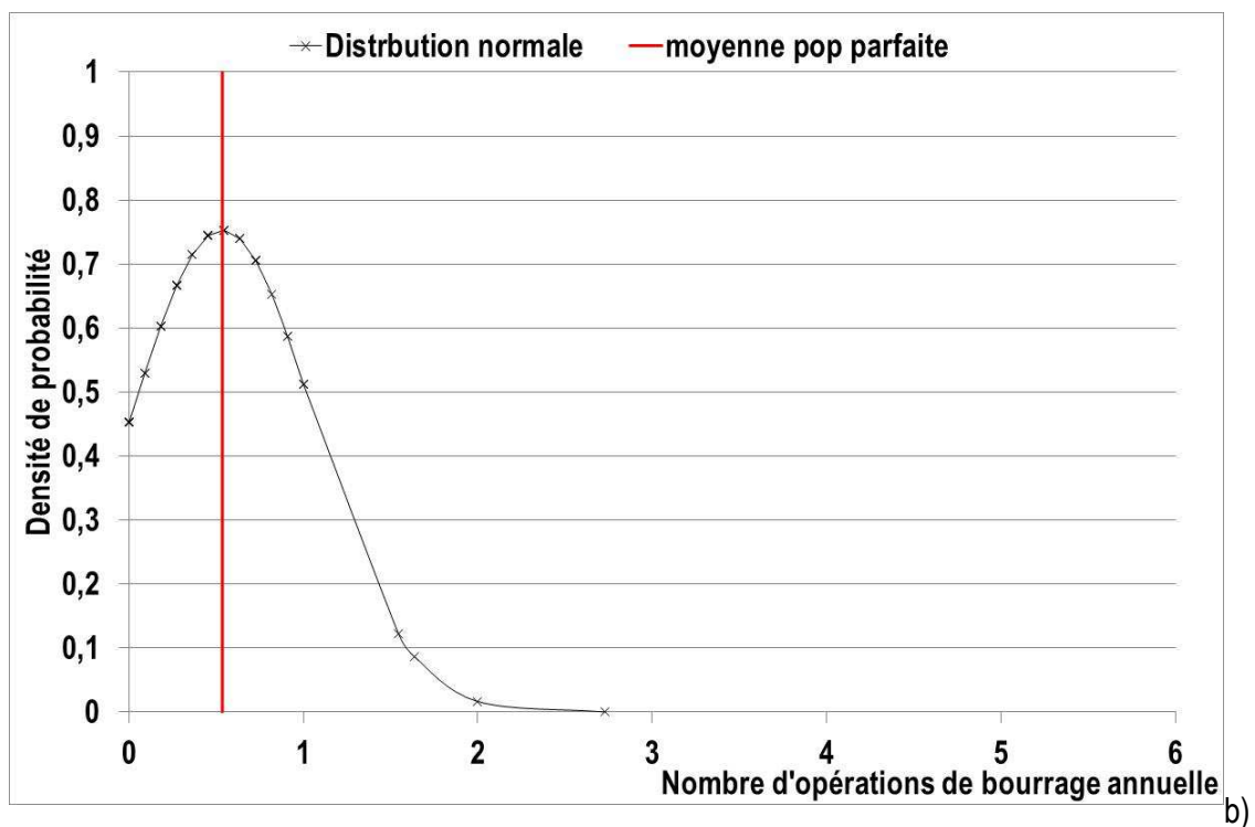
Figure VI.14 : Répartition statistique des tronçons des groupes 3 (a) et 4 (b) après 11 années d'exploitation
