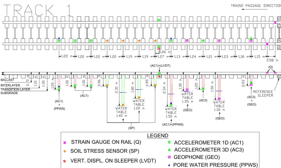
Figure V.6 : Implantation des capteurs sur le site de Vierzon en V1 (Lamas-Lopez, 2016)
