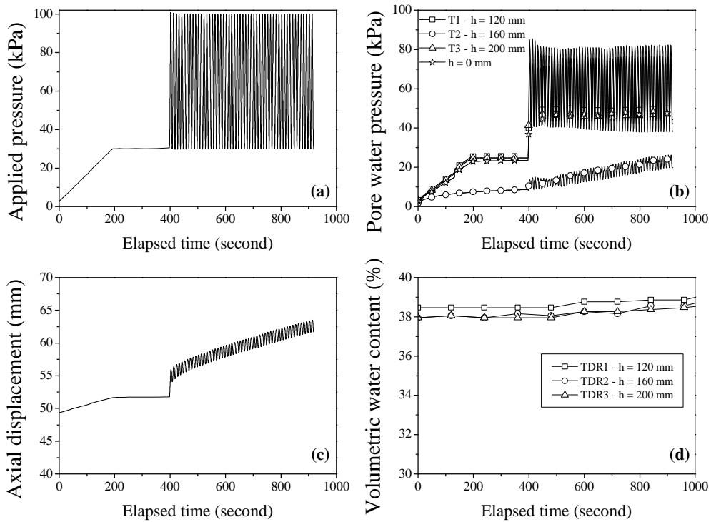
Figure III.15 : Comportement de l'échantillon \rho_{d-initial}=1,4\text{Mg/m}^3 : a) contrainte appliquée ; b) pression interstitielle ; c) déplacement du piston ; d) teneur en eau volumique (Duong 2013)
