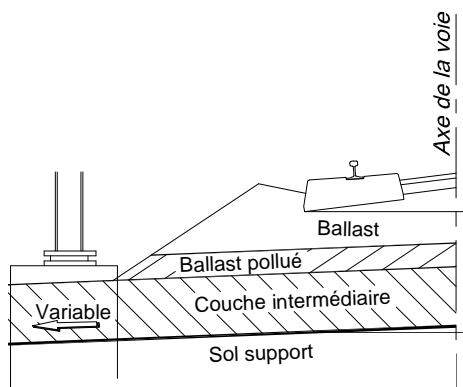
Figure 1.9 : Structure classique (SNCF, 1996)
