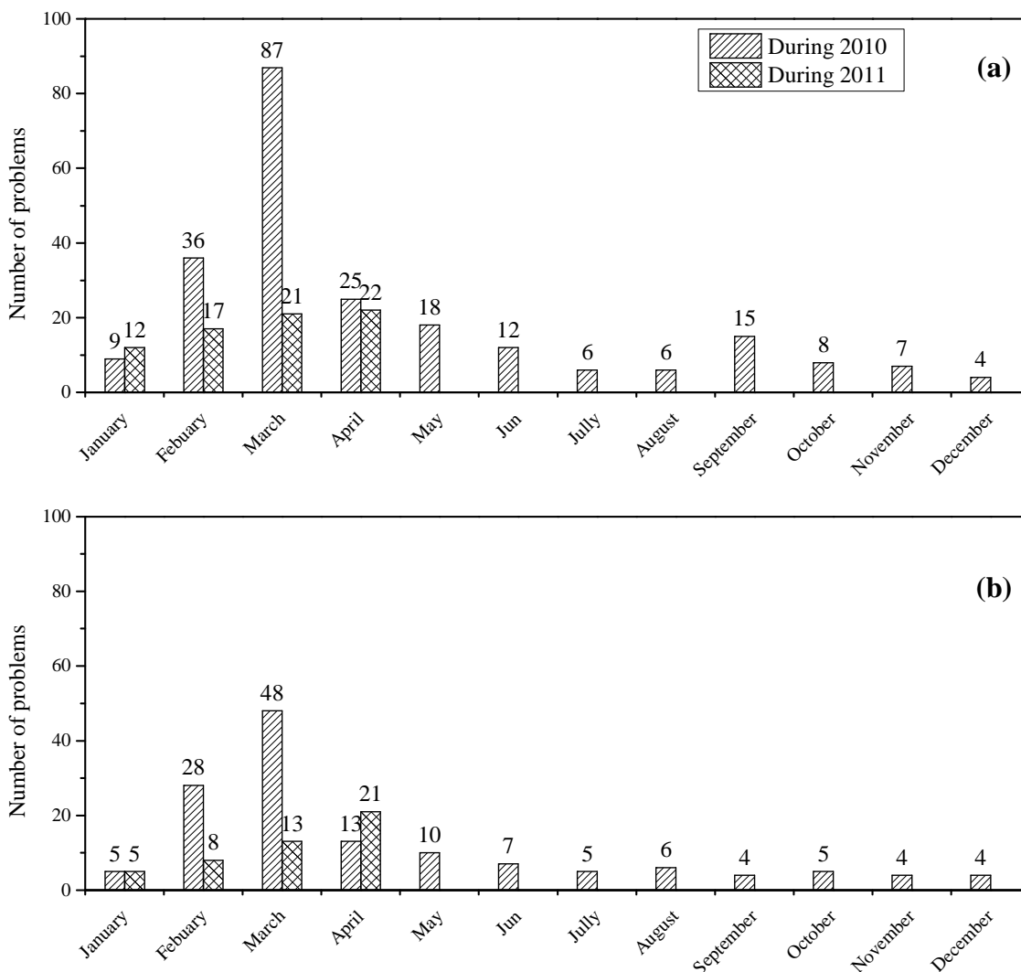
Figure 1.21 : Problèmes survenant au cours d'une année. a) Problèmes liés à l'infrastructure et la b) problèmes liés aux zones sensibles (Duong, 2013)
