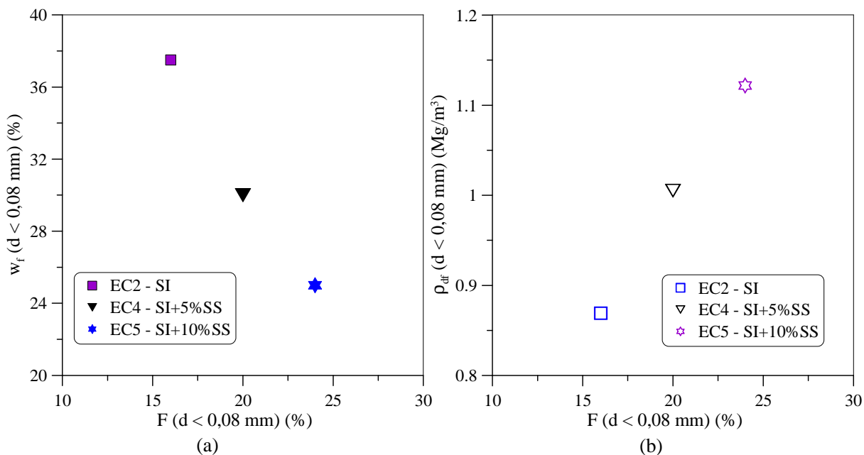
Figure IV.33 : Partis inférieures à 0,08 mm pour les essais EC2, EC4 et EC5 : (a) évolution de la teneur en eau (a) et évolution de la masse volumique sèche (b) en fonction de la teneur en fines (Trinh, 2011)
