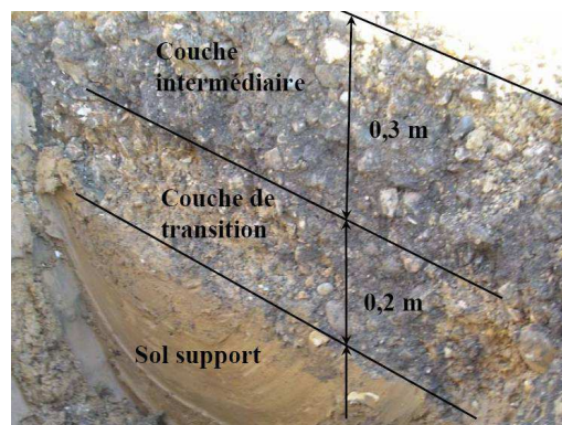
Figure 1.10 : Stratigraphie des structures anciennes (Trinh, 2011)
