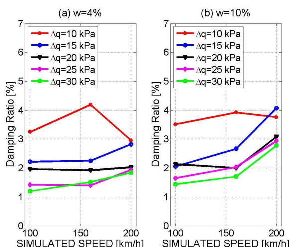
Figure V.34 : Evolution du coefficient d'amortissement en fonction de la teneur en eau et de la vitesse (Lamas-Lopez, 2016)
