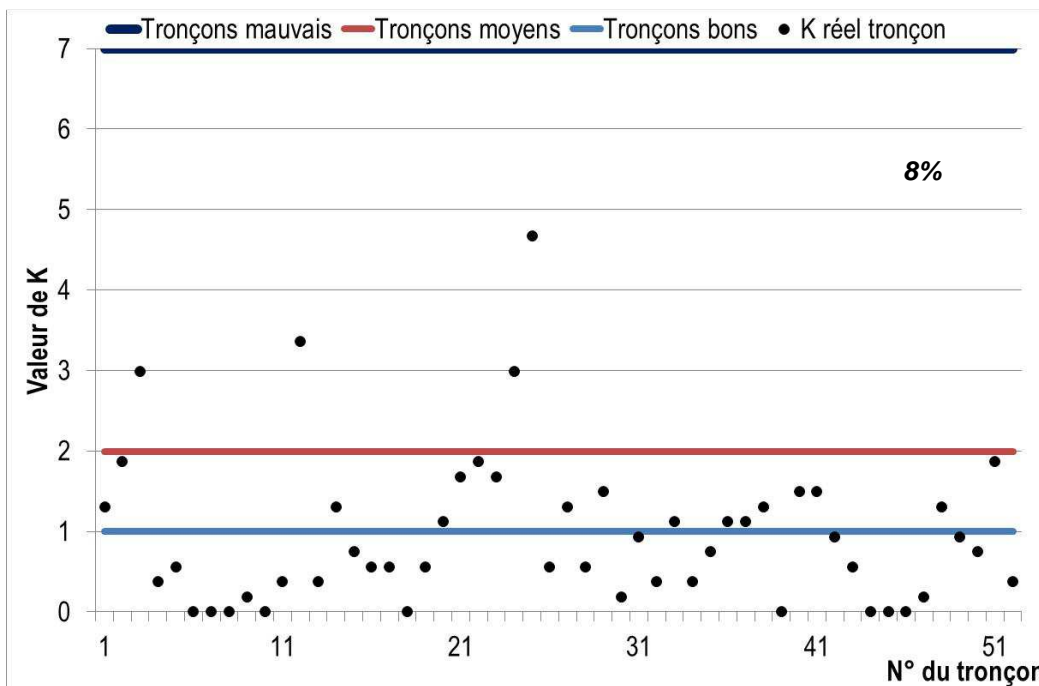
Figure VI.17 : Cotation des tronçons groupe UIC 4
