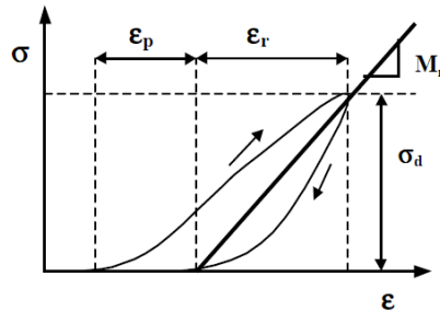
Figure V.19 : Définition du module réversible ( M_r )
