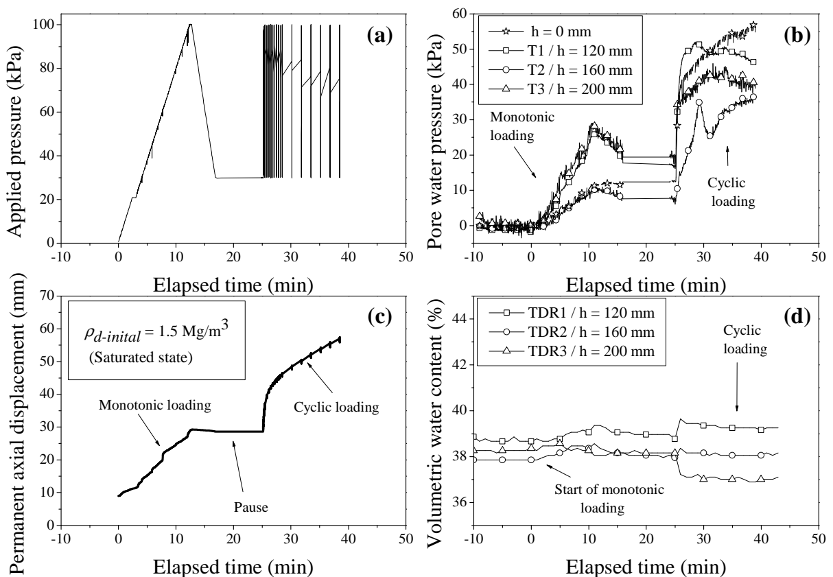
Figure III.17 : Comportement de l'échantillon \rho_{d-initial} = 1,5 \text{ Mg/m}^3 : a) contrainte appliquée ; b) pression interstitielle ; c) déplacement du piston ; d) teneur en eau volumique (Duong 2013)
