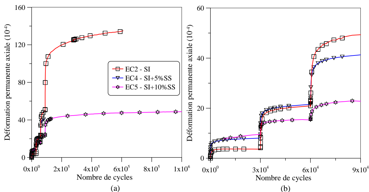
Figure IV.23 : Essais EC2, EC4 et EC5 – Déformation permanente axiale en fonction du nombre de cycles : (a) essais complets, (b) trois premiers paliers (Trinh, 2011)
