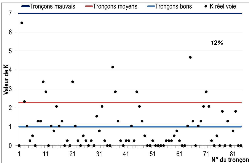
Figure VI.15 : Cotation des tronçons groupe UIC 3
