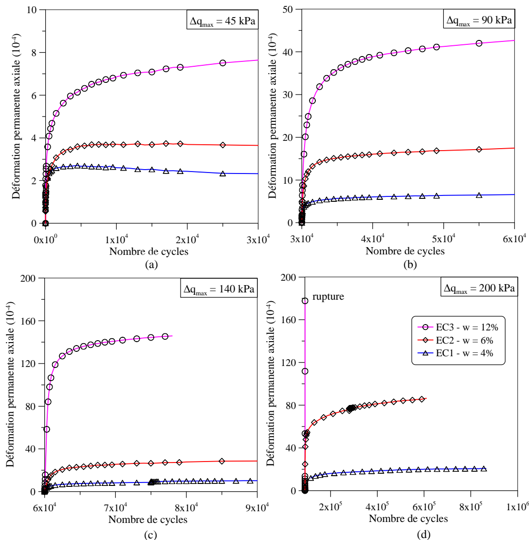
Figure IV.18 : Essais EC1, EC2, EC3 – Déformation permanente axiale en fonction du nombre de cycles : (a) 1 er palier, (b) 2 e palier, (c) 3 e palier, (d) 4 e palier (Trinh, 2011)
