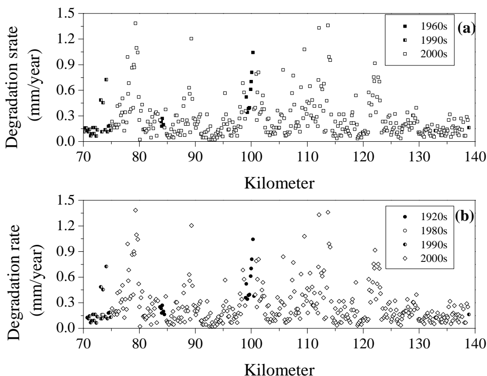
Figure 1.30 : La vitesse de dégradation de la voie 1 selon (a) l'année de pose du rail et (b) l'année de pose de la traverse (Duong, 2013)
