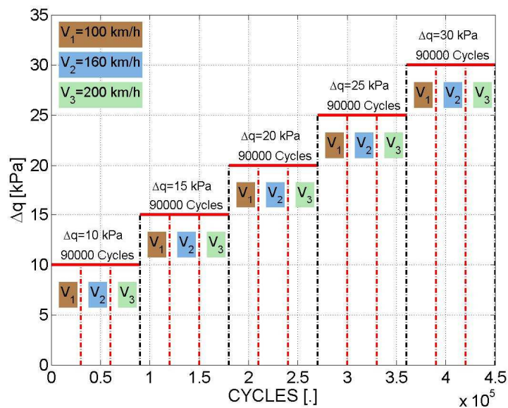
Figure V.29 : sollicitation cyclique appliquée à l'échantillon (Lamas-Lopez, 2016)
