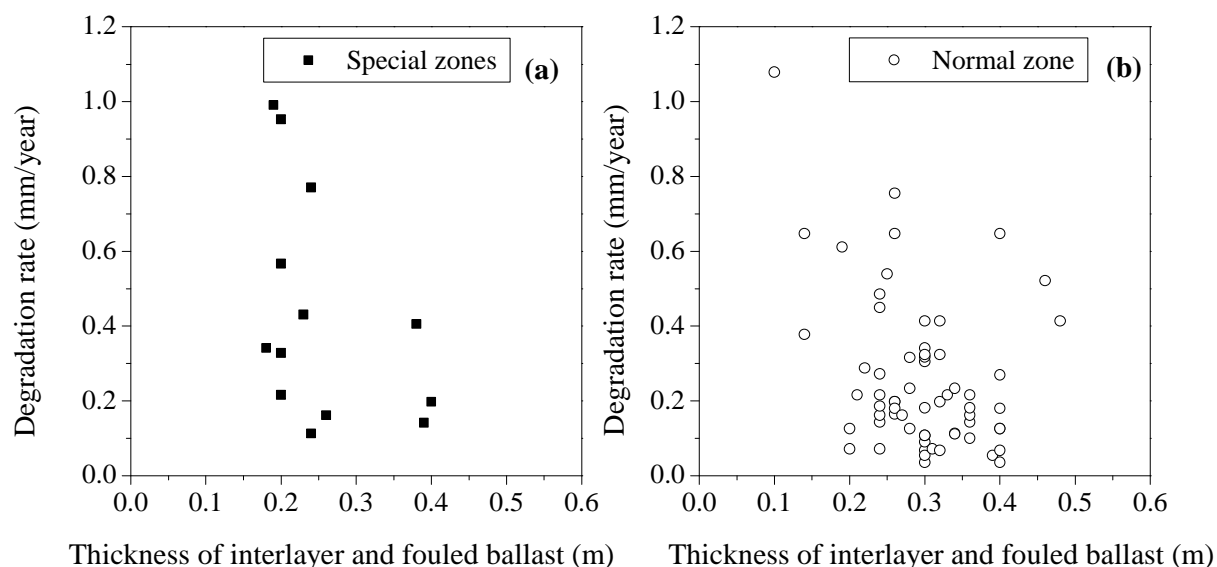
Figure 1.33 : Corrélation entre la vitesse de dégradation du NL et l'épaisseur du ballast couche intermédiaire et colmaté pour la voie 1 - données de train carotteur. a) des zones singulières et b) zone normale (Duong, 2013)
