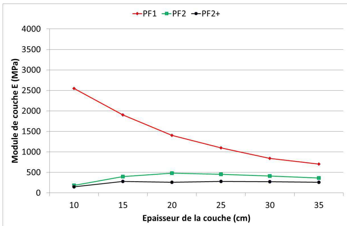
Figure VI.4 : Module d'élasticité nécessaire à la traficabilité en fonction de la classe de plateforme et de l'épaisseur de CI
