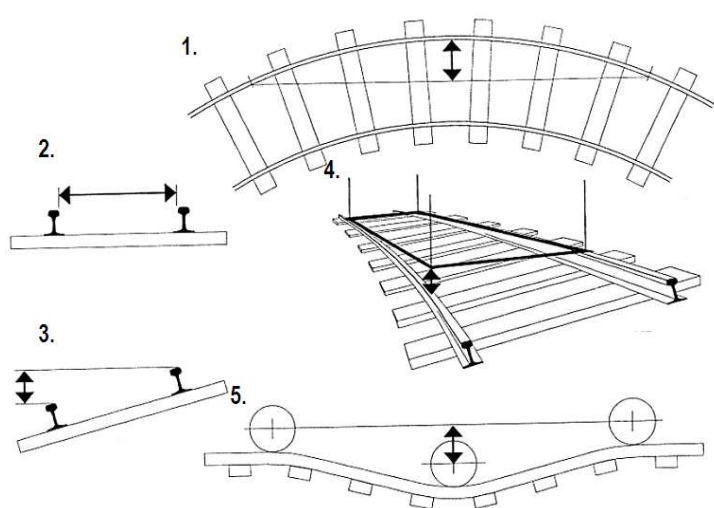
Figure I.11 : Critères de géométrie de la voie
