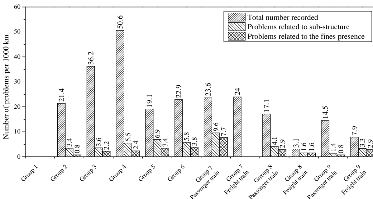
Figure I.20 : Nombre de problèmes par rapport aux groupes UIC (Duong, 2013)
