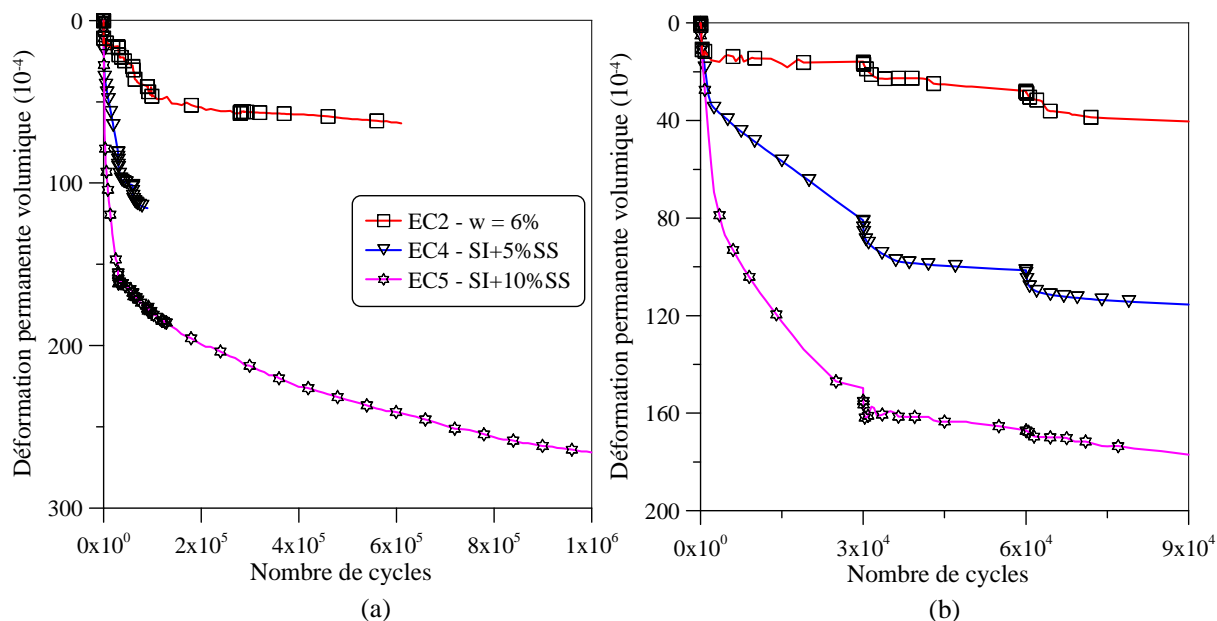
Figure IV.26 : Essais EC2 ; 4 & 5 – Déformation permanente volumique en fonction du nombre de cycles : (a) essais complets, (b) trois premiers paliers (Trinh, 2011)
