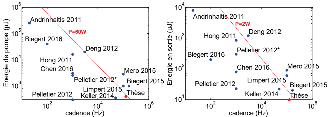
Fig. 9 : Etat de l'art classifié des OPCPA selon la cadence et l'énergie par impulsion de leurs pompes, ou selon la cadence et l'énergie dans le milieu infrarouge en sortie du système.
