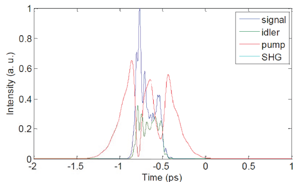
Fig. 56 : Profil temporel en sortie d'OPA 3.
