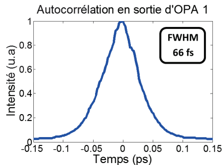
Fig. 62 : Récapitulatif des performances du 1 er étage.
