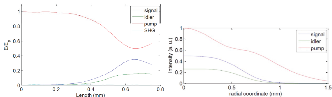
Fig. 57 : Evolution de l'énergie de pompe, de signal et d'idler durant l'OPA 3 à gauche. Profil spatiaux des faisceaux en fin d'étage à droite.
