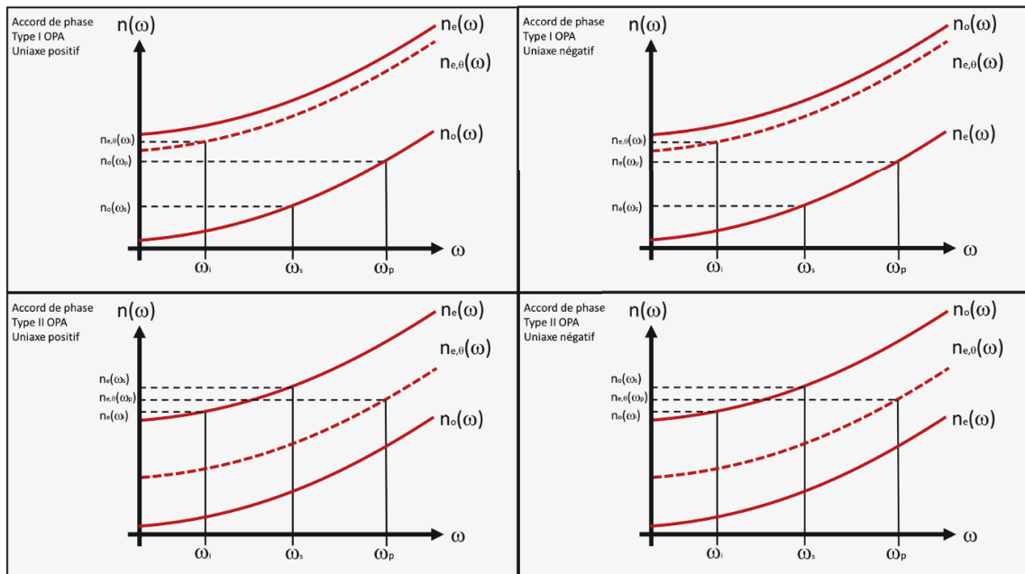
Fig. 22 : Accord de phase de type I et II pour un mélange à 3 ondes par biréfringence dans un milieu non linéaire uniaxe positif ou négatif
