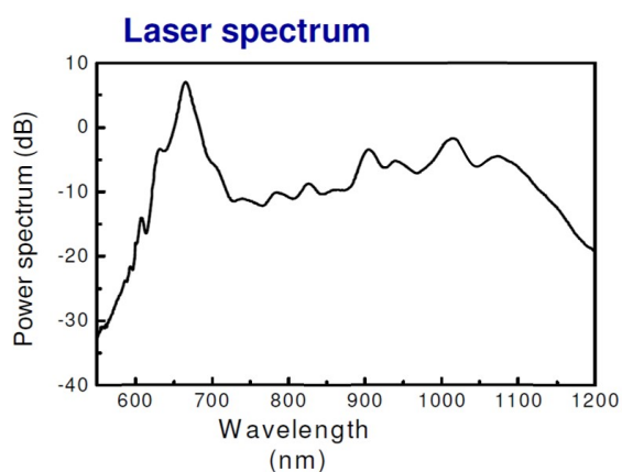
Fig. 10 : Spectre de l'oscillateur Ti:Sa dans (Hong, et al., 2011).
