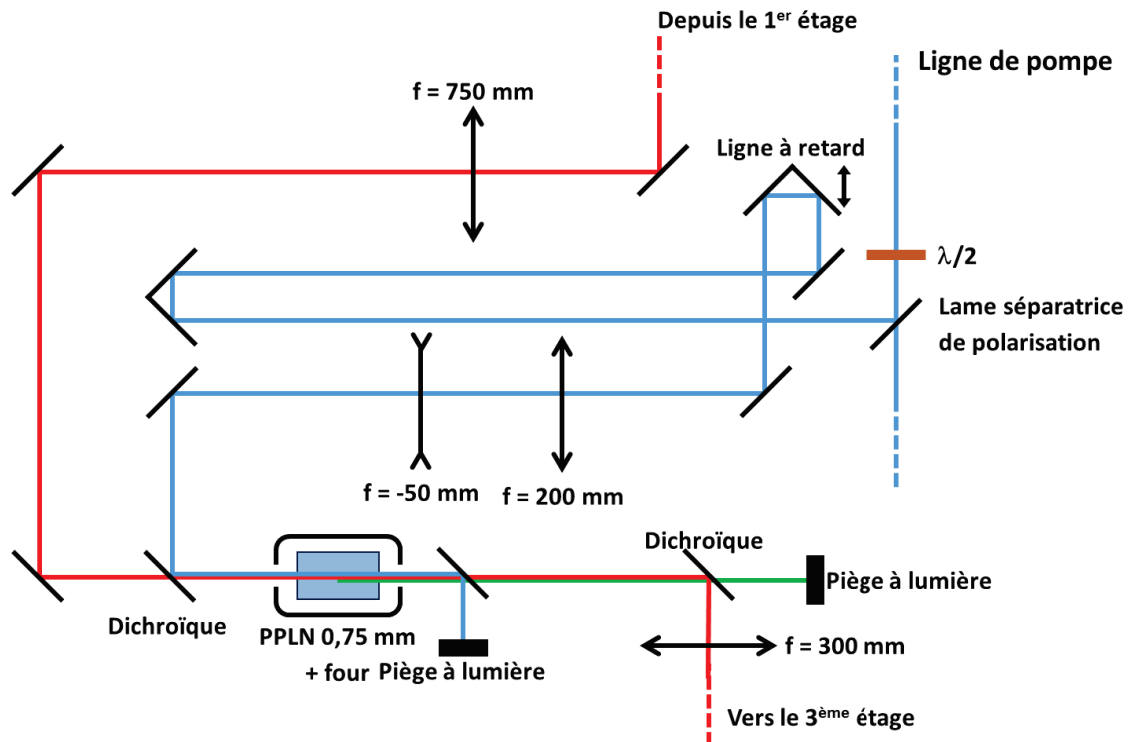
Fig. 64 : Récapitulatif de l'implémentation du 2 ème étage.
