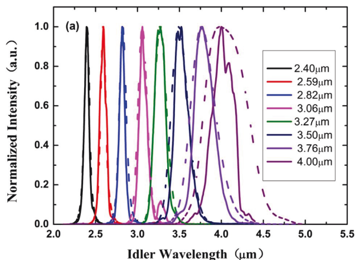
Fig. 11 : Accordabilité de l'OPCPA (Chen, Li, Li, Guo, & Leng, 2016). En trait pleins les résultats expérimentaux, et en pointillé les simulations numériques.
