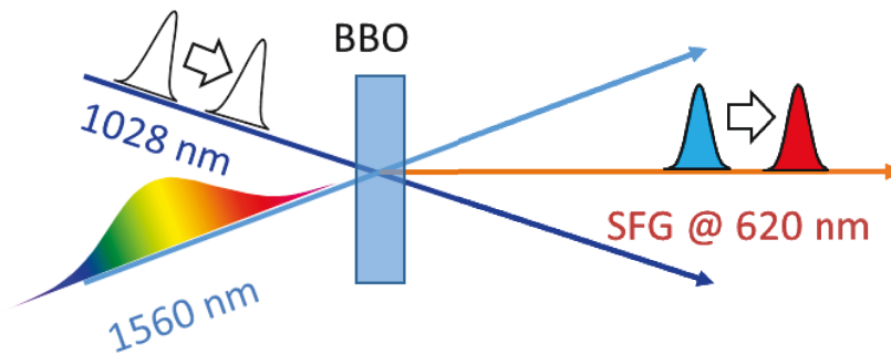
Fig. 37 : Schéma de principe pour la mesure de la gigue temporelle totale.
