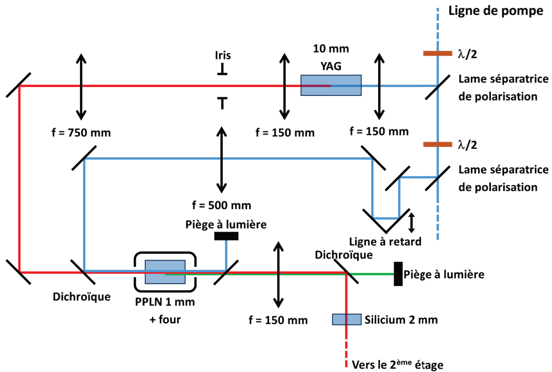
Fig. 61 : Récapitulatif de l'implémentation du 1 er étage.
