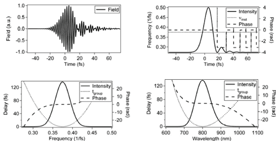
Fig. 15 : Illustration de l'effet d'une dispersion d'ordre 3 sur une impulsion. D'après (Trebino, 2012).
