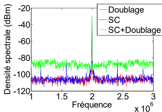
Fig. 76 : Signaux observés sur l'analyseur de spectre.
