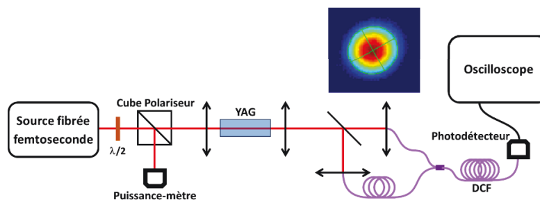
Fig. 45 : Montage expérimental. DCF : fibre à compensation de dispersion. Inset : Profil spatial (champ lointain) du supercontinuum enregistré avec une camera InGaAs après un filtre passe-haut à 1400 \text{ nm} .
