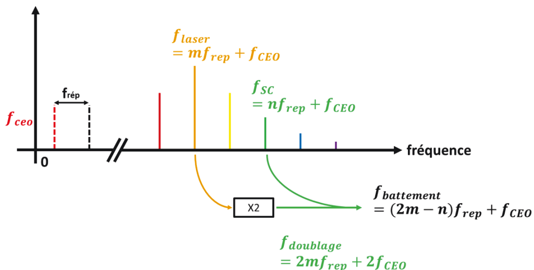
Fig. 74 : Schéma explicatif de la méthode f-2f. La fréquence de battement est un multiple de la fréquence de répétition du laser à la fréquence CEO près. Un choix judicieux de la fréquence SC permet d'observer ce battement dans le domaine RF en réalisant la condition (2m-n) proche de 0.
