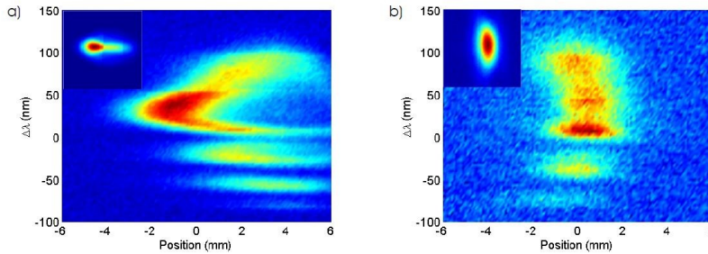
Fig. 12 : Résultat de la compensation du chirp spatial dû à l'utilisation d'un étage d'OPA non colinéaire dans (Pelletier, Sell, Leitenstorfer, & Dwayne Miller, 2012). On voit le faisceau chirpé en a), puis une fois la compensation réalisée en b). En inclusion les profils spatiaux des faisceaux.
