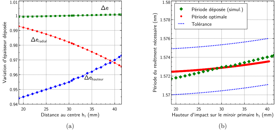
FIGURE 4.28 – Simulation de l'uniformité des couches déposées sur le miroir primaire : (a) Non-uniformité naturelle \Delta e_{\text{radial}} et due à la flèche du substrat \Delta e_{\text{hauteur}} pour le miroir primaire ; (b) Période déposée (simulation), période optimale et les tolérances en fonction de la distance au centre du miroir primaire sur sa zone utile. La simulation de la période déposée correspond au calcul de la période suivant l'équation (4.32) avec d_{1,\text{visée}}=1,5729 nm.
