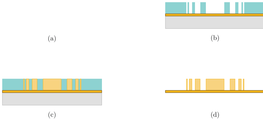
FIGURE 1.12 – Représentation très schématisée des différentes étapes de fabrication d'une lentille à zones de Fresnel (vue transverse). Les zones bleu grisé représentent les portions de polymère éclairées par le faisceau d'électrons. En bleu clair : le polymère non éclairé ; en jaune : le matériau pour les zones absorbantes de la lentille à zones de Fresnel.
