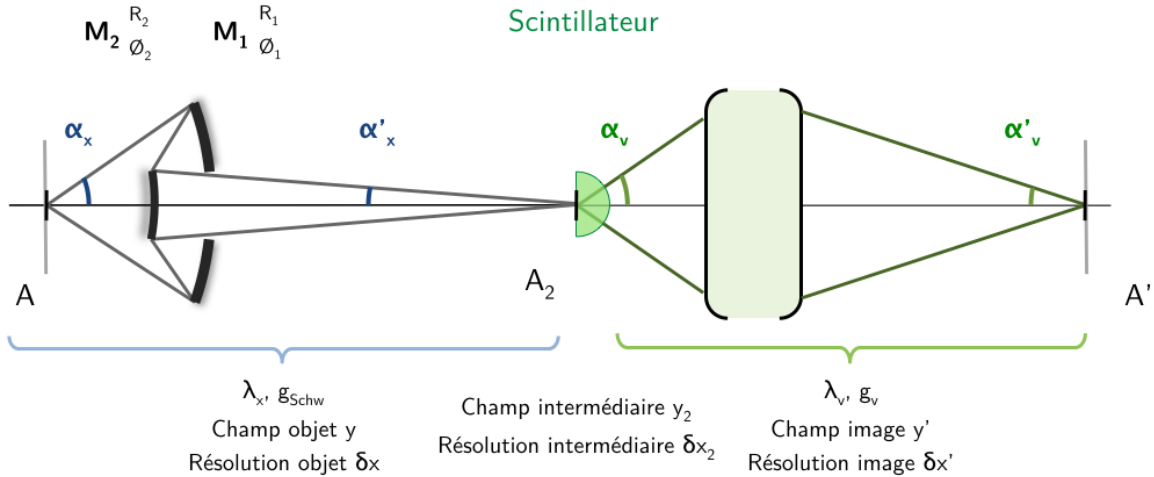
FIGURE 2.11 – Schéma du système avec conversion des rayons X en lumière visible.
