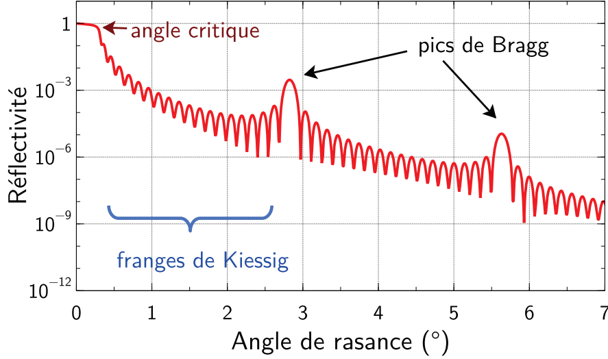
FIGURE 1.17 – Simulation de la réflectivité en fonction de l'angle d'incidence pour une multicouche [Cr/Sc] 20 à une énergie de 8,05 keV.
