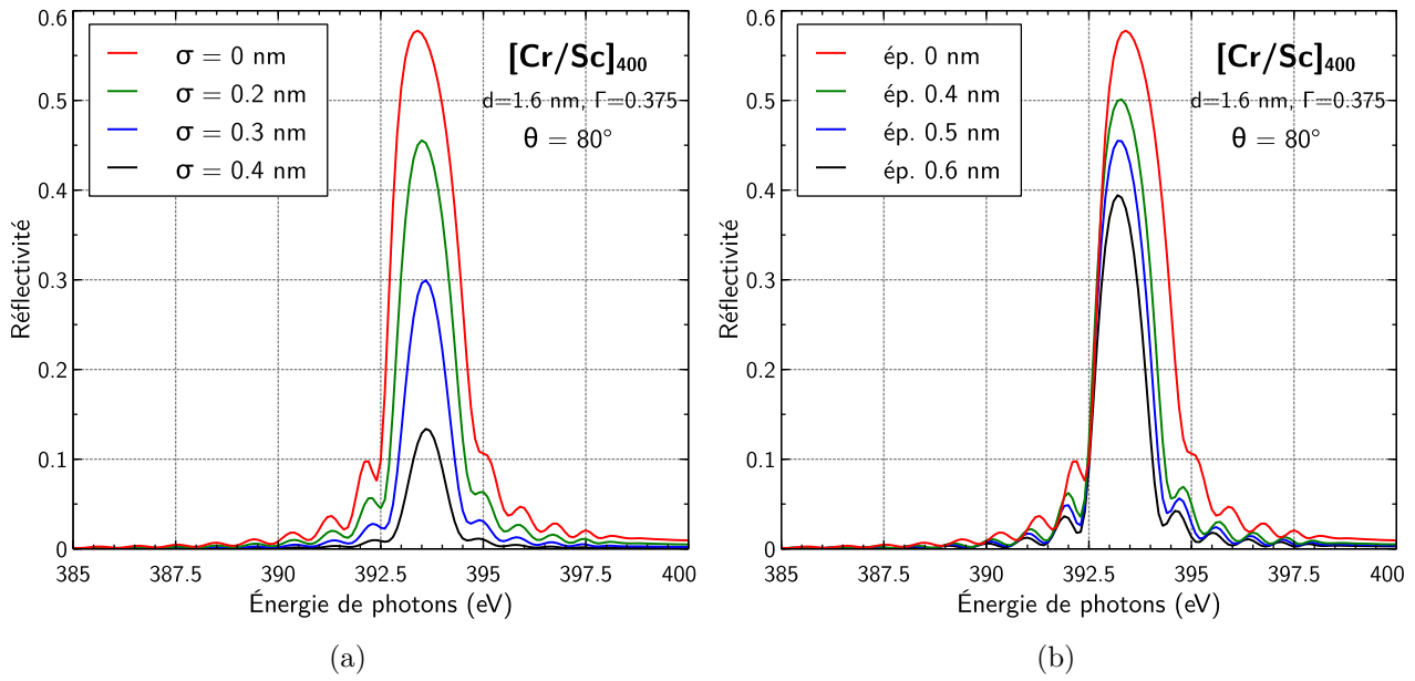
FIGURE 1.20 – Simulation de la réflectivité d’une multicouche [\text{Cr/Sc}]_{400} avec (a) différentes valeurs de la rugosité \sigma (b) simulation de l’interdiffusion pour différentes valeurs de l’épaisseur de l’interface.
