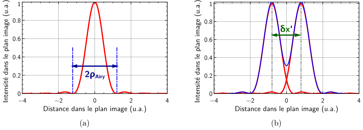
FIGURE 1.2 – Fonctions d’Airy pour (a) un point unique (b) deux points proches (en rouge : la fonction d’Airy pour les deux points séparément ; en bleu : l’intensité totale due aux deux points)
