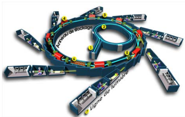
FIGURE 3.6 – Schéma de principe d'un synchrotron.
