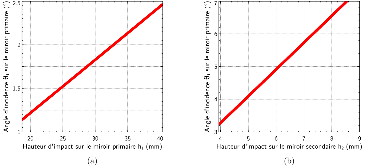
FIGURE 4.21 – Angles d'incidence sur les miroirs primaire et secondaire en fonction de la hauteur d'impact sur le miroir dans la zone utile.
