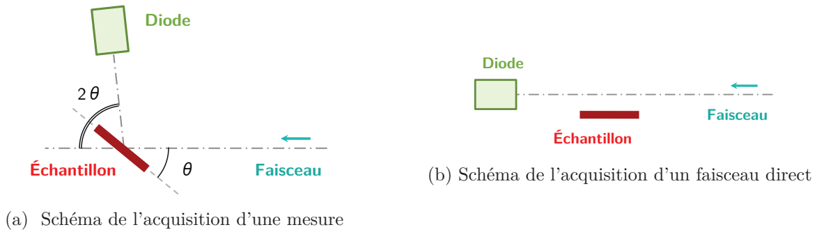
FIGURE 3.9 – Principe des mesures sur ligne de lumière synchrotron
