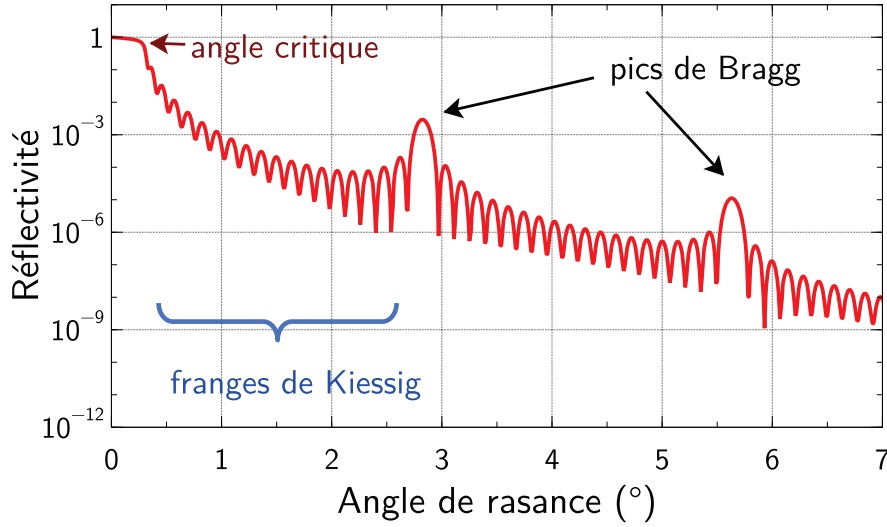
FIGURE 1.17 – Simulation de la réflectivité en fonction de l'angle d'incidence pour une multicouche [Cr/Sc] 20 à une énergie de 8,05 keV.
