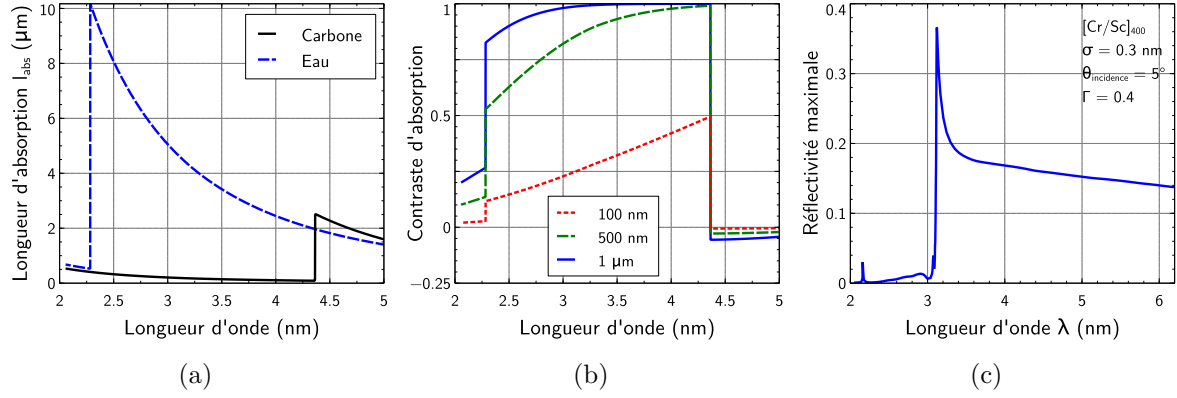
FIGURE 2.2 – Détermination de la longueur d'onde d'utilisation : (a) Longueur d'atténuation dans l'eau et le carbone en fonction de la longueur d'onde; (b) Contraste entre l'eau et le carbone pour différentes épaisseurs en fonction de la longueur d'onde (voir aussi la Figure 1.9 du Chapitre 1); (c) Réflectivité maximale de multicouches Cr/Sc en fonction de la longueur d'onde d'optimisation.
