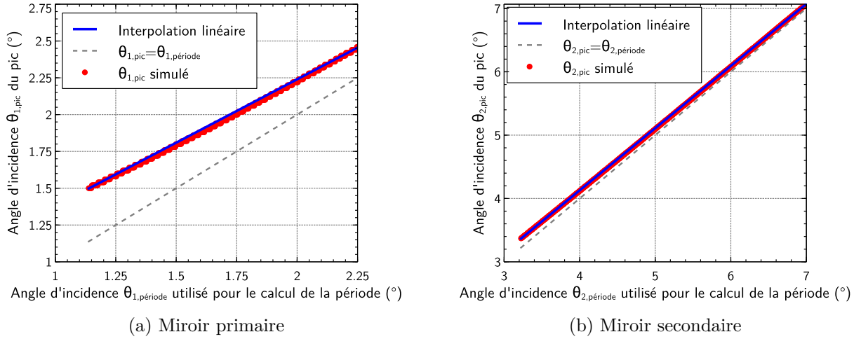
FIGURE 4.22 – Position du pic de réflectivité en fonction de celle donnée par la loi de Bragg corrigée.
