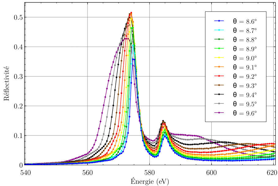
FIGURE 3.20 – Réflectivité en fonction de l'énergie pour l'échantillon MP14031 à un angle de rasance variant de 8,6° à 9,6°, mesurée sur la ligne 6.3.2 à l'ALS.
