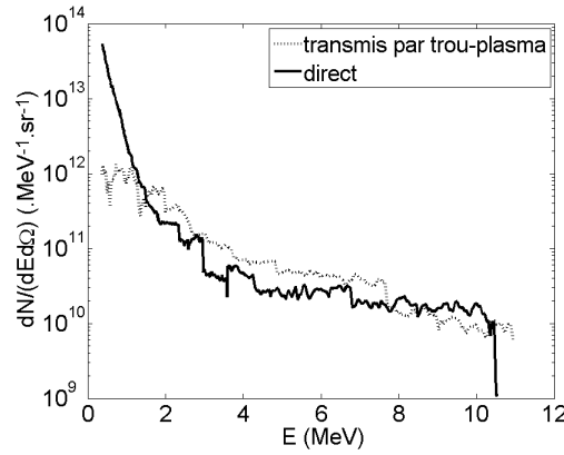
FIGURE 4.19 – Mesures de spectres de protons accélérés par TNSA sur une feuille d'or 10\ \mu m , transmis directement ou transmis par un trou effectué sur la cible de bore, placée au TCC et chauffée par le faisceau chirpé (tirs 1510098 1510099).
