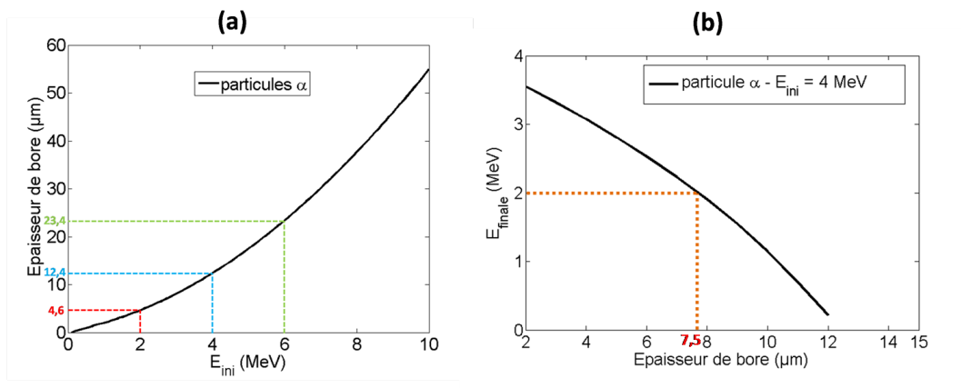
FIGURE 5.35 – (a) Épaisseur de bore que peuvent traverser des particules \alpha jusqu'à atteindre 0,1 MeV en fonction de leur énergie initiale. (b) Énergies finales de particules \alpha d'énergies initiales égales à 4 MeV en fonction de l'épaisseur de bore traversée [128].
