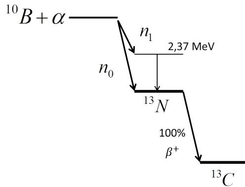
FIGURE 2.20 – Chaîne de réactions suivant la réaction ^{10}\text{B}(\alpha, n)^{13}\text{N} , ^{13}\text{N}^* .
