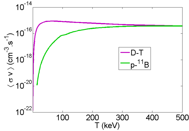
FIGURE 1.2 – Taux de réaction moyens des réactions de fusion T(D,n)\alpha et ^{11}\text{B}(p,\alpha)2\alpha en fonction de la température électronique T_e = T du plasma considéré à l'équilibre thermique [13].
