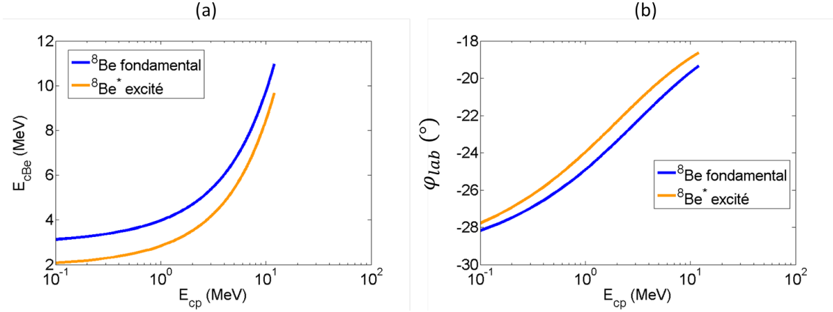
FIGURE 2.12 – (a) Energie cinétique E_{cBe} du noyau {}^8Be produit par la réaction {}^{11}B(p, \alpha){}^8Be , en fonction de l'énergie cinétique du proton E_{cp} . L'angle d'émission de la particule \alpha est fixé à \theta_{lab} = 150^\circ . (b) Angle d'émission \varphi_{lab} du noyau de {}^8Be en fonction de l'énergie cinétique du proton E_{cp} .
