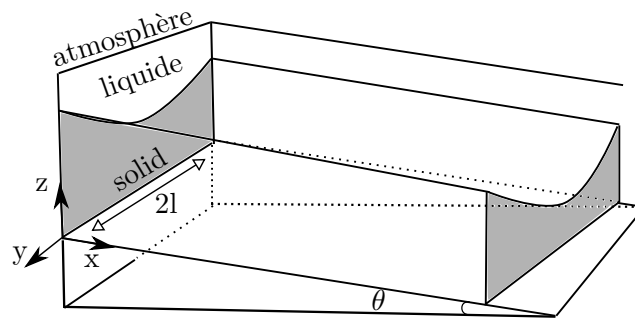
FIGURE 1 – L'écoulement quasi-statique sur un plan incliné
