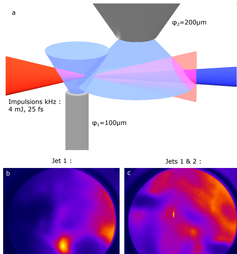
FIGURE 4.17 – a) Installation du second jet de gaz de diamètre \phi_2 = 200\mu\text{m} après le premier capillaire de diamètre \phi_1 = 100\mu\text{m} . b) Distribution électronique transverse mesurée avec le premier jet de gaz (Azote) uniquement. c) Distribution électronique transverse mesurée avec les 2 jets de gaz (Azote).
