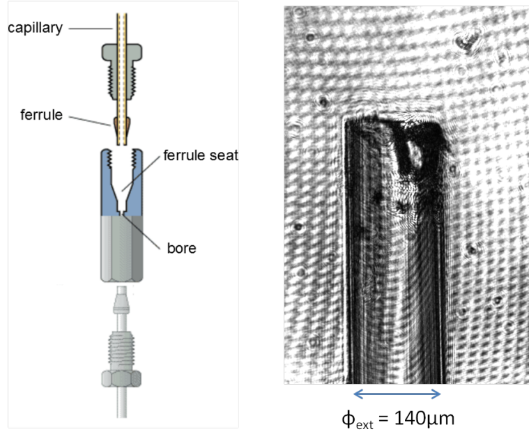
FIGURE 4.4 – Gauche : Schéma du système de fixation du capillaire permettant une utilisation en continu, et image d'un capillaire de diamètre intérieur 100 \mu\text{m} et de diamètre extérieur 140 \mu\text{m} monté dans la chambre d'interaction (droite).
