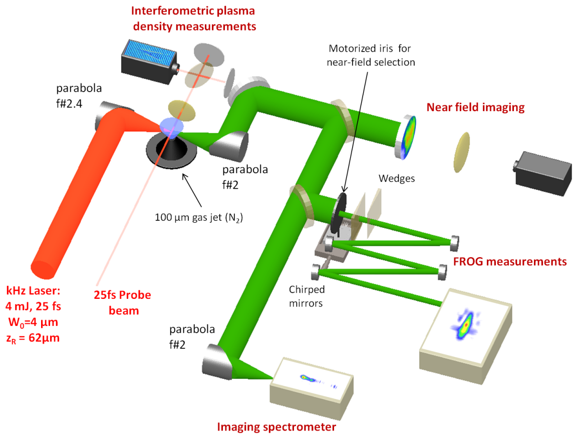
FIGURE 6.3 – Montage expérimental pour l'expérience de compression temporelle induite par ionisation.
