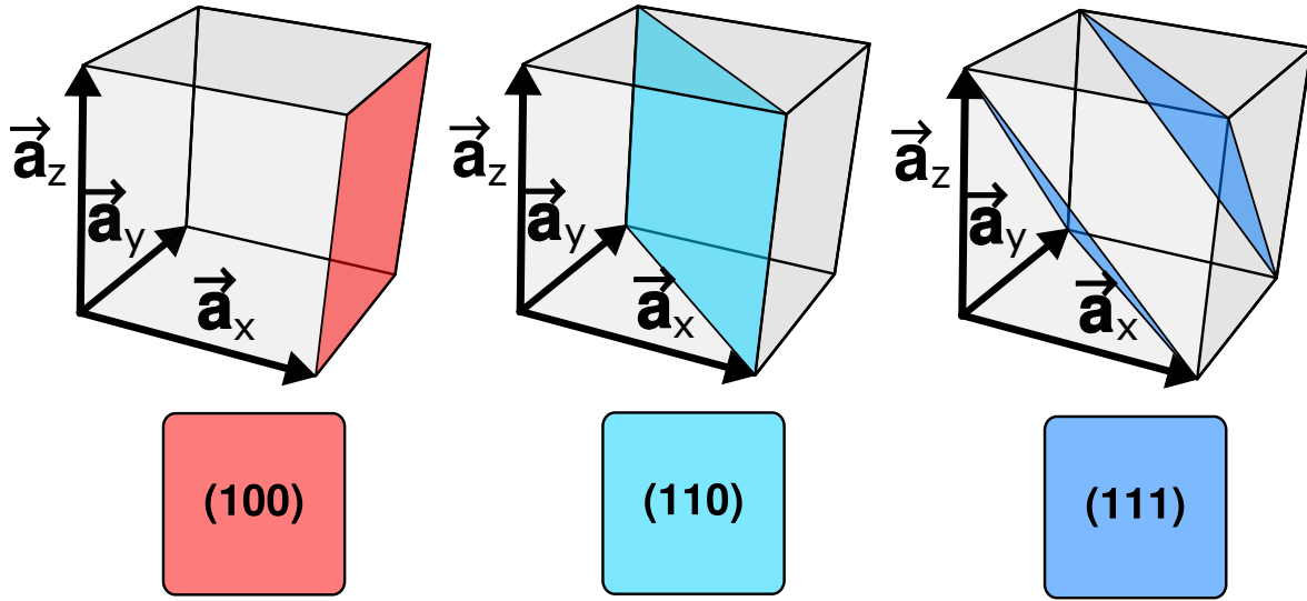
FIGURE 2.6 – Exemples de mailles et de plans définis par les indice de Miller. (image adaptée de Wikipedia)
