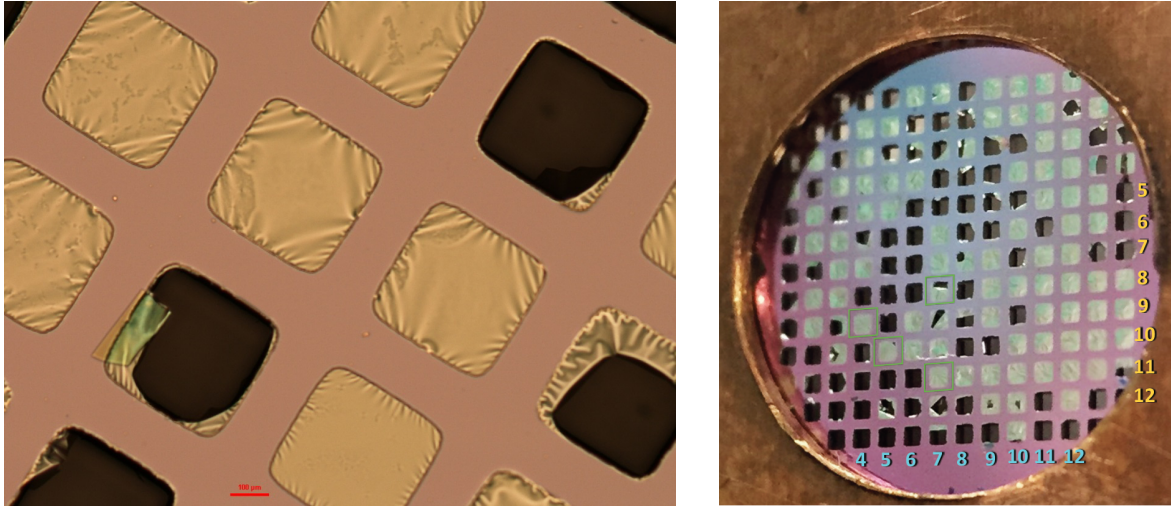
FIGURE 5.10 – A gauche : image au TEM de l'échantillon, montrant une grille de pas 350 \mu\text{m} sur laquelle sont synthétisées des couches de 30 nm de Si. A droite : Photo de l'échantillon dans sa monture, dans l'enceinte expérimentale.
