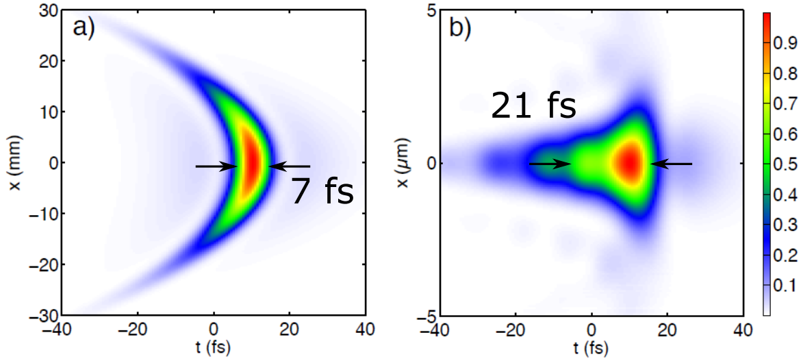
FIGURE 6.2 – Représentation de l'effet du couplage spatio-temporel \phi(x, y, \omega) = \alpha(x^2 + y^2)(\omega - \omega_0) . a) Intensité I(x, t) d'une impulsion dont le spectre en intensité correspond au type de spectre mesuré expérimentalement après élargissement spectral, et dont la phase spectrale représente ce couplage appelé "pulse front curvature". b) Résultat de la propagation de l'impulsion jusque dans le champ lointain : la durée de l'impulsion augmente de 7 fs FWHM dans le champ proche à 21 fs FWHM au foyer.
