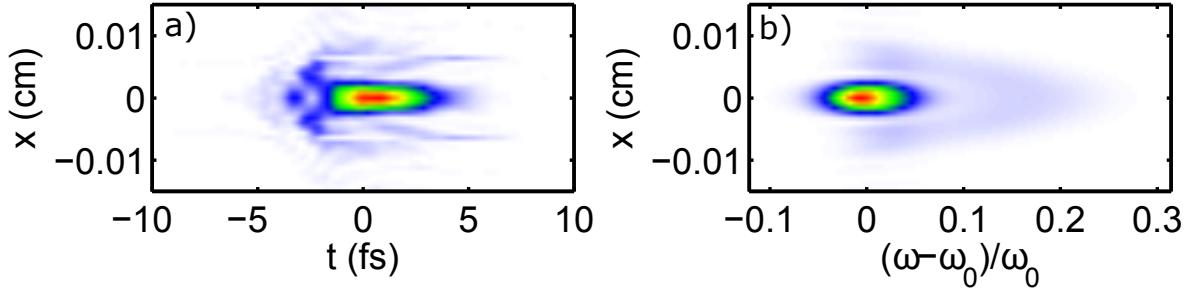
FIGURE 6.15 – Enveloppes temporelle (a) et spectrale (b) de l'impulsion obtenues après propagation jusqu'en champ proche du spectre et de la phase provenant du modèle pour l'ionisation.
