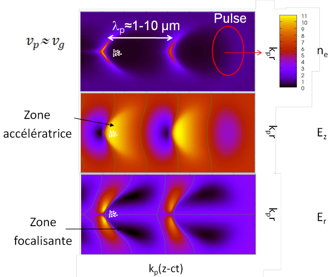
FIGURE 3.3 – Représentation des champs longitudinaux et transverse associés à la génération d'une onde plasma non linéaire. En haut : carte de la densité électronique. L'impulsion laser est représentée en rouge, et la flèche indique la direction de propagation. La vitesse de phase de l'onde plasma excitée est proche de la vitesse de groupe de l'impulsion laser. Au milieu : Champ électrique longitudinal. En bas : champ électrique transverse. La longueur d'onde plasma \lambda_p \approx 1 - 10\ \mu\text{m} donne une idée de la longueur d'onde typique dans les expériences d'accélération d'électrons. La partie arrière de la cavité ionique est propice pour l'accélération d'électrons car les champs y sont à la fois accélérateur et focalisant.
