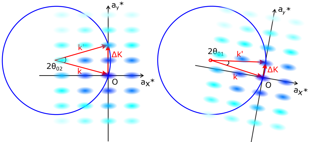
FIGURE 2.8 – Représentation de la sphère d'Ewald pour 2 angles de Bragg différents. En pratique, il est plus commode de tourner le cristal plutôt que de changer l'angle du faisceau incident. À gauche, l'angle optimise la diffraction sur le pic d'indice (h,k) = (0,2) , et à droite sur le pic (h,k) = (0,1) .
