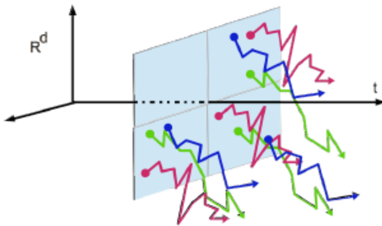
FIGURE 2.4: Description sur comment utiliser les root samples pour construire de nouvelles trajectoires
