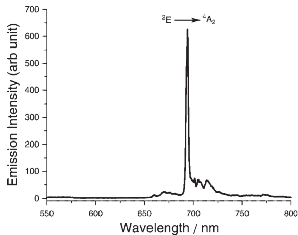
Figure A5 - 7 : Spectre d'émission du rubis (Esposti & Bizzocchi 2007).
