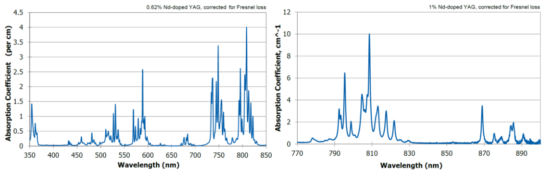
Figure A5 - 3 : Spectre d'absorption du Nd:YAG (source : Northrop Grumman).
