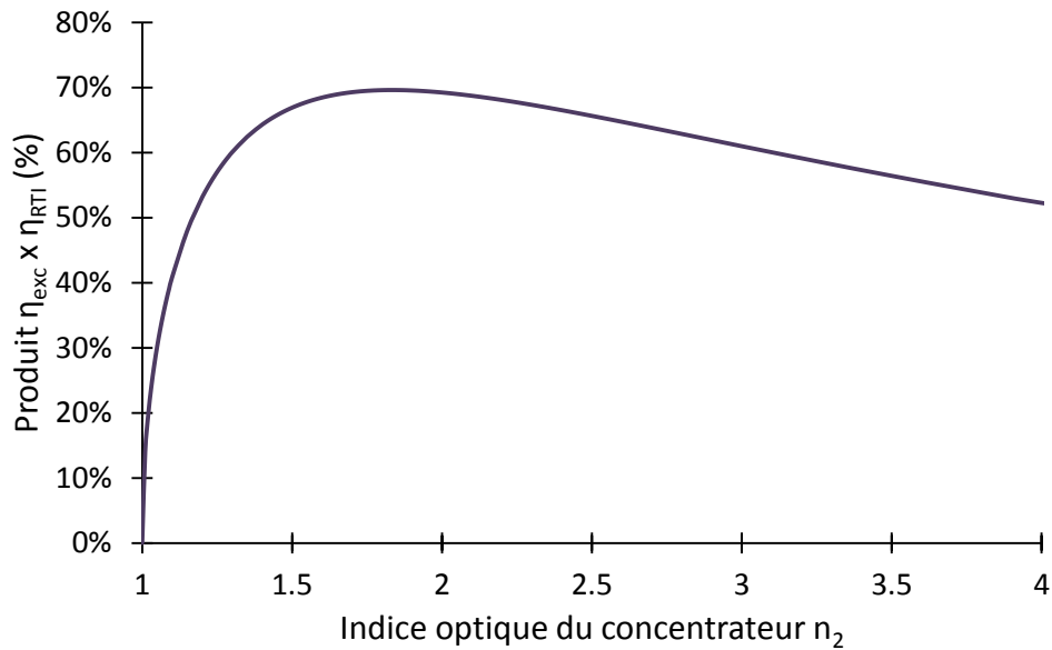
Figure III-12 : Évolution du produit \eta_{exc} \times \eta_{RTI} en fonction de l'indice du concentrateur ( \eta_Q = 1, n_1 = 1 ).
