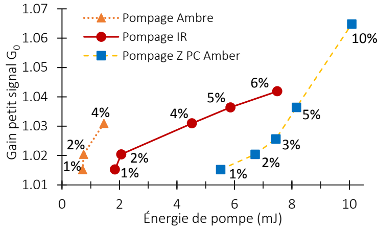
Figure II-35 : Gain petit signal G_0 en fonction de l'énergie de pompe nécessaire pour atteindre le seuil laser, pour différentes transmissions de coupleur, pour chacun des pompages.
