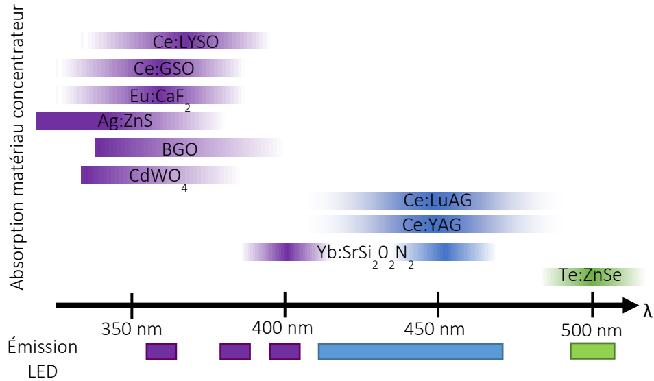
Figure III-16 : Comparaison des bandes d'absorption des matériaux concentrateur (en haut) et d'émission des LEDs (en bas).
