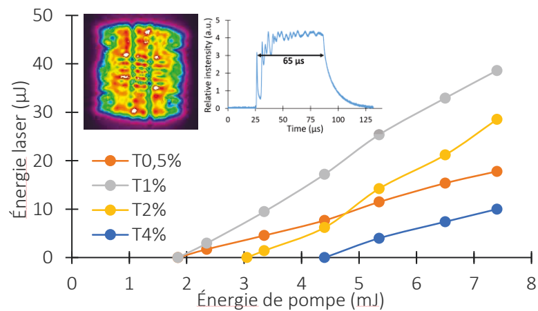
Figure II-31 : Énergie laser en fonction de l'énergie de pompe émise par les deux panneaux de LEDs IR. Durée de pompe : 100 \mu s, fréquence : 250 Hz, rayon de courbure du miroir HR : 500 mm. Insert : photos des profils spatial et temporel du laser.
