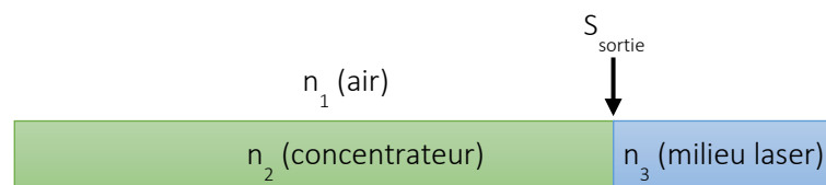
Figure III-10 : Différences d'indices optiques à prendre en compte pour extraire le plus de lumière possible : \Delta n_{21} = n_2 - n_1 et \Delta n_{32} = n_3 - n_2 .
