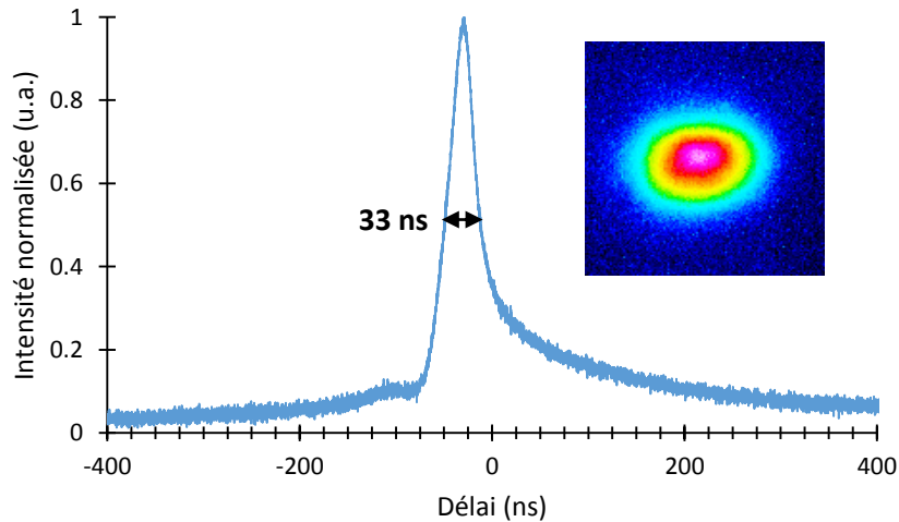
Figure IV-27 : Profils temporel et spatial de l'impulsion laser monomode transverse, ayant une énergie de 263 \mu\text{J} . Pompage avec les concentrateurs de 2,5 et 14 mm pendant 250 \mu\text{s} à 10 Hz, absorbant saturable T_0 = 80\% , coupleur de sortie T = 10\% , R = 500 \text{ mm} , L_{cav} = 80 \text{ mm} .
