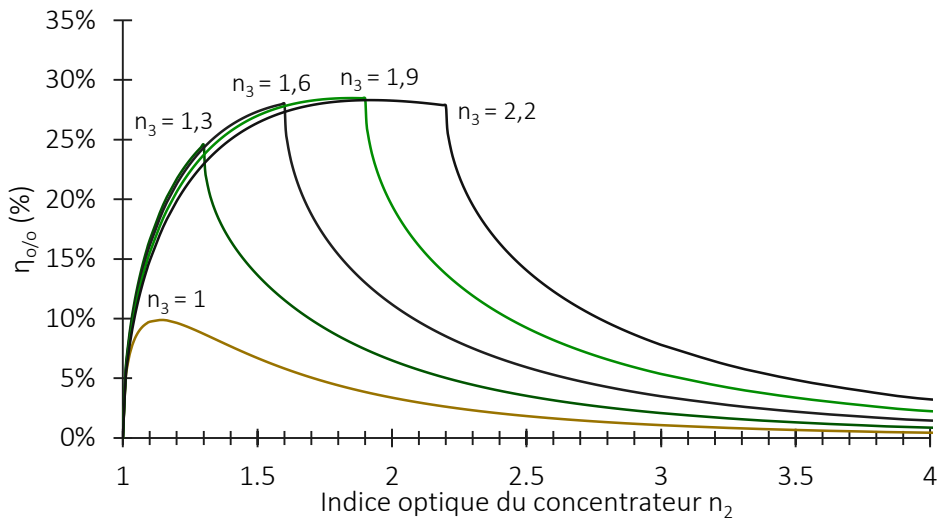
Figure III-13 : Efficacité optique \eta_{o/o} du concentrateur en fonction de son indice, pour différents indices optiques du milieu laser, en supposant un concentrateur sans perte avec \eta_0 = 1 .
