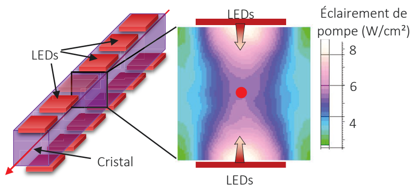
Figure II-11 : Carte d'éclairement de pompe au sein du cristal – coupe transversale.
