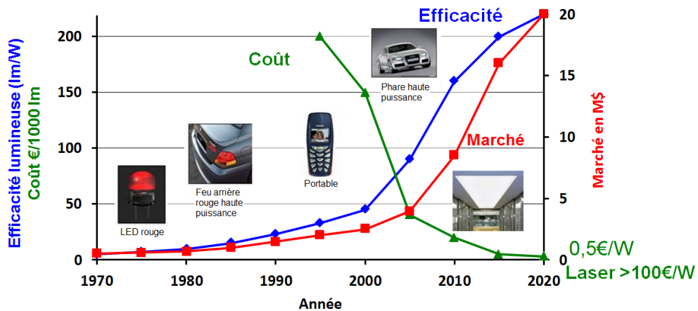
Figure I-2 : Évolution de l'efficacité et du coût des LEDs au fil des années.
