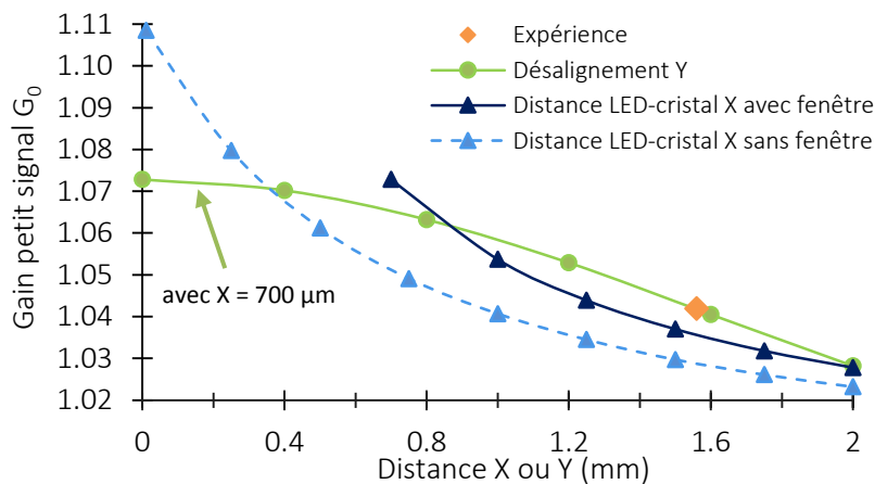
Figure II-38 : Évolution du gain petit signal théorique G_0 en fonction du désalignement entre les deux panneaux de LEDs IR ( Y ) et la distance entre les LEDs et le cristal ( X ).
