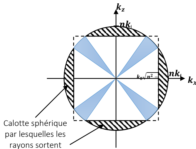
Figure A2- 6 : Coupe à 2D des rayons sortant et piégés.
