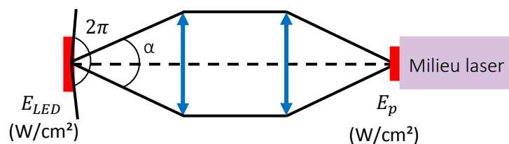
Figure II-5 : Focalisation de l'éclairement émis par une LED à l'aide d'un jeu de lentilles. E_{LED} = éclairement de la LED, E_p = éclairement de pompe incident sur le cristal laser, \alpha = angle d'ouverture du système optique.
