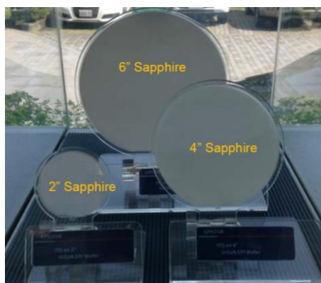
Figure I-22 : Substrats de saphir servant de base pour l'épitaxie (présentation Épistar).
