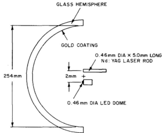
Figure I-6 : Schéma du réflecteur utilisé pour coupler la lumière en sortie de la LED dans un barreau laser.
