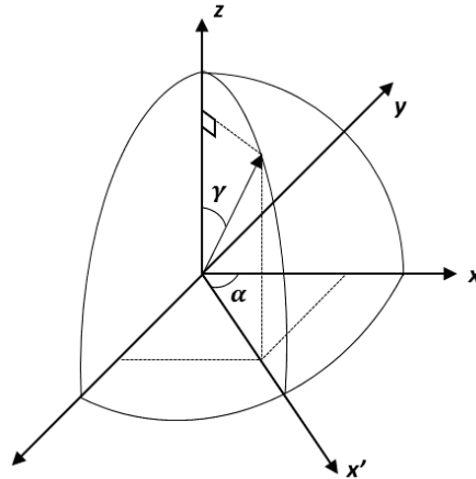
Figure A2-3 : Repère dans lequel sont définies les coordonnées sphériques.
