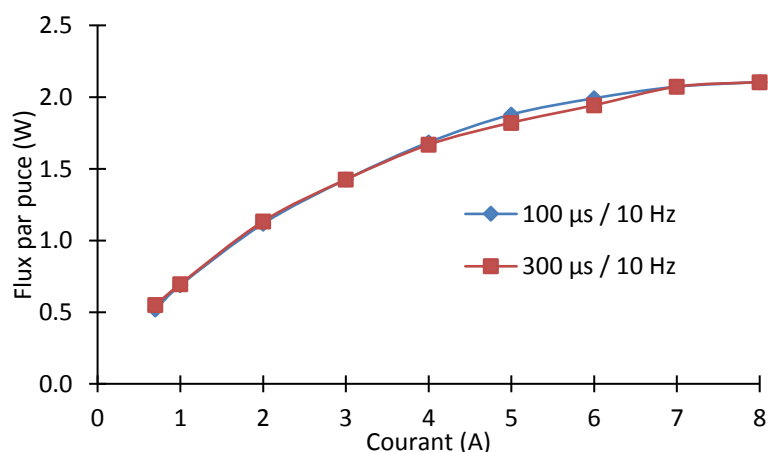
Figure II-28 : Évolution de la puissance en sortie d'une LED Z PC Amber en fonction du courant injecté, pour des impulsions de 100 \mu s et 300 \mu s, à 10 Hz.
