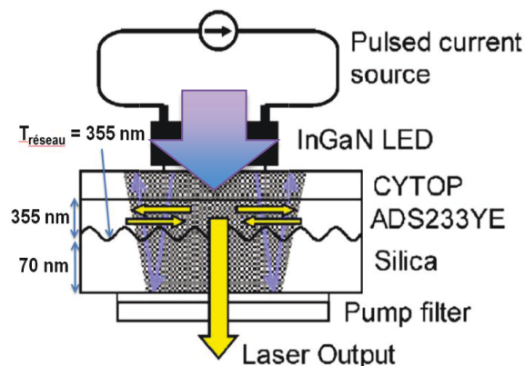
Figure I-7 : Schéma d'un laser à polymère pompé par LED (Yang et al. 2008).
