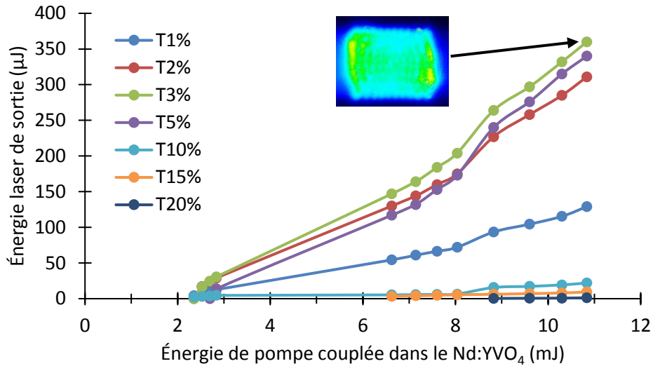
Figure IV-9 : Évolution de l'énergie en sortie du laser en fonction de l'énergie couplée dans le Nd:YVO 4 , pour différentes transmissions du coupleur de sortie. Pompage avec le concentrateur de 9 mm pendant 100 µs à 100 Hz, cavités plans-concaves, longueurs = 70 - 85 mm.
