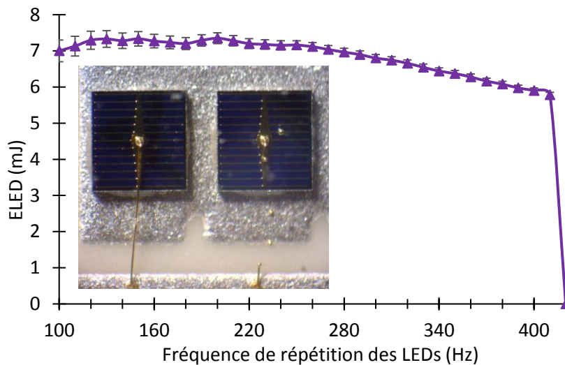
Figure II-26 : Étude en fréquence de l'énergie émise par les 2 panneaux de LEDs IR au courant maximal de 6,7 A/mm 2 . Insert : photographie des LEDs IR après la cassure.
