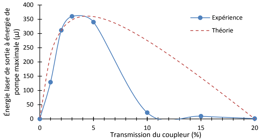
Figure IV-10 : Évolution de l'énergie de sortie à énergie de pompe maximale (10,8 mJ) en fonction de la transmission des coupleurs de sortie.
