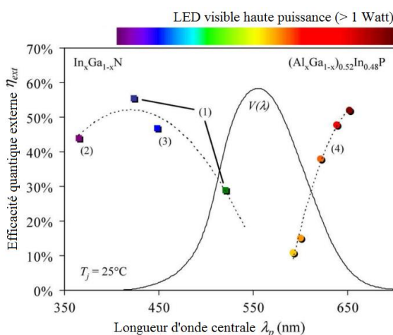
Figure I-23 : État de l'art des rendements quantiques externes de LEDs visibles hautes puissances, à 25°C. (1) LEDs TFFC 6 en InGaN, 350 mA ; (2) LED VTF en InGaN, 1000 mA ; (3) LEDs CC en InGaN avec des substrats structurés ; (4) Performances de LEDs de production en AlGaInP à 350 mA de chez Philips Lumileds Lighting Co.; V(\lambda) est la
