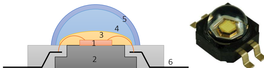
Figure I-27 : (à gauche) Schéma d'une LED « Leadform » avec une puce (1), un support d'interconnexion et de dissipation thermique (2), un luminophore (3), un encapsulant (4), une lentille (5) et des pattes d'interconnexion externes (6) ; (à droite) illustration d'une LED « Leadform », source : Lumileds.
