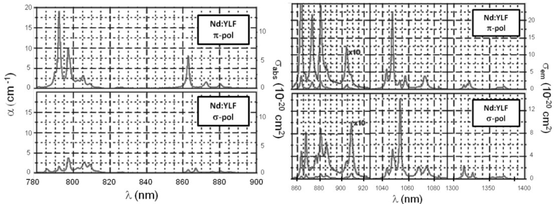
Figure A5 - 4 : Sections efficaces d'absorption et d'émission du Nd:YLF (Neto 2012).
