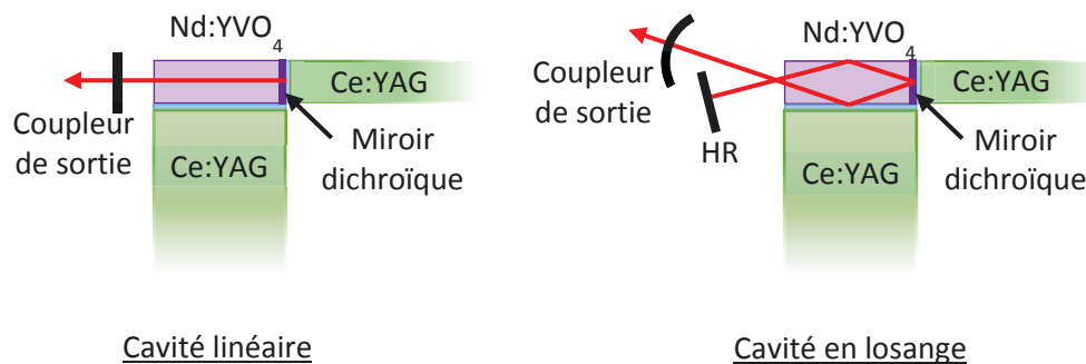
Figure IV-17 : Types de cavités laser testées.
