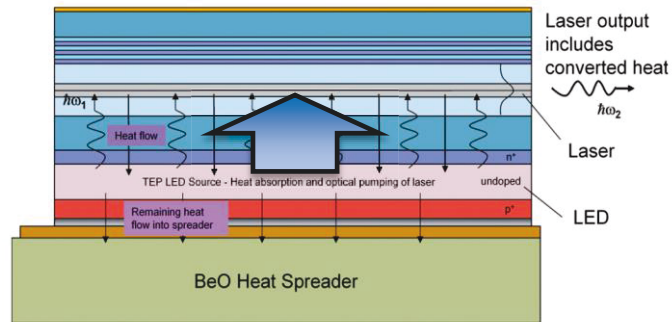
Figure I-8 : Illustration schématique de la LED (GaAs) intégrée au semi-conducteur laser (X. Liu et al. 2013).
