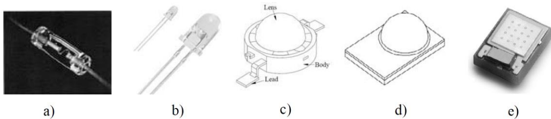
Figure I-25 : Évolution des boîtiers des LEDs : a) 1ère LED (Holonyak & Bevacqua 1962), b) LED à broches, c) LED CMS « Leadform », d) LED CMS « Leadless », e) LED CSP
