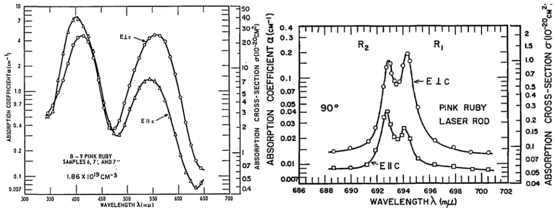
Figure A5 - 6 : Spectre d'absorption du rubis (Cronemeyer 1966).
