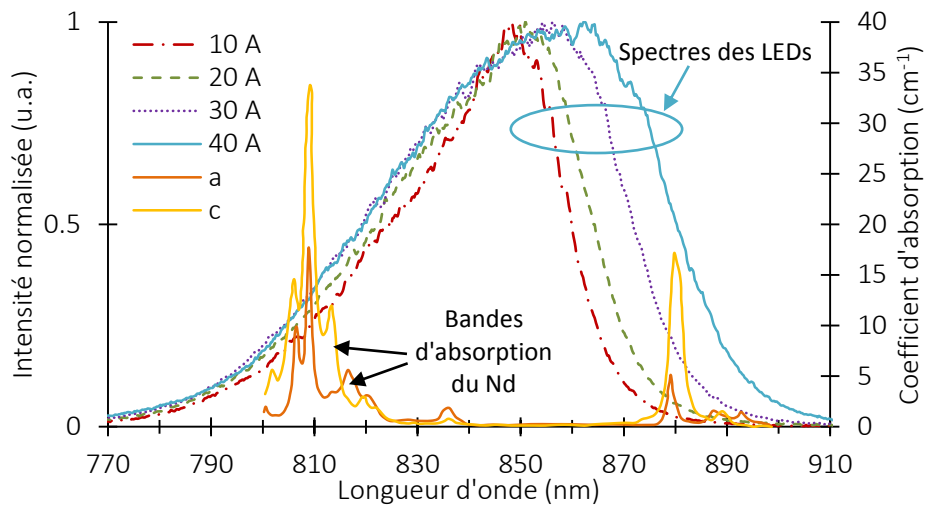
Figure II-25 : Déformation spectrale pour différents courants injectés et bandes d'absorption du Nd:YVO 4 pour un dopage de 1,0 at. % (Mcdonagh et al. 2006).
