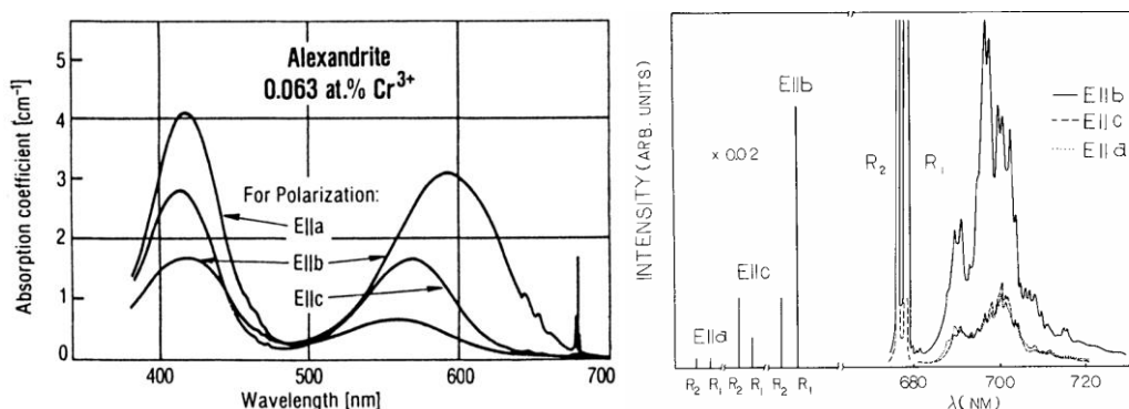
Figure A5 - 1 : (à gauche) absorption et (à droite) émission à 77 K de l'alexandrite (Bukin & Matrosov 1981; Koechner 2006).
