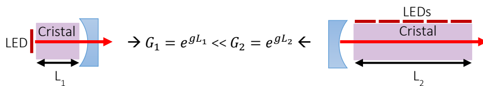
Figure II-3 : Comparaison des pompages longitudinal et transverse.
