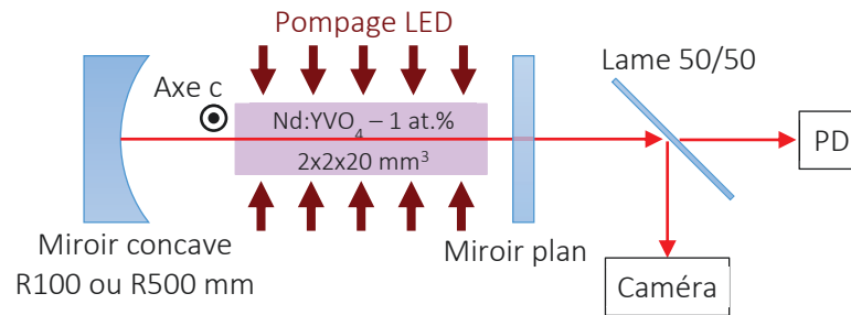
Figure II-15 : Architecture de la cavité laser. PD = photodiode.
