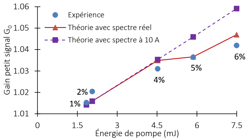
Figure II-36 : Gain petit signal G_0 théorique et expérimental en fonction de l'énergie de pompe en sortie des deux panneaux de LEDs IR nécessaire pour atteindre le seuil laser, pour différentes transmissions de coupleur.
