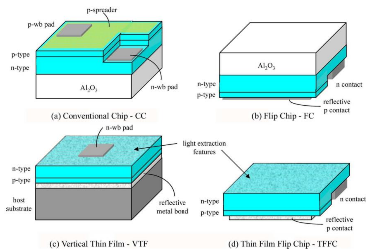
Figure I-24 : Configurations typiques de LEDs en InGaN-GaN. (a) Conventional chip (CC) avec un contact p semi-transparent, (b) Flip-chip (FC) avec un contact p réfléchissant, (c) Vertical-injection thin film (VTF) adhérent à un réflecteur en métal, (d) Thin-film flip-chip (TFFC). Les deux configurations « thin-film » permettent d'avoir accès à la surface en GaN et d'améliorer l'extraction de la lumière (en structurant la surface ou à l'aide de micro-optiques), (Krames et al. 2007).
