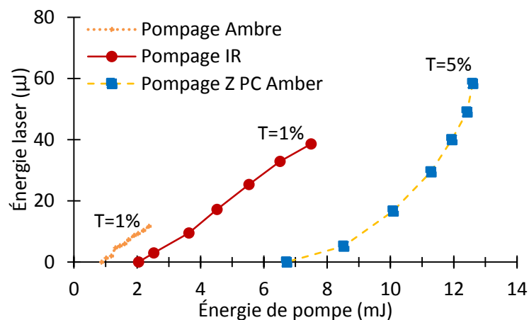
Figure II-34 : Comparaison des énergies laser en fonction de l'énergie de pompe pour un pompage dans l'ambre, dans l'IR ou avec des LEDs Z PC Amber. Durée de pompe 100 \mu s.
