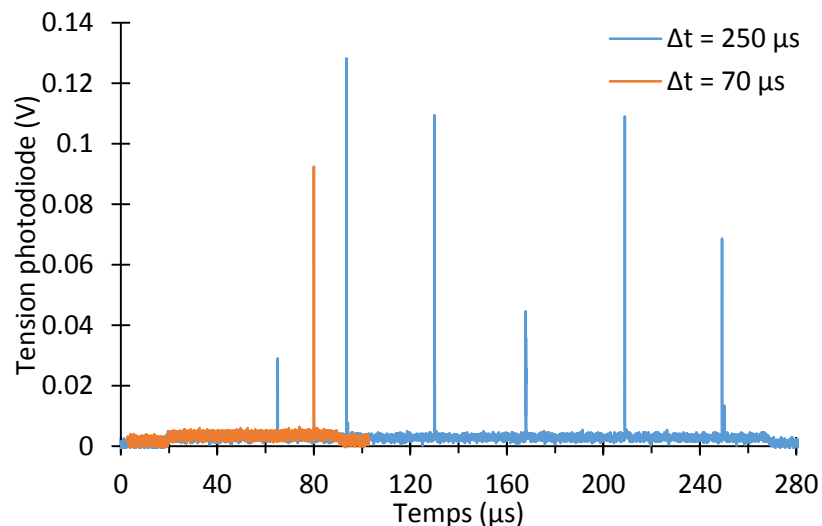
Figure IV-25 : Profil temporel typique des impulsions laser Q-switch pour des durées de pompe différentes. Mesures réalisées avec un oscilloscope Tektronix TDS3032 (bande passante = 300 MHz).
