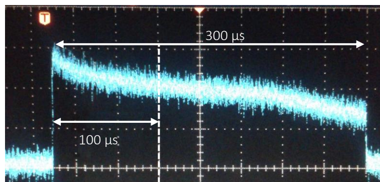
Figure II-24 : Profil temporel d'une impulsion de pompe émise par un panneau de LEDs ambre.
