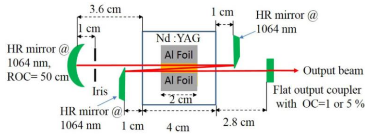
Figure I-13 : Schéma de la cavité en Z réalisée par (Huang et al. 2016).
