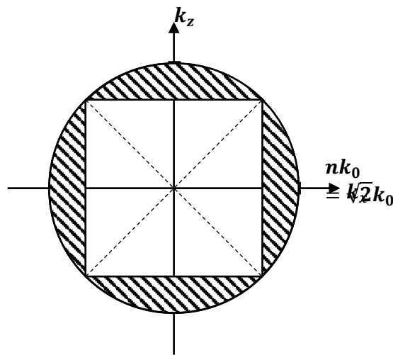
Figure A2- 8 : En 2D, la condition limite pour qu'il y ait des rayons piégés est n > \sqrt{2} .
