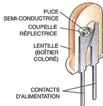
Figure I-26 : Schéma d'une LED à broches (Craford et al. 2001).
