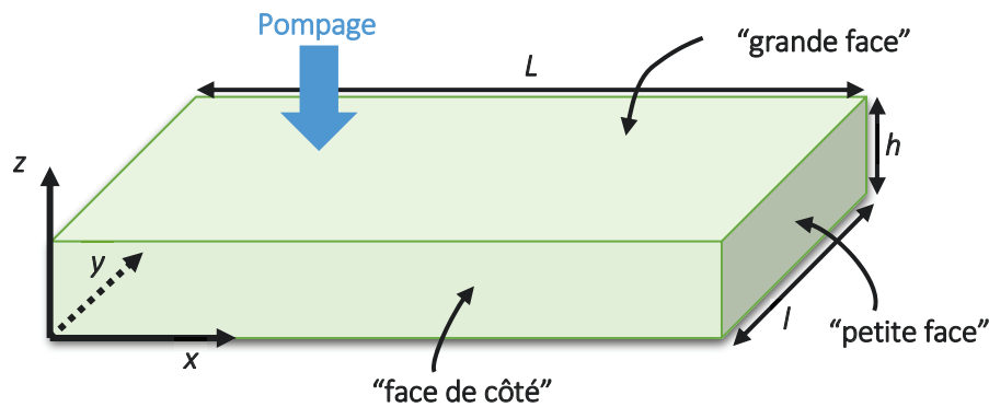
Figure A2- 1 : Géométrie du concentrateur considéré.
