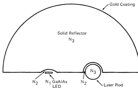
Figure I-5 : Schéma de pompage utilisé par (Farmer & Kiang 1974) utilisant un réflecteur d'indice N_3 .
