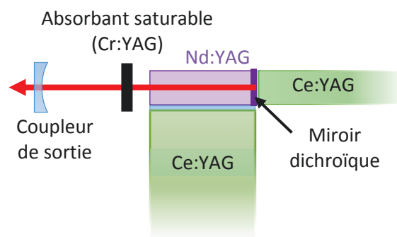
Figure IV-21 : Schéma de la cavité laser en déclenchement passif à l'aide d'absorbants saturables.
