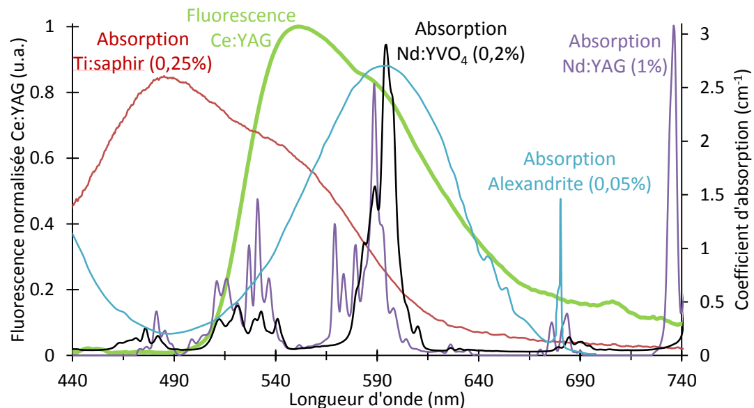
Figure IV-11 : Spectres d'émission du Ce:YAG et d'absorption du Ti:saphir (moyenne des axes a et c), du Nd:YAG, du Nd:YVO 4 (axe c) et de l'alexandrite (parallèle à l'axe b) 20 , avec les dopages associés.
