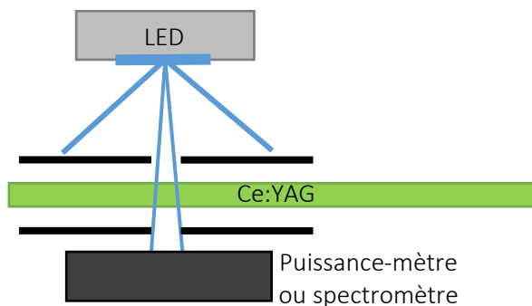
Figure III-19 : Schéma expérimental pour mesurer l'absorption du Ce:YAG après 1 mm de propagation.
