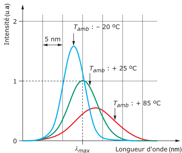
Figure I-15 : Évolution du spectre d'émission d'une LED avec la température (Zissis & Logivière 2011).
