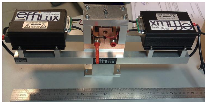
Figure II-18 : Photo du dispositif de pompage réalisé et assemblé avec les alimentations des LEDs de chaque côté.
