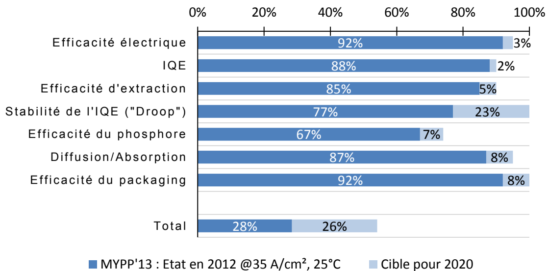
Figure I-30 : Les différentes efficacités d'une LED, MYPP = Multi-Year Program Plan, IQE = Internal Quantum Efficiency, EQE = External Quantum Efficiency, stabilité de l'EQE : EQE à 100 A/cm 2 relative à 35 A/cm 2 .
