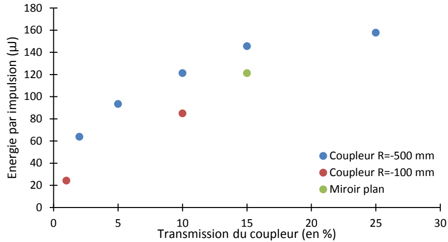
Figure IV-26 : Énergie laser pour une émission monomode transverse pour différents coupleurs de sortie, en régime déclenché. Pompage avec les concentrateurs de 2,5 et 14 mm pendant 80 \mu\text{s} à 10 Hz, absorbant saturable T_0 = 85\% , L_{cav} = 80 \text{ mm} .
