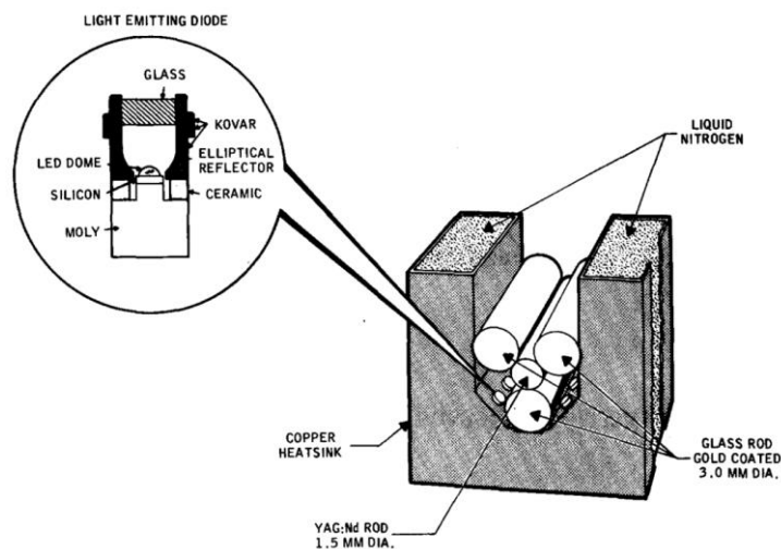
Figure I-3 : Schéma du laser Nd:YAG pompé par LED de (Allen & Scalise 1969).
