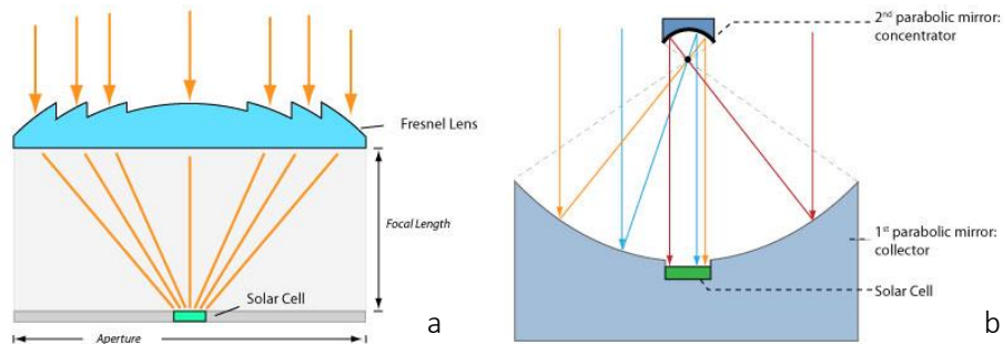
Figure III-1: (a) lentille de Fresnel illuminant une cellule photovoltaïque, (b) concentrateur à deux miroirs paraboliques. 18
