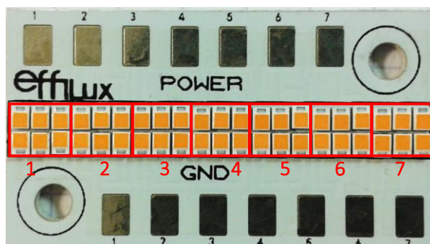
Figure II-27 : Illustration d'un panneau de LEDs Luxeon Z PC Amber avec la répartition en groupes de 6 puces.
