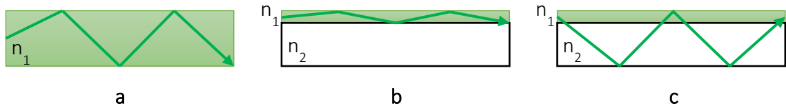
Figure III-4 : (a) concentrateur massif uniformément dopé, (b) colorant sur lame bas indice n_1 > n_2 , (c) colorant sur lame haut indice n_1 < n_2 .
