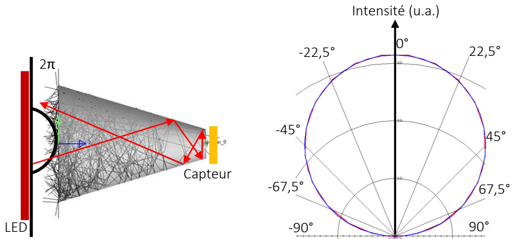
Figure II-6 : Simulation d'un cône concentrant la lumière de la LED (à gauche). Indicatrice de sortie de la petite face (à droite).
