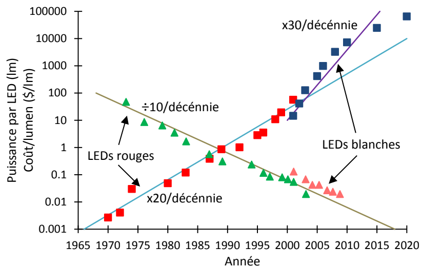
Figure I-21 : Loi de Haitz : en 10 ans, la puissance émise par une LED augmente d'un facteur 20 et son prix est divisé par 10 (Liu et al. 2009).
