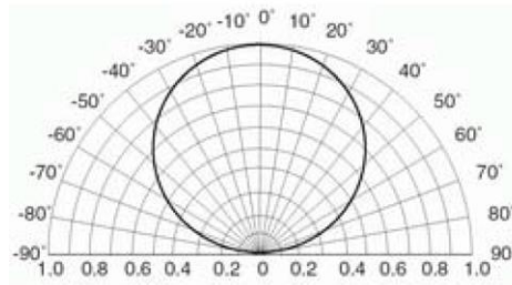
Figure II-4 : Indicatrice d'intensité (ou diagramme d'émission) d'une LED non-lentillée.
