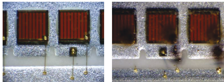
Figure II-22 : À gauche : connectique des LEDs ambre avant cassure, à droite : connectique après cassure.
