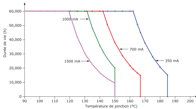
Figure I-20 : Durée de vie d'une LED K2 Luxeon (B50 L70) en fonction du courant et de la température de jonction (Zissis & Logivière 2011), issue de la documentation Luxeon.
